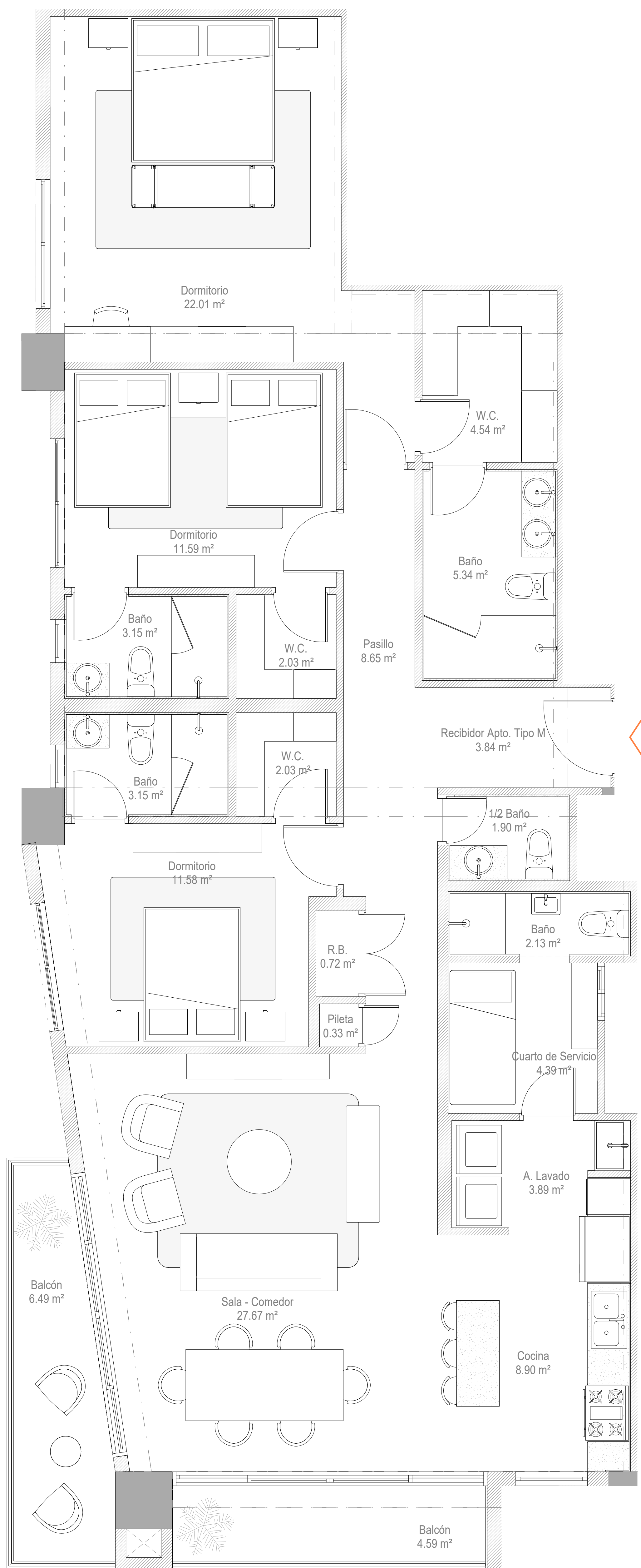
1 PLANTA ARQ. AMUEBLADA APTO. TIPO M 7/89 1:30
