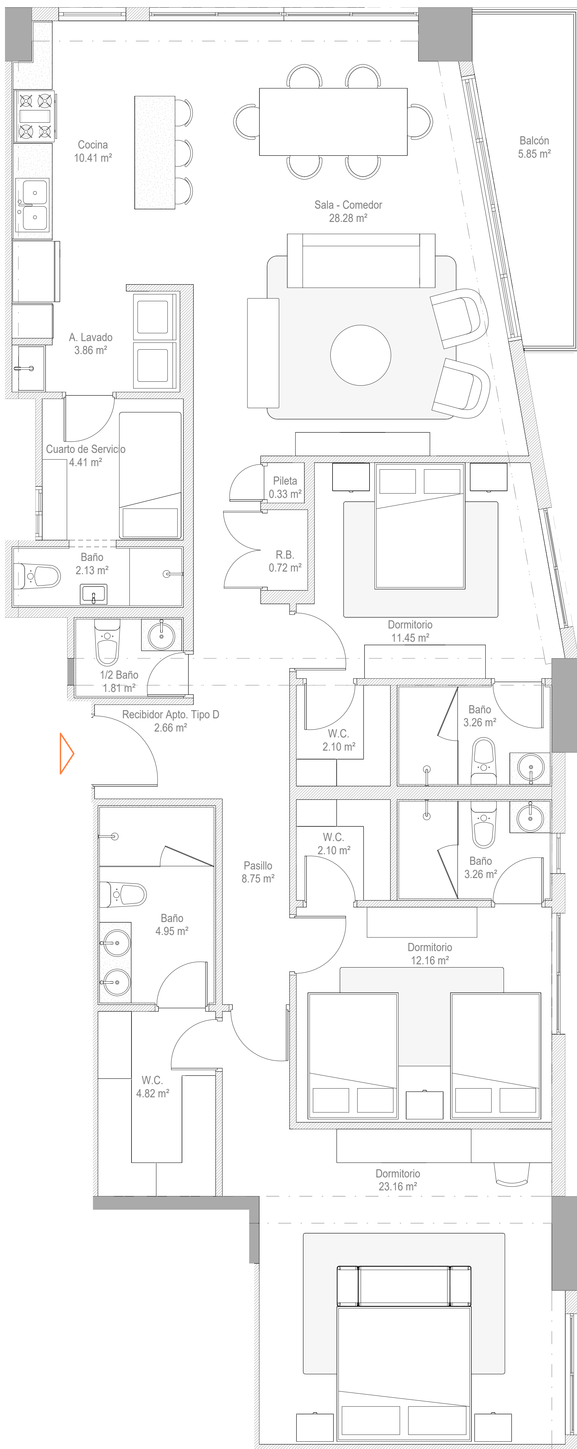
2 PLANTA ARQ. AMUEBLADA APTO. TIPO D A12 1:30
