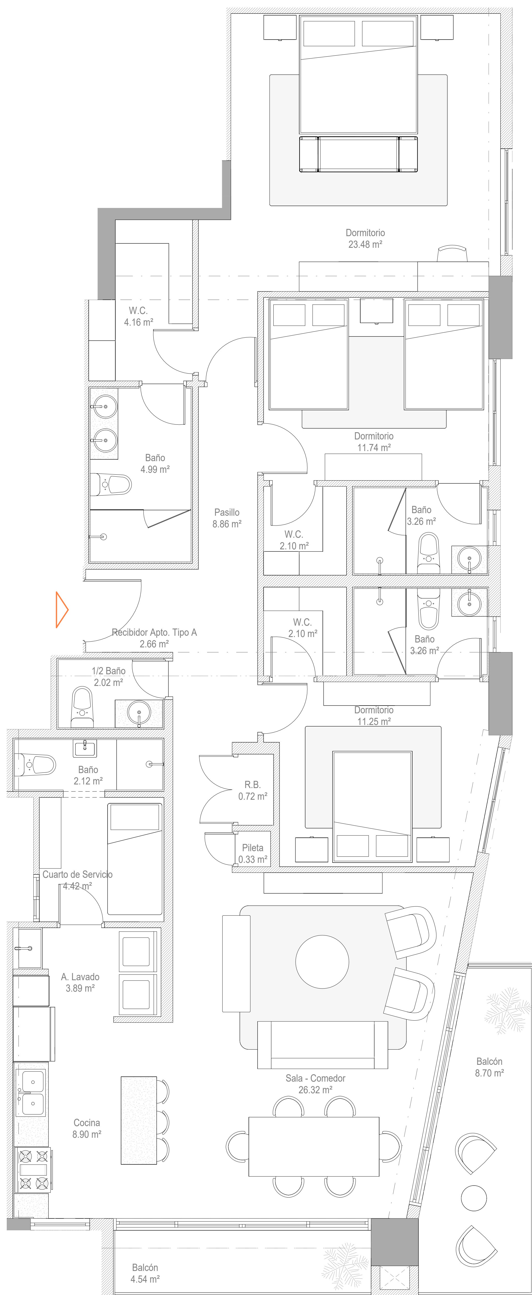
2 PLANTA ARQ. AMUEBLADA APTO. TIPO A A10/1-30
