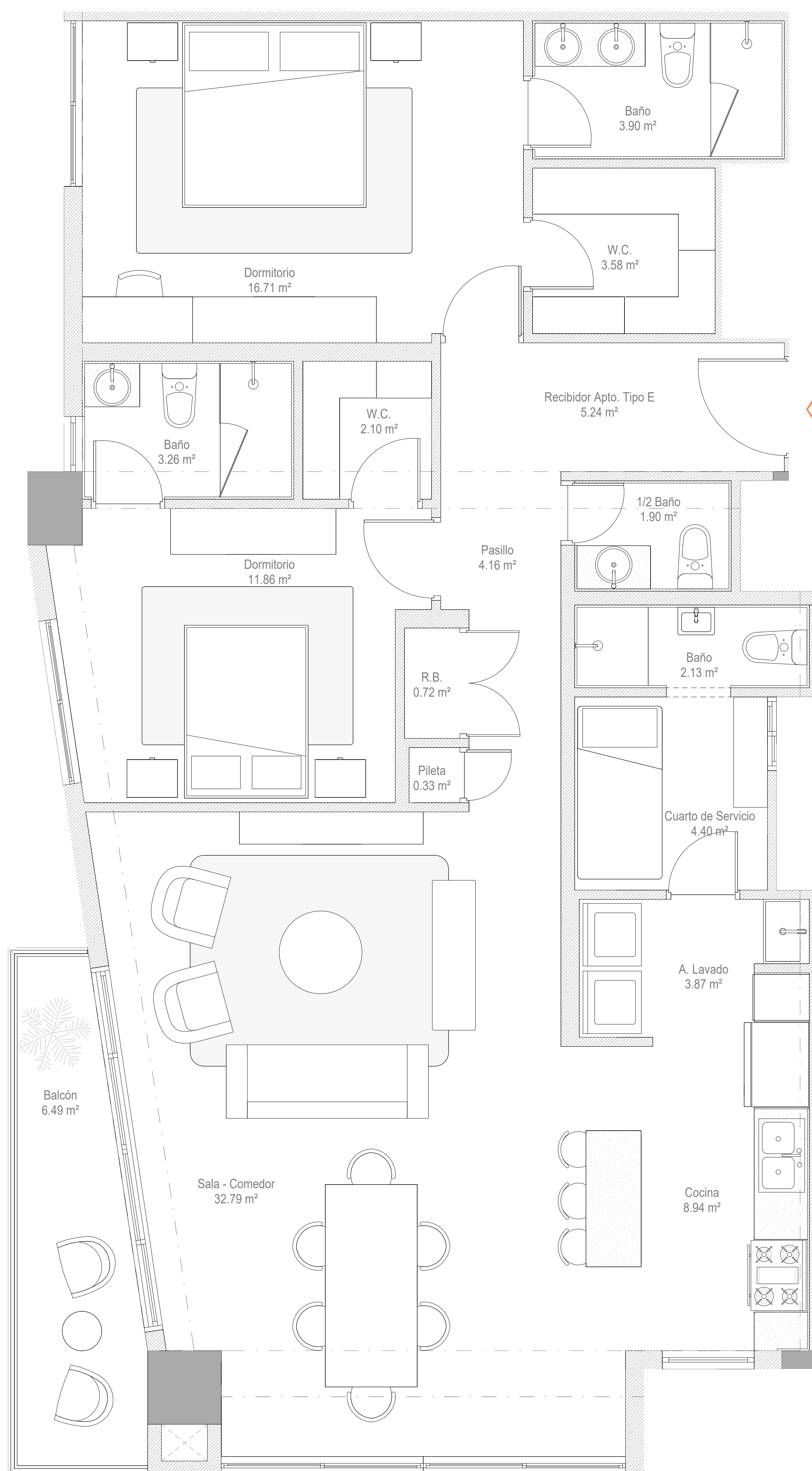
PLANTA ARQ. AMUEBLADA APTO. TIPO E 1:25
