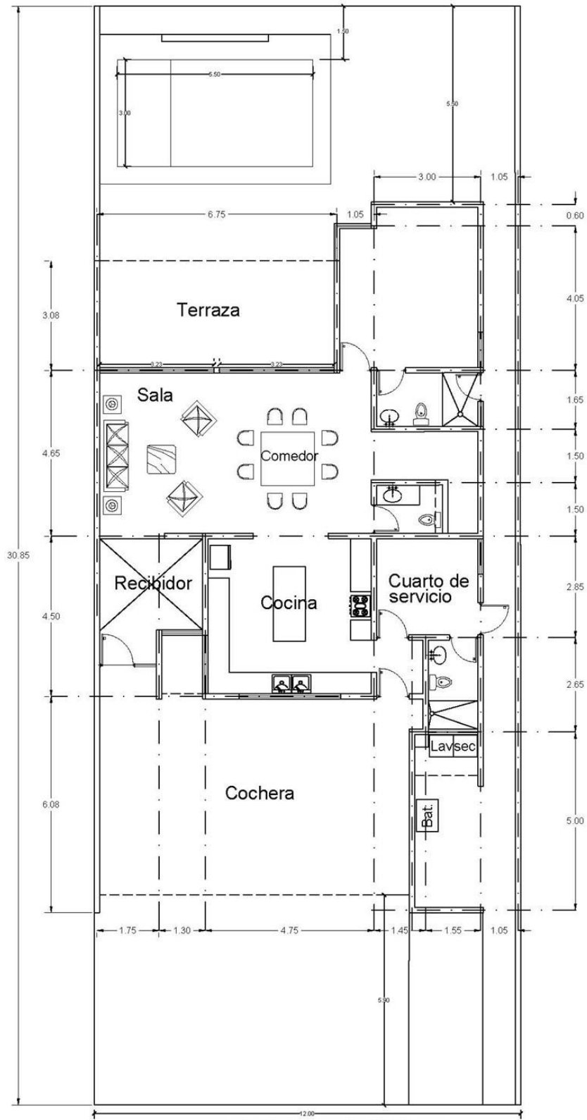
PLANTA ARQUITECTONICA P.B. 192.83 m 2
