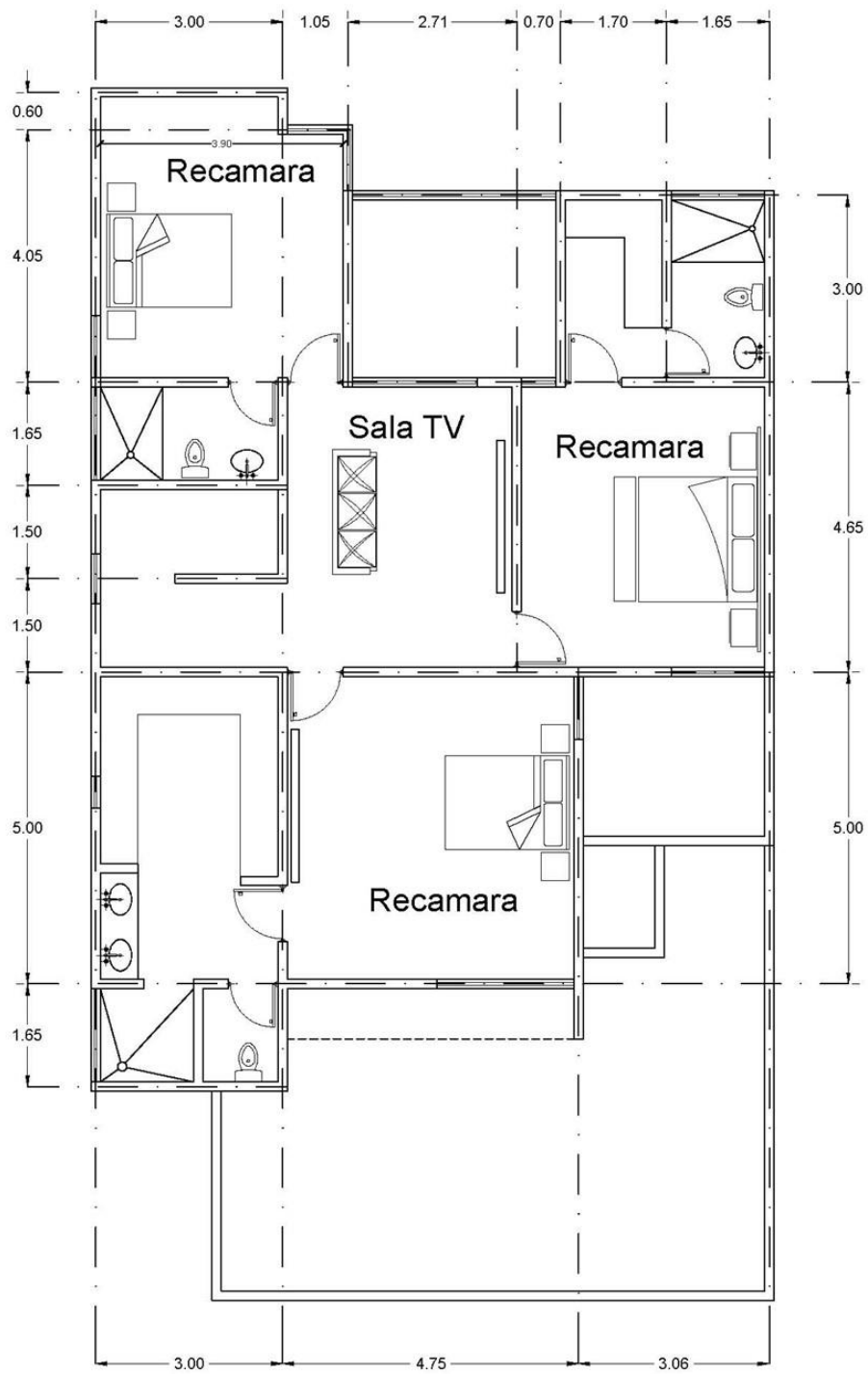
PLANTA ARQUITECTONICA P.A.
