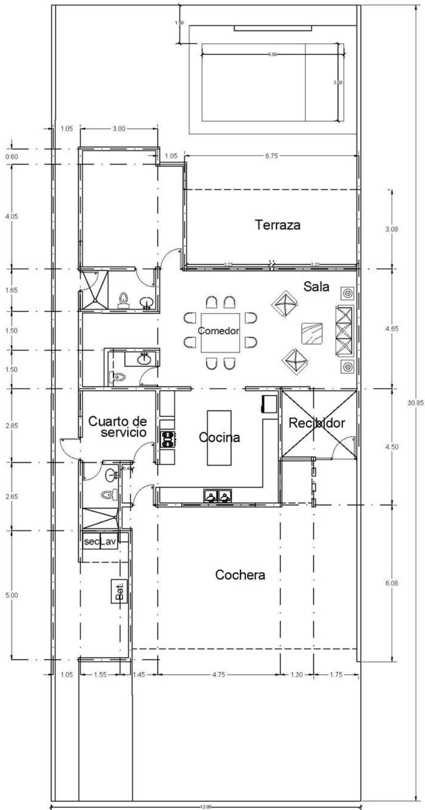
PLANTA ARQUITECTONICA P.B. 192.85 m2
