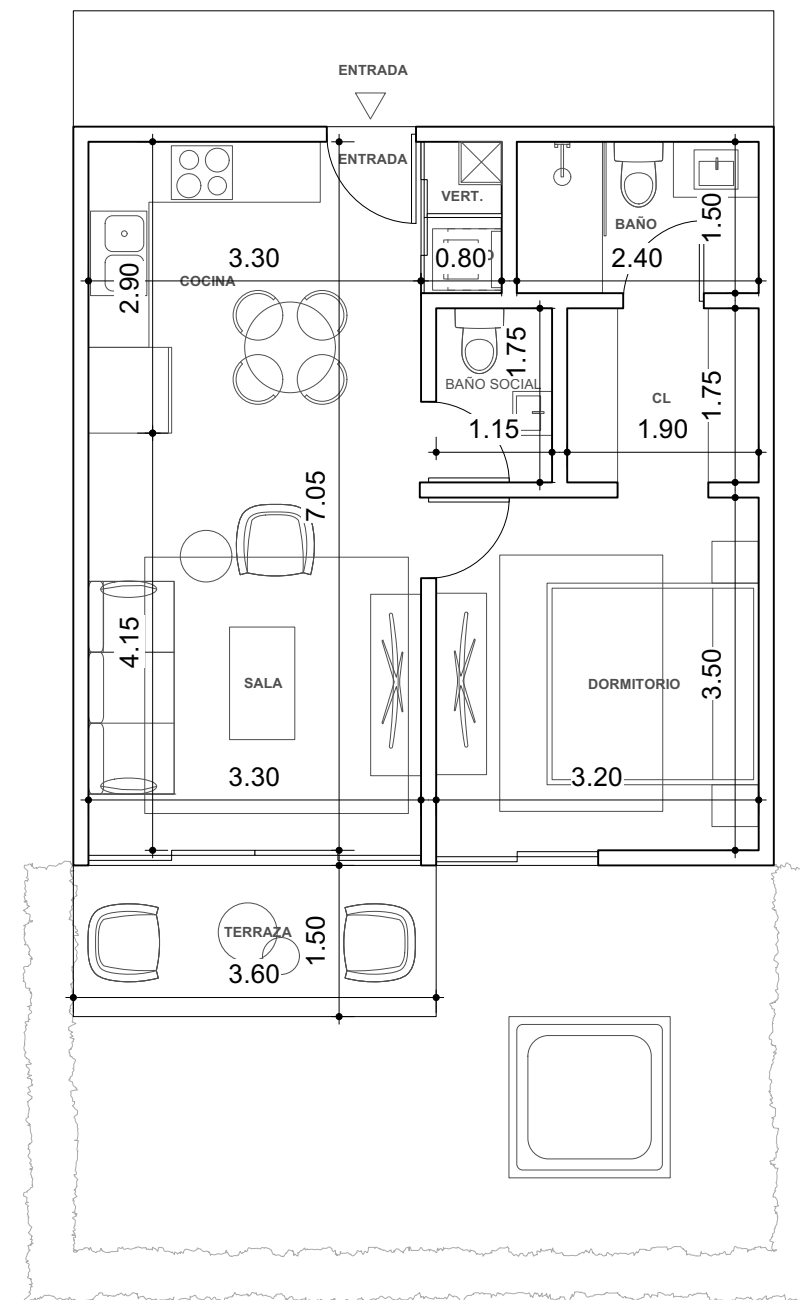
PLANTA DIMENSIONADA
