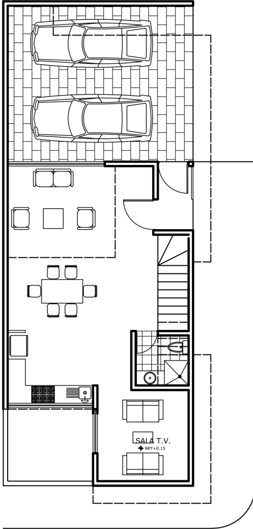
PLANTA BAJA
