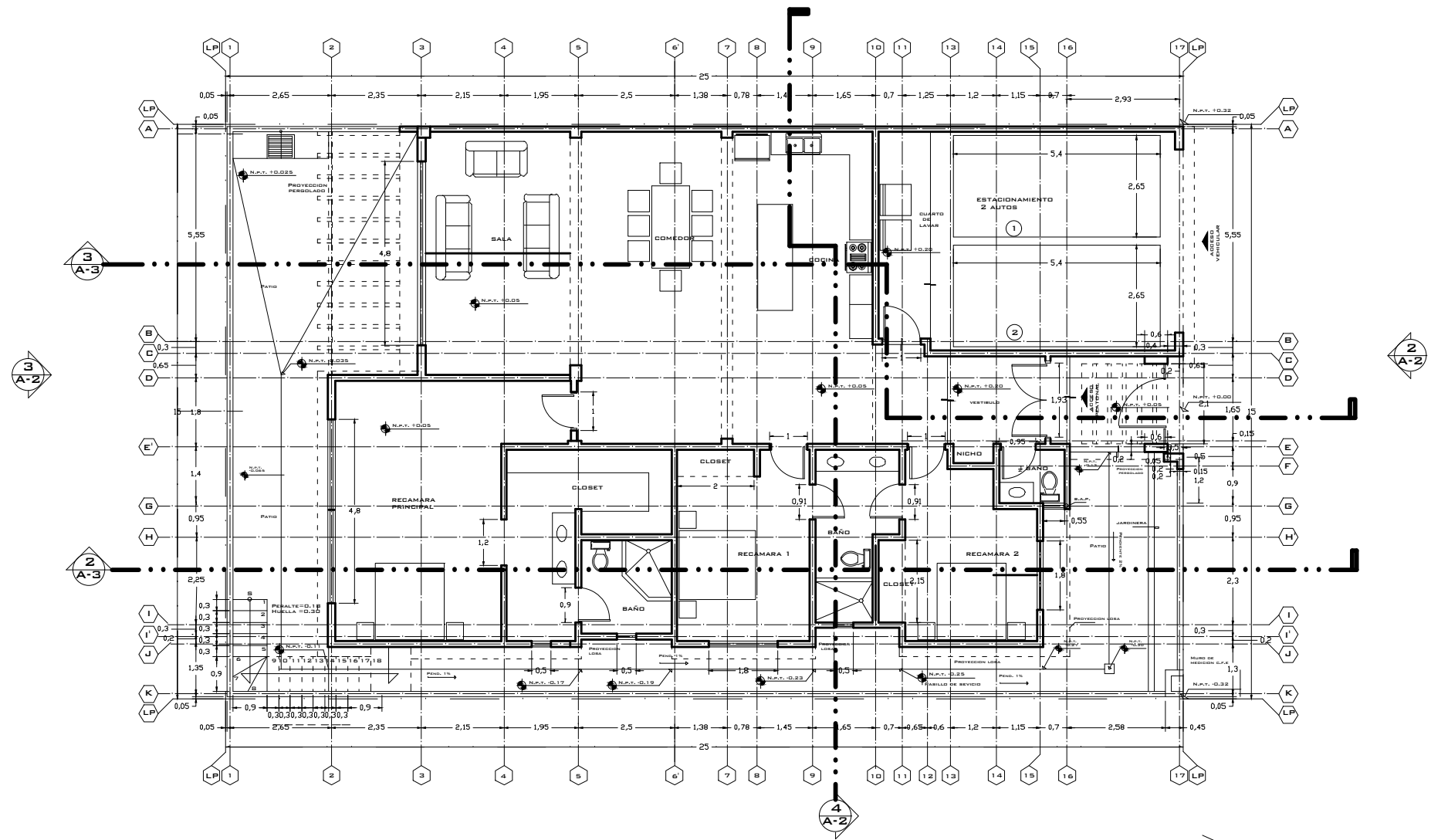
PLANTA ARQUITECTONICA ESCALA 1 = 50 METROS CUADRADOS DE CONSTRUCCION = 280.00 M2
