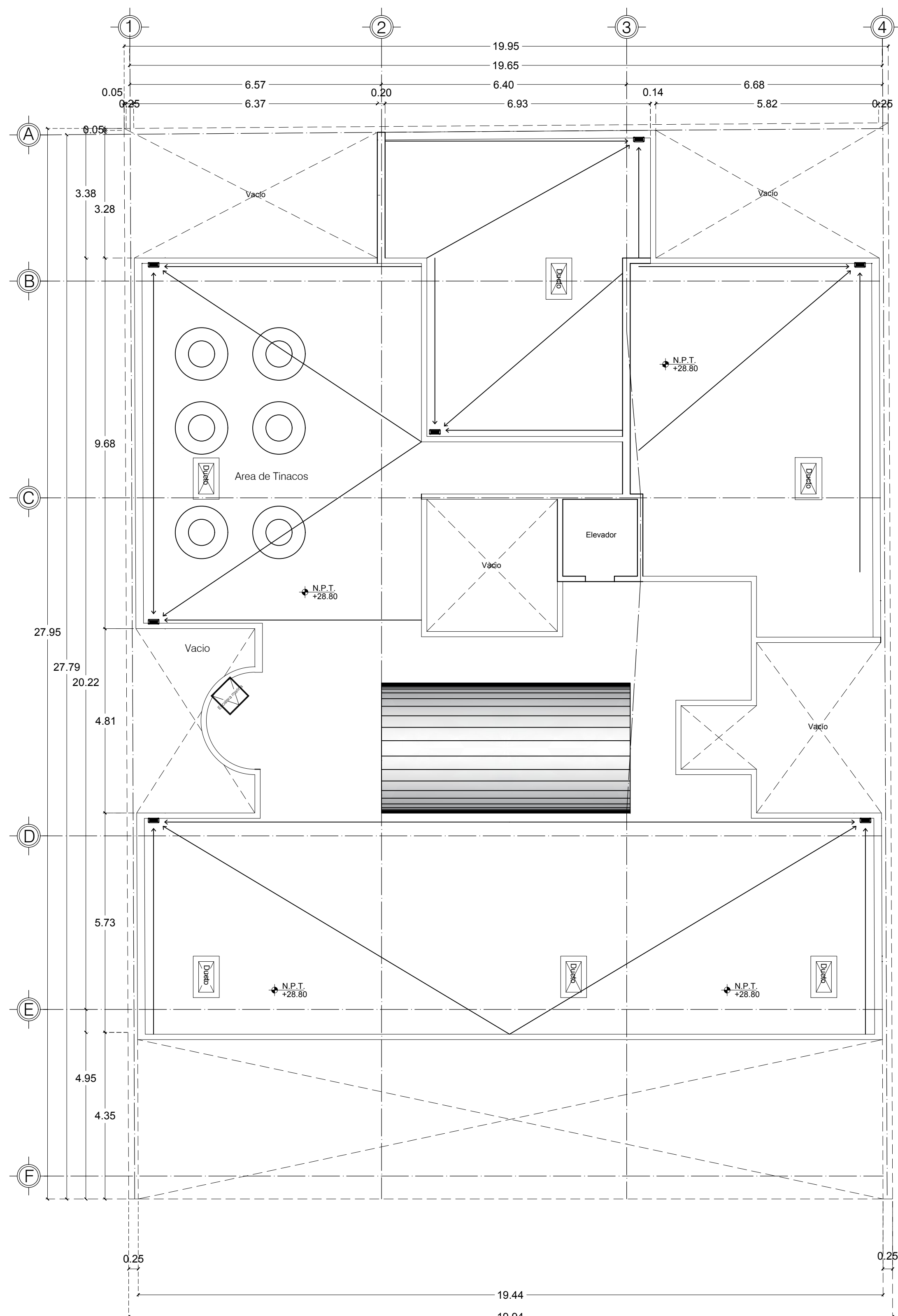
PLANTA AZOTEA
