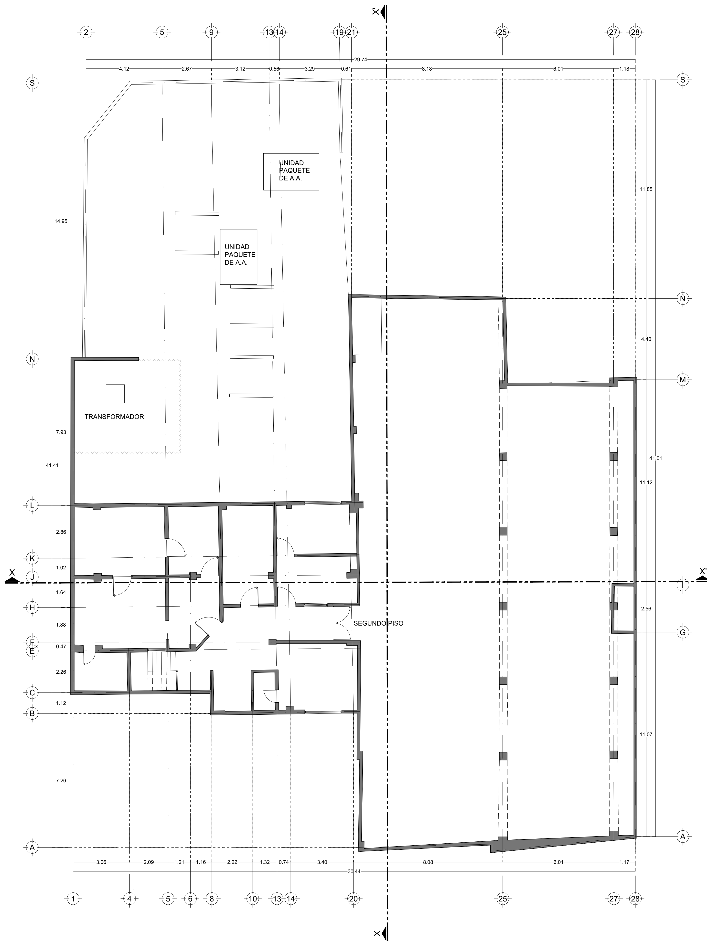
01 SEGUNDO PISO 1:100
