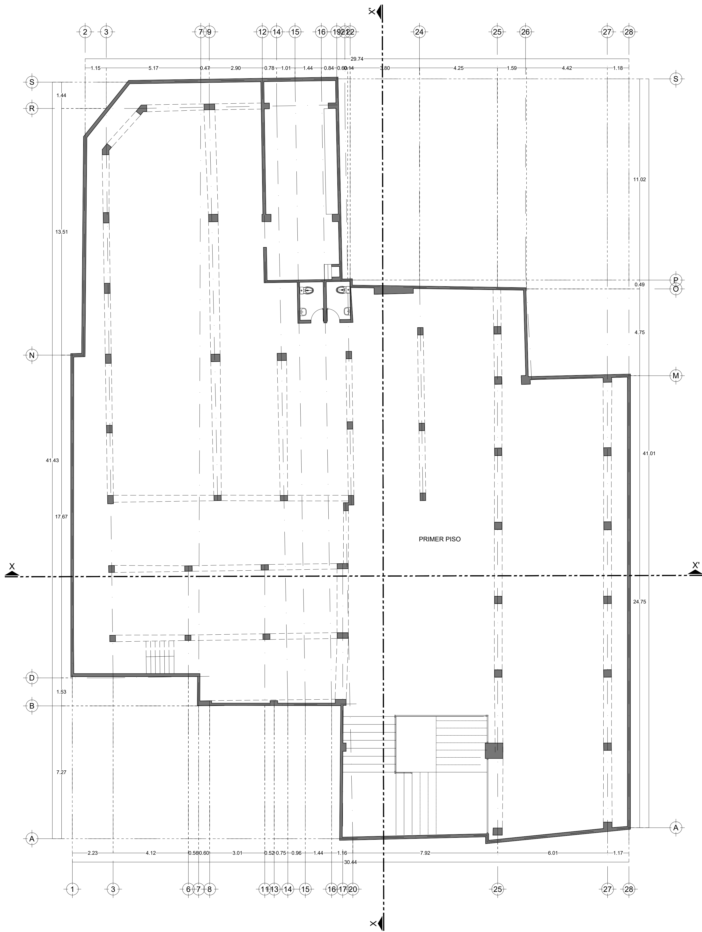
01 PRIMER PISO 1:100
