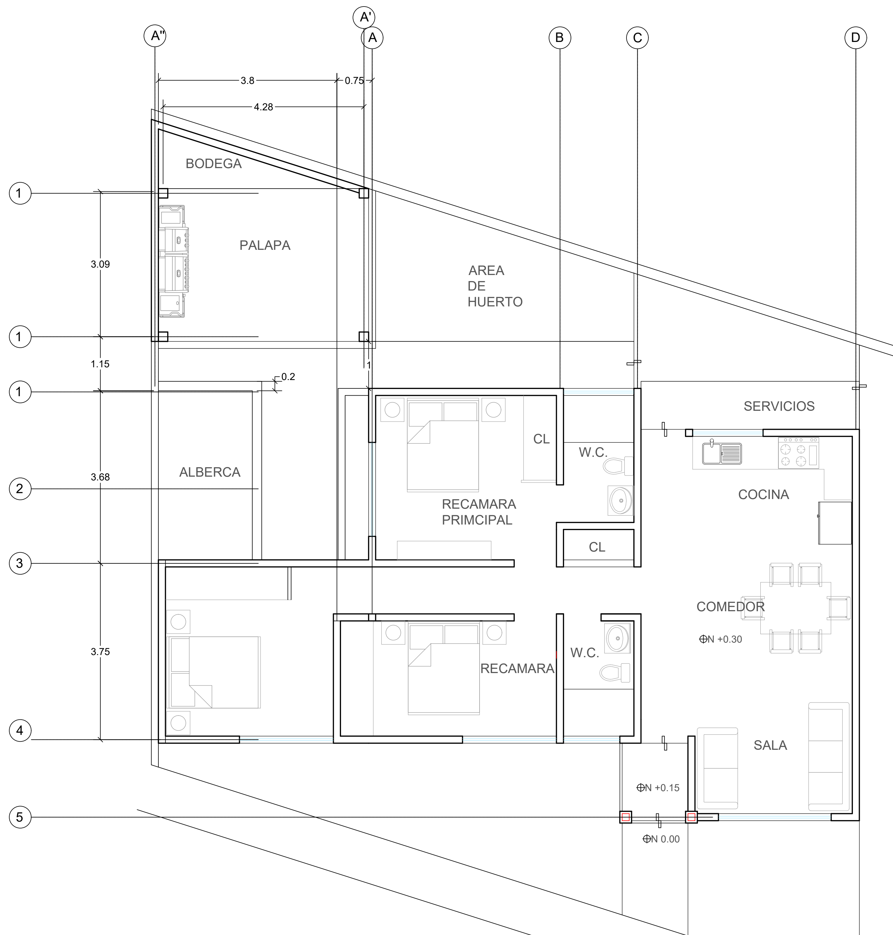
PLANTA ARQUITECTONICA ADITIVAS ESC 1:50
