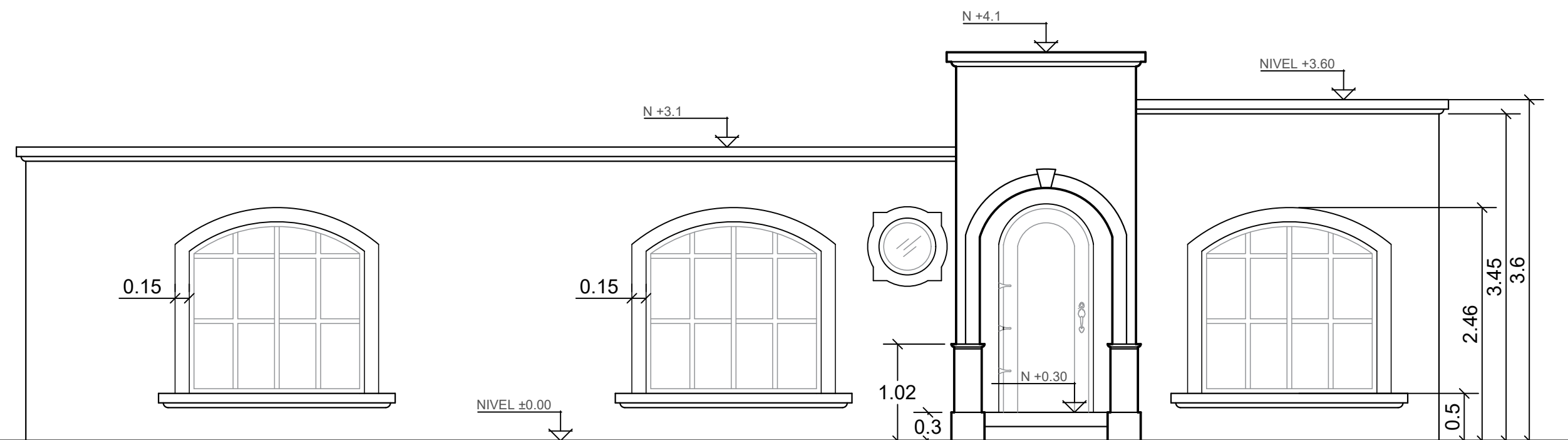
FACHADA PRINCIPAL ESC. 1:50
