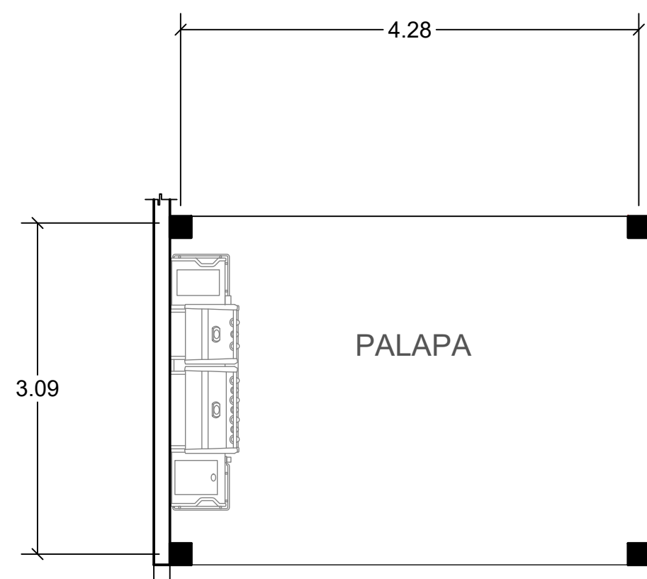
PLANTA PALAPA ESC. 1:50
