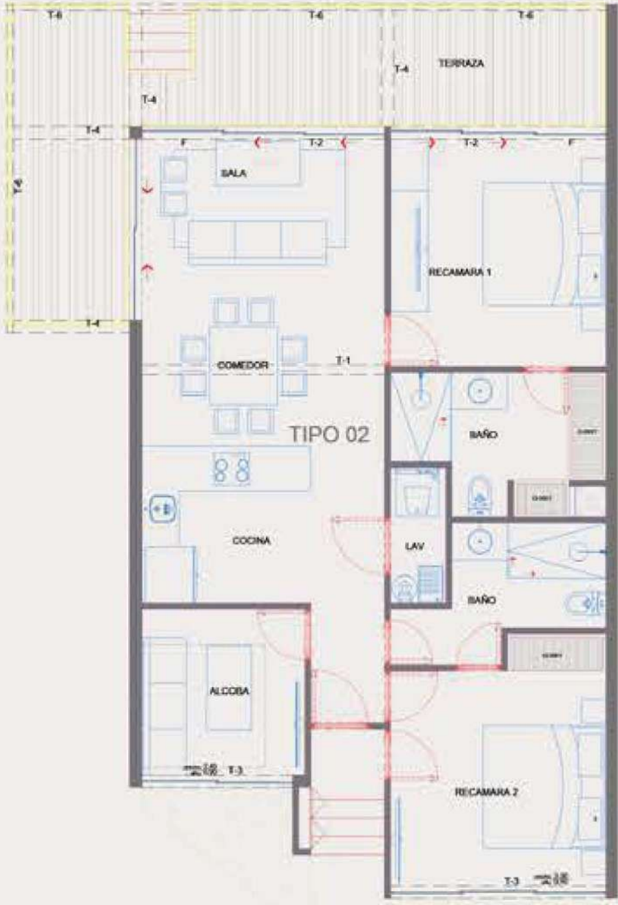
PLANTA DEPARTAMENTO
