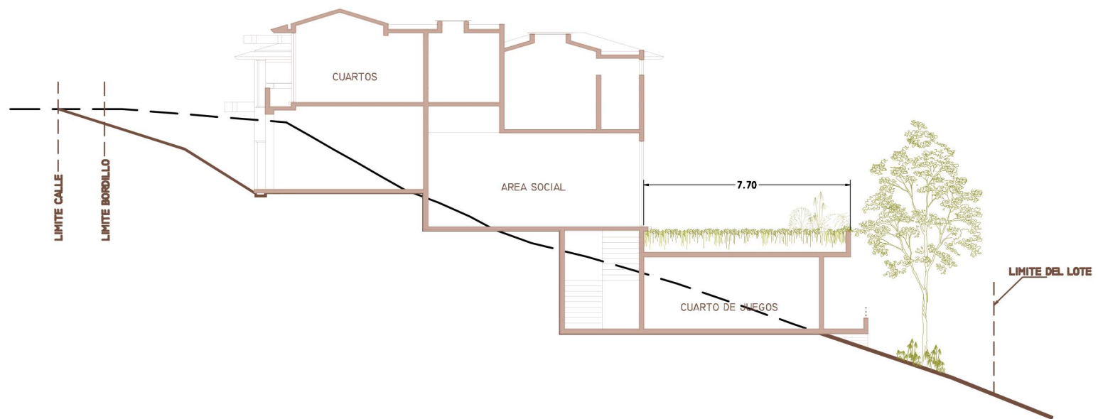
SECCION LOTE 1 OPCION "A" ESC. 1:200
