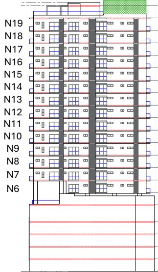
PERFIL LATERAL DERECHO TORRE LUXOR
