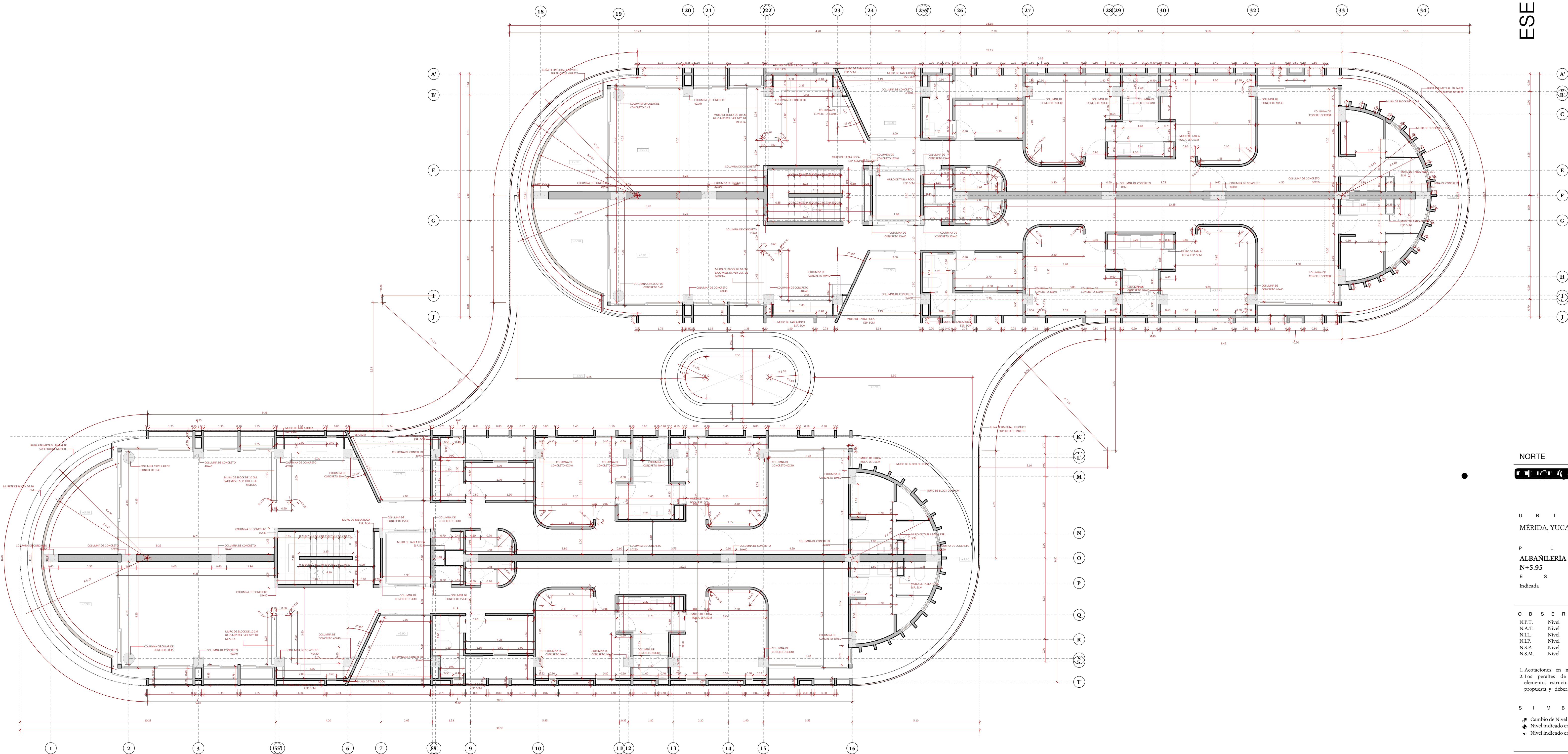
1 | ALB - N+5.95 - DEPTO CLÁSICO ESC 1 : 75
