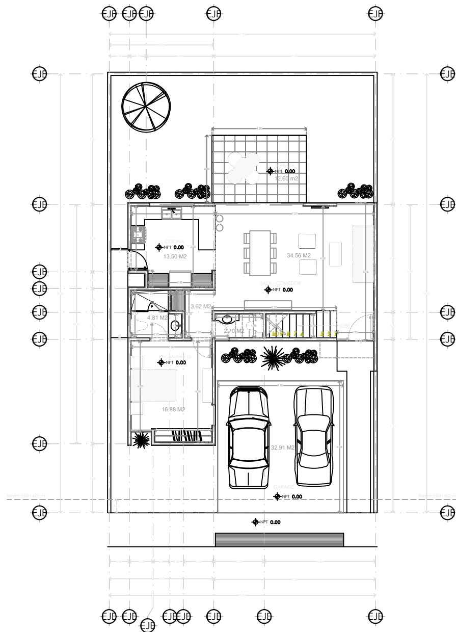
PLANTA BAJA
