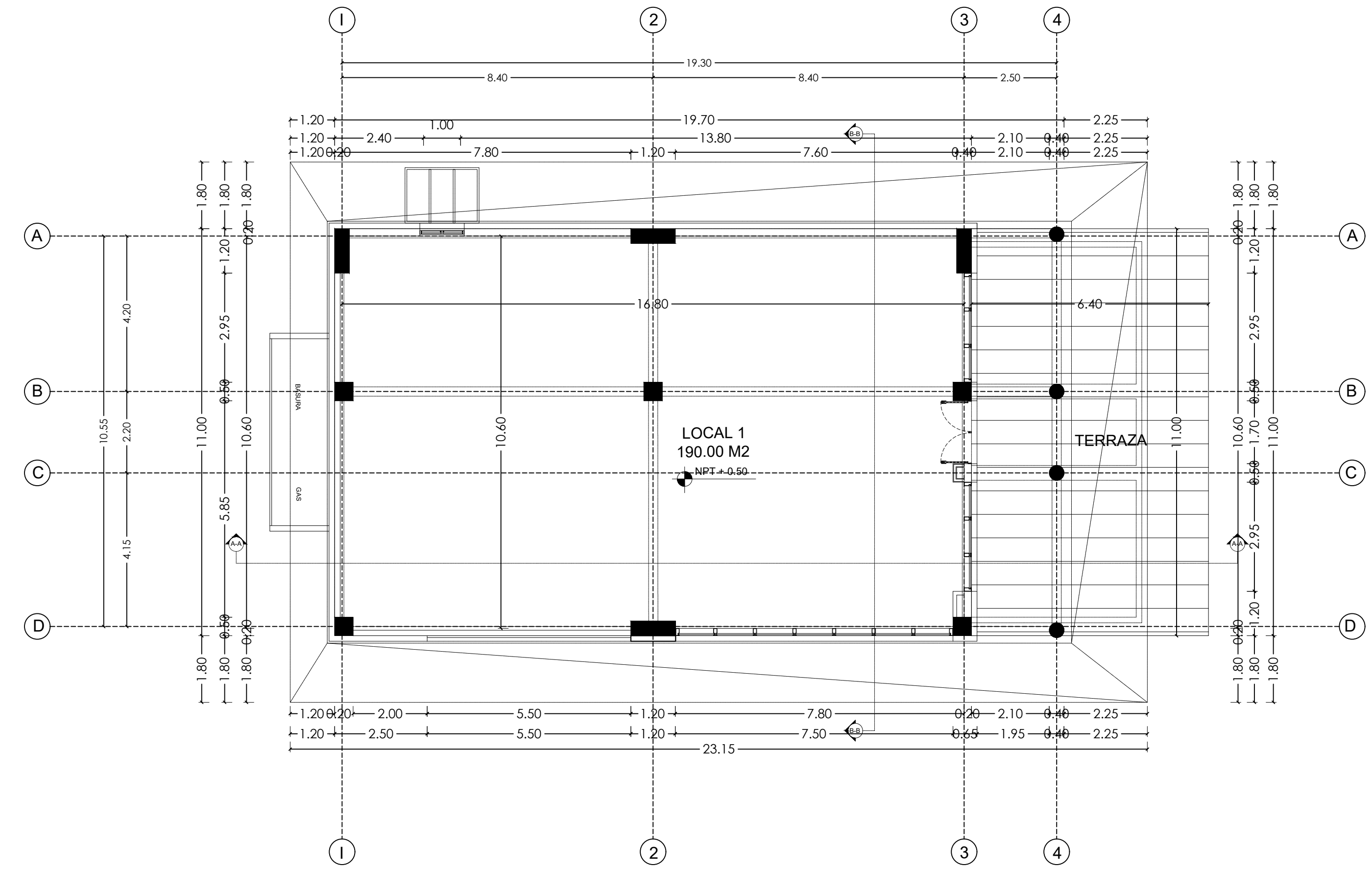
PLANTA DIMENSIONADA 1ER NIVEL LOCAL 1 THE PLAZA ESC: 1:100
