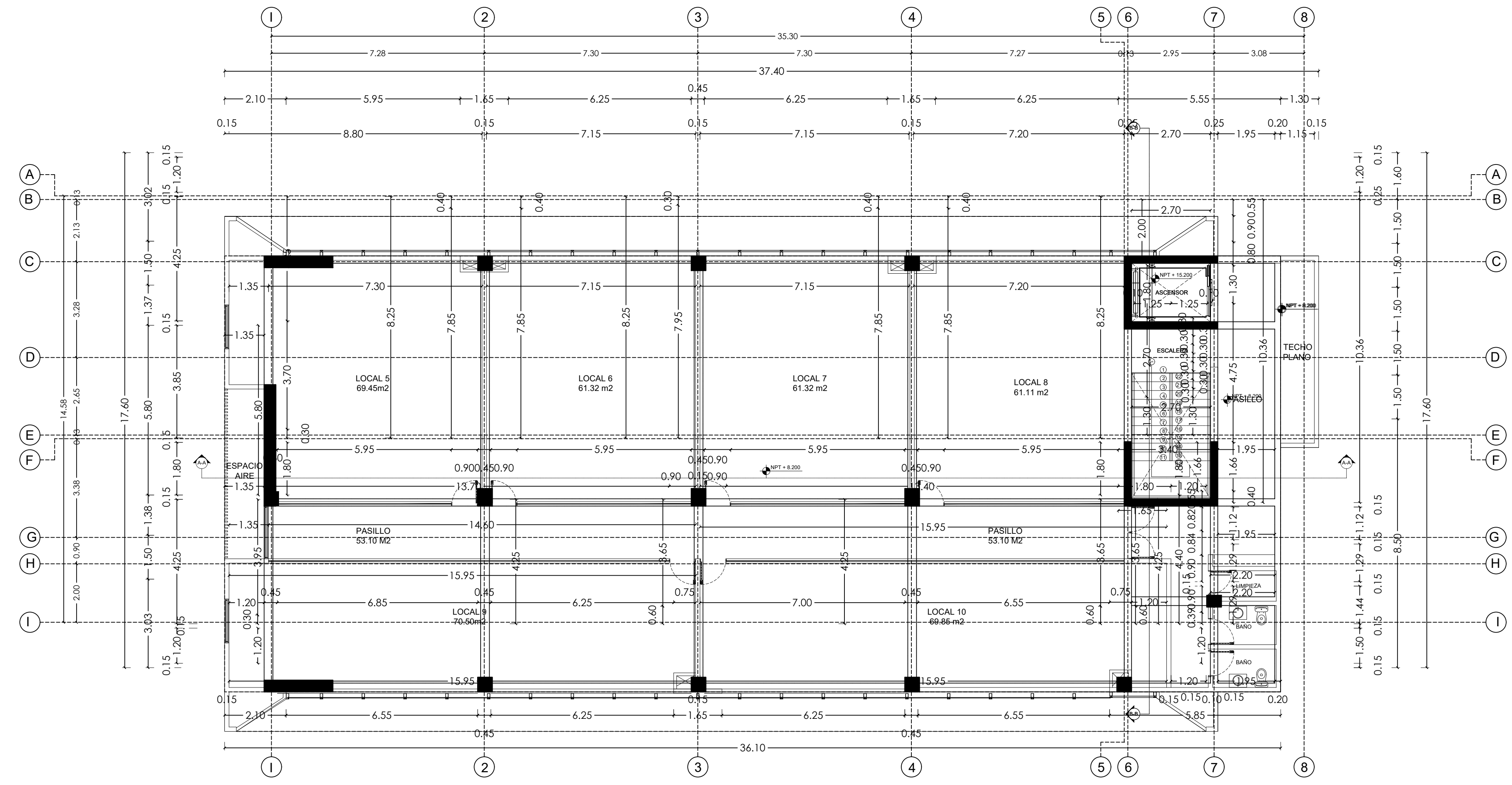
PLANTA DIMENSIONADA 3ER NIVEL EDIFICIO CORPORATIVO THE PLAZA ESC: 1:100
