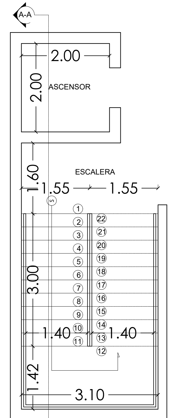
DELLATE DE ESCALERA / BLOQUE L THE PLAZA ESC: 1:50
