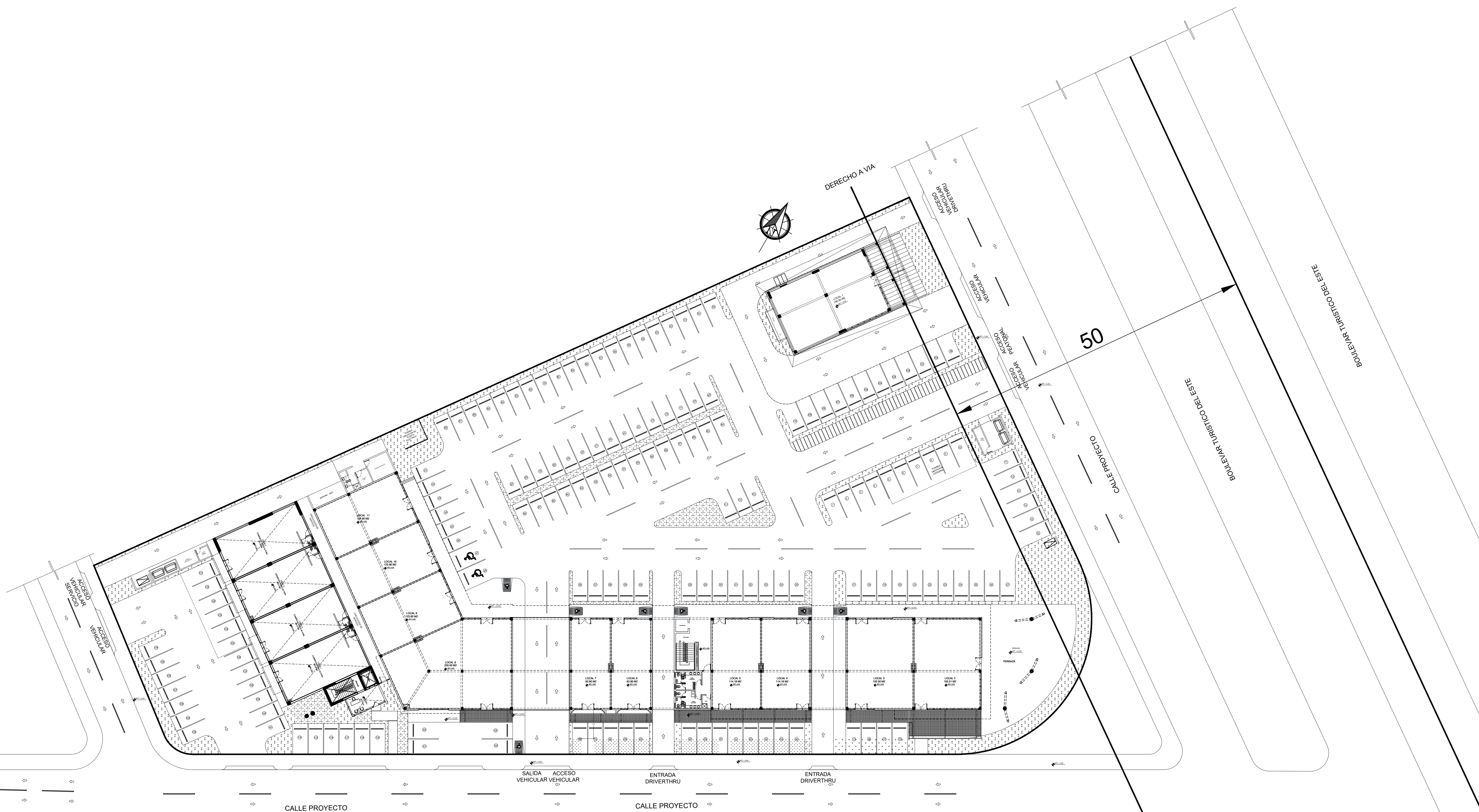
PLANTA ARQUITECTONICA DE CONJUNTO 1ER NIVEL THE PLAZA ESC: 1:300
