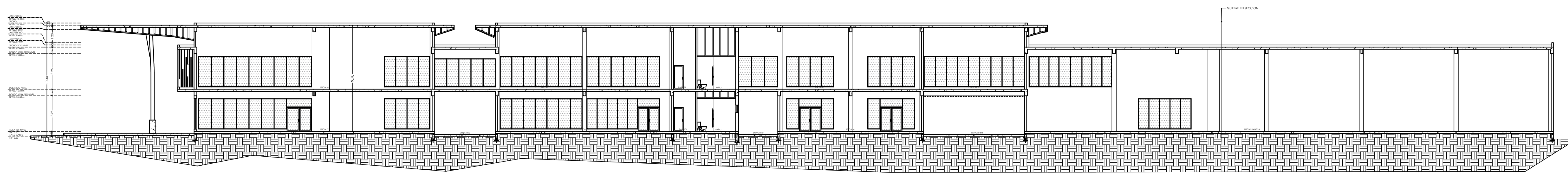
SECCION A-A BLOQUE I THE PLAZA ESC: 1/200
