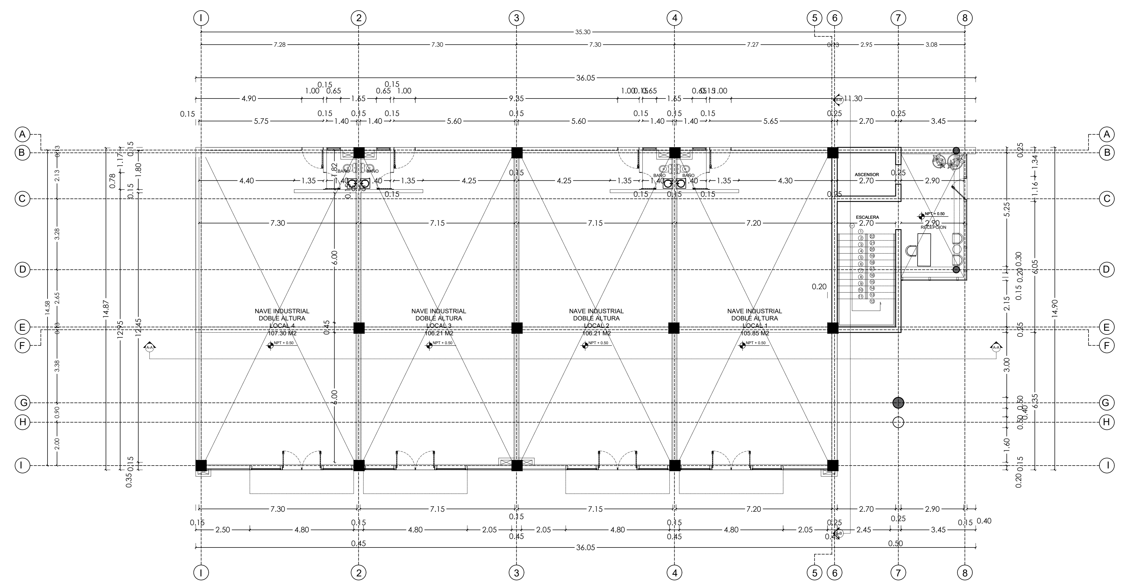
PLANTA DIMENSIONADA 1ER NIVEL EDIFICIO CORPORATIVO THE PLAZA ESC: 1:100
