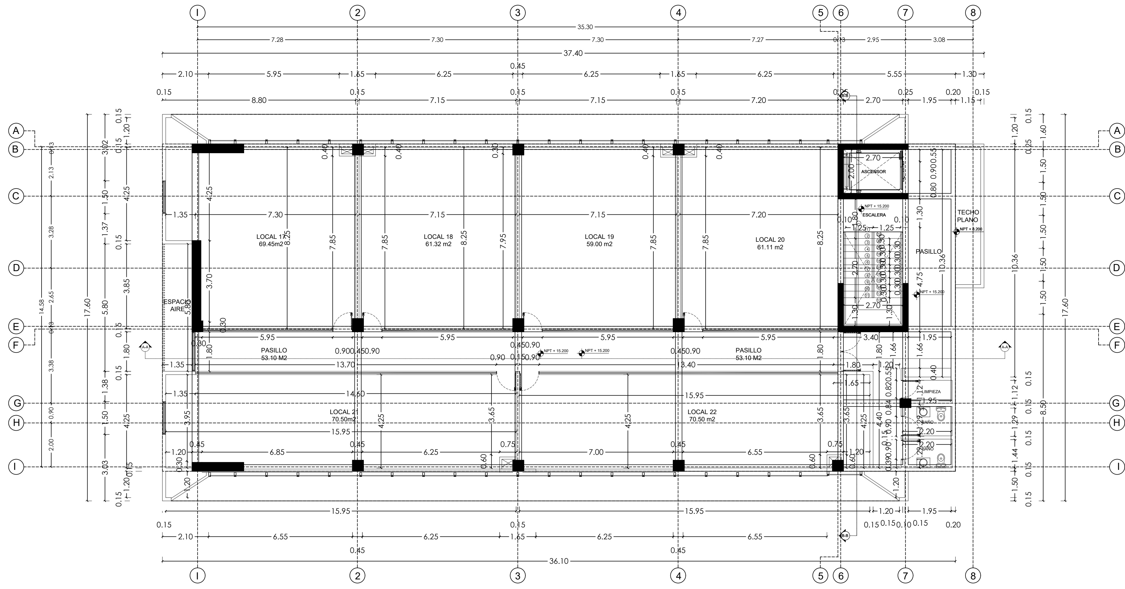
PLANTA ARQUITECTONICA 5TO NIVEL EDIFICIO CORPORATIVO THE PLAZA ESC: 1:100
