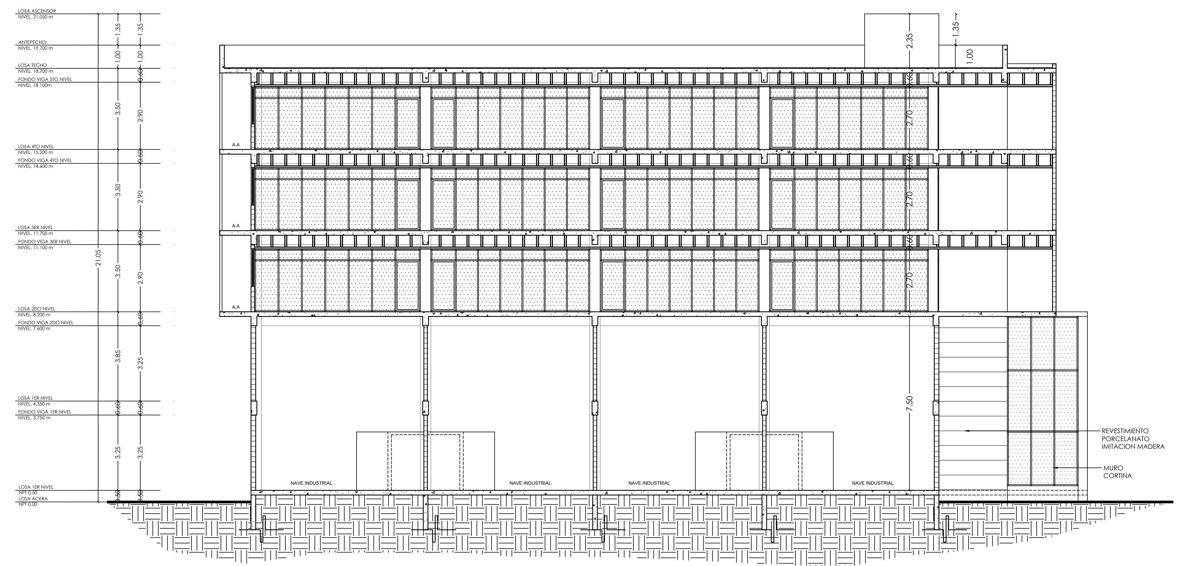
SECCION A-A EDIFICIO CORPORATIVO THE PLAZA ESC: 1:150
