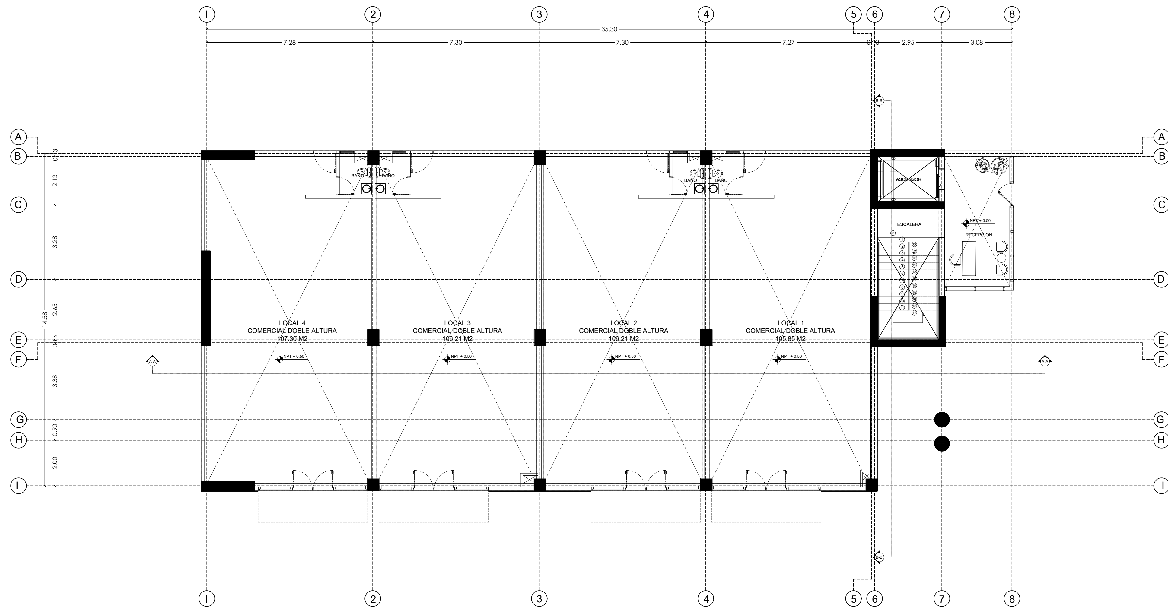
PLANTA ARQUITECTONICA 1ER NIVEL EDIFICIO CORPORATIVO THE PLAZA ESC: 1:100
