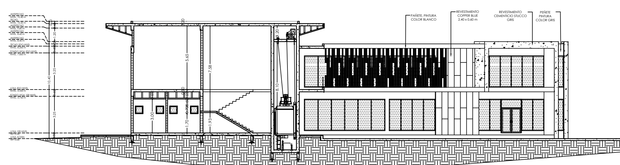
SECCION B-B BLOQUE I THE PLAZA ESC: 1/200
