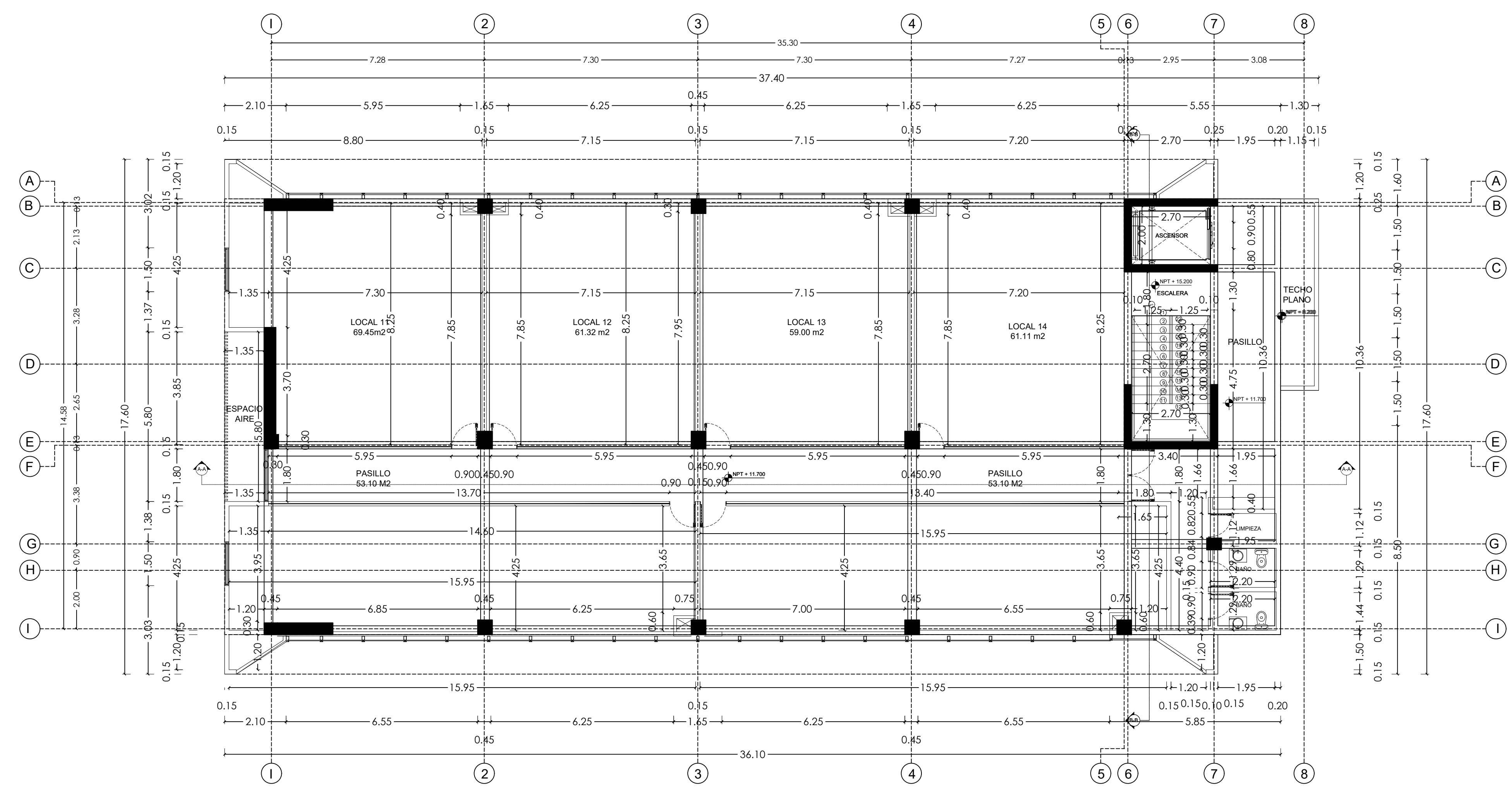
PLANTA DIMENSIONADA 4TO NIVEL EDIFICIO CORPORATIVO THE PLAZA ESC: 1:100
