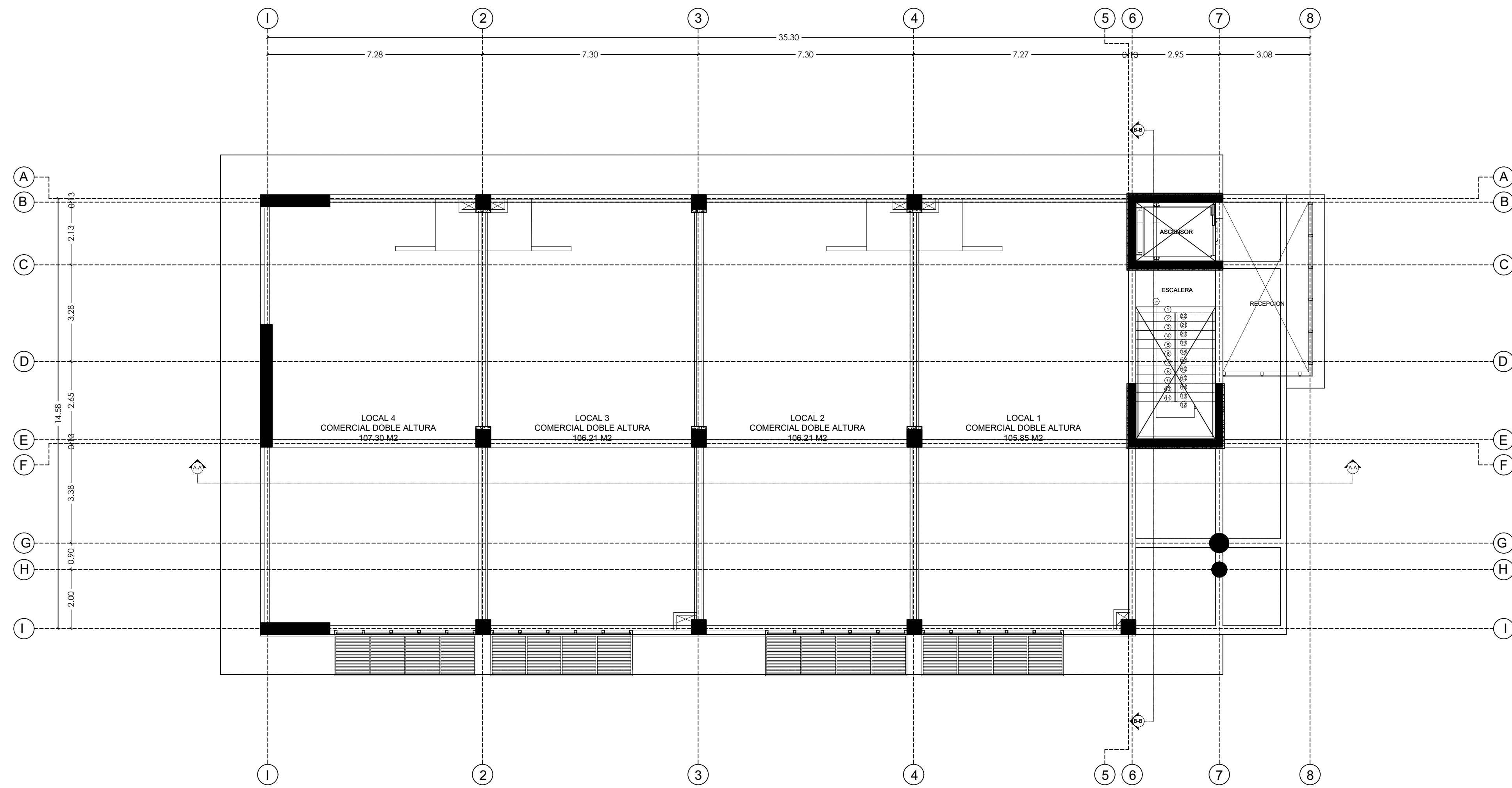
PLANTA ARQUITECTONICA 2DO NIVEL EDIFICIO CORPORATIVO THE PLAZA ESC: 1:100
