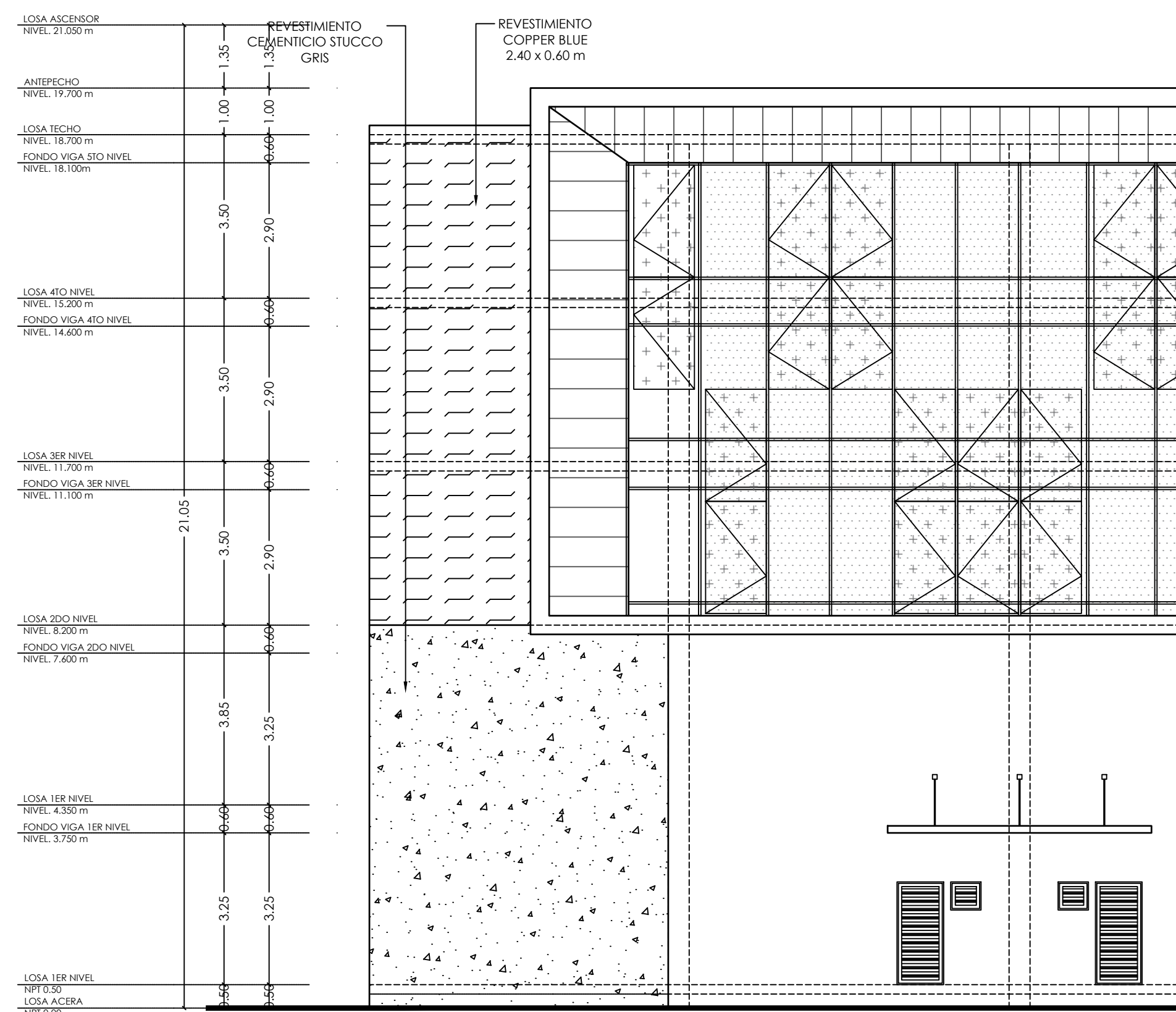
ELEVACION LATERAL DERECHO EDIFICIO CORPORATIVO THE PLAZA ESC: 1:100
