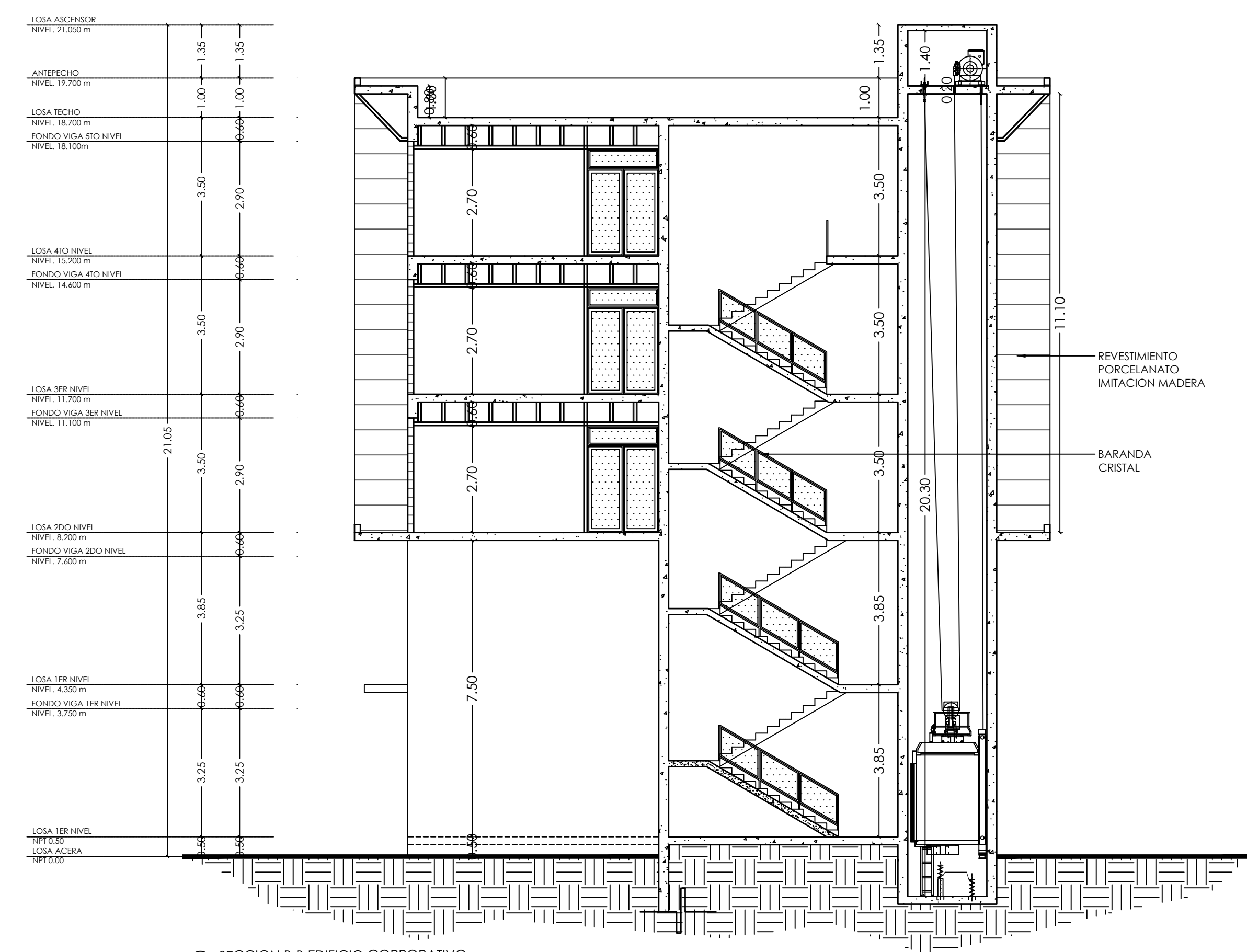
SECCION B-B EDIFICIO CORPORATIVO THE PLAZA ESC: 1:150
