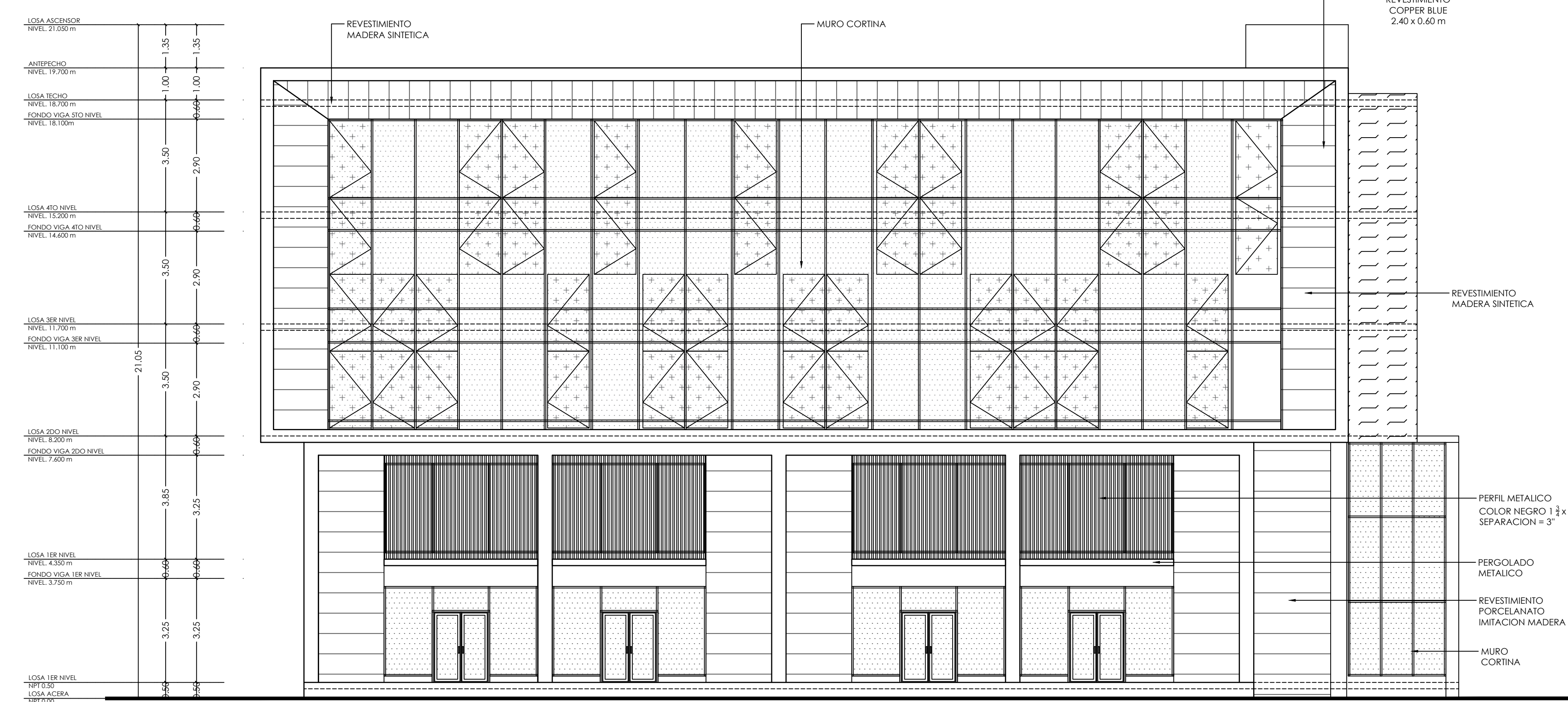
ELEVACION LATERAL IZQUIERDO EDIFICIO CORPORATIVO THE PLAZA ESC: 1:100
