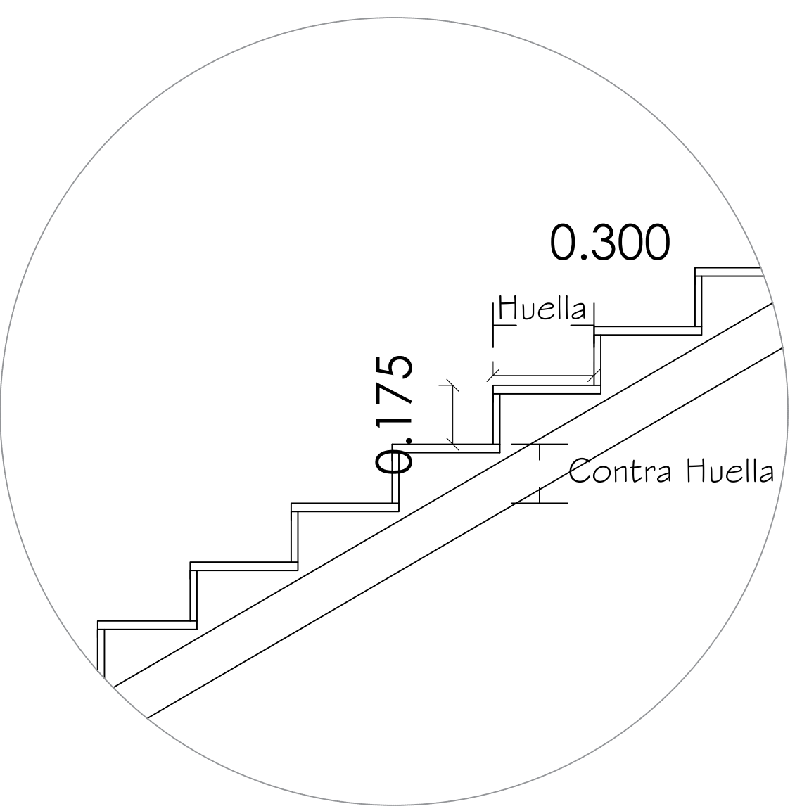
DELLATE PELDAÑOS THE PLAZA ESC:
