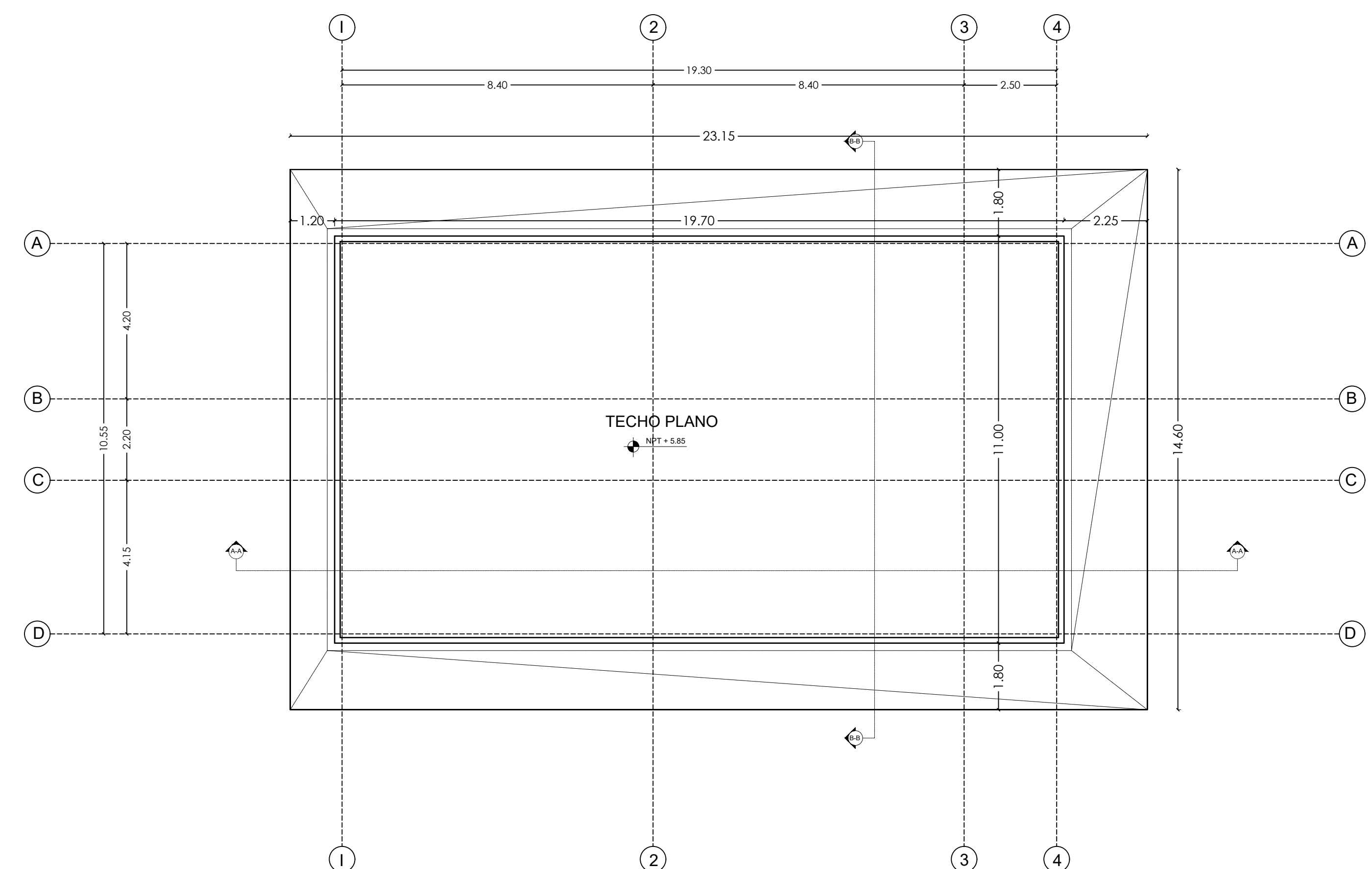
PLANTA DIMENSIONADA TECHO LOCAL 1 THE PLAZA ESC: 1:100
