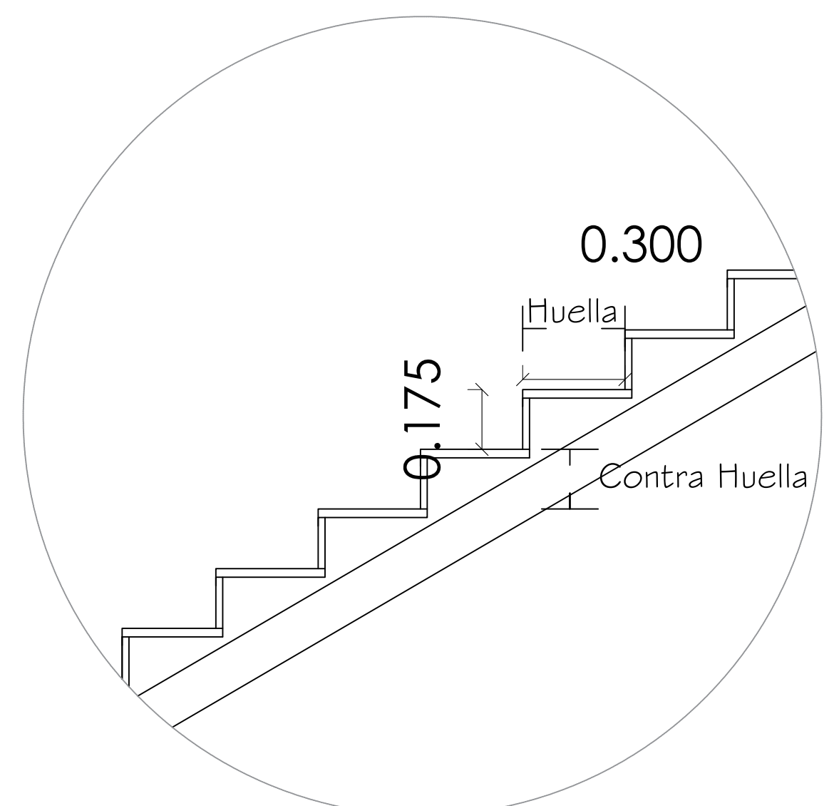
DELLATE Peldaños THE PLAZA ESC:
