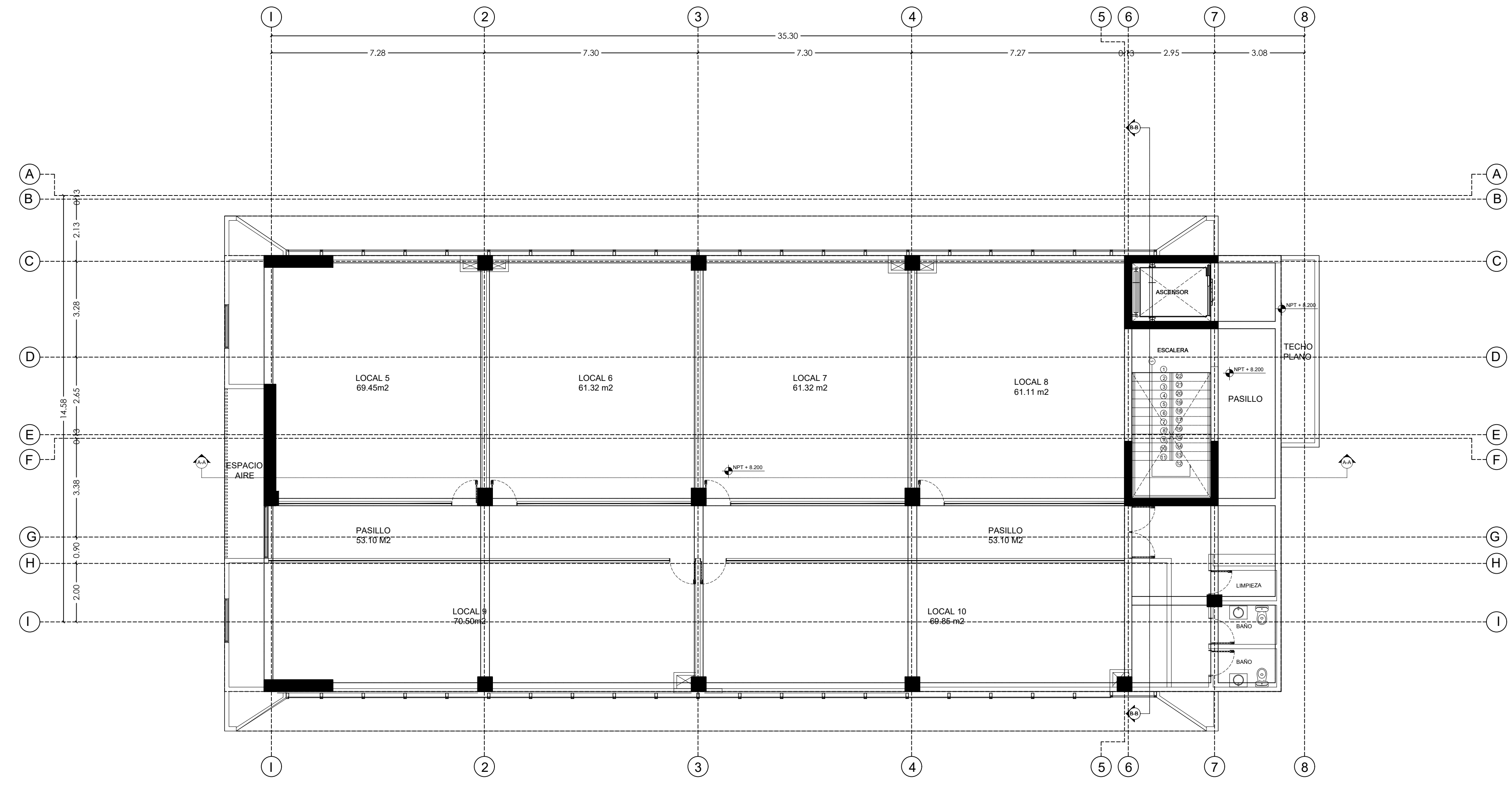
PLANTA ARQUITECTONICA 3ER NIVEL EDIFICIO CORPORATIVO THE PLAZA ESC: 1:100
