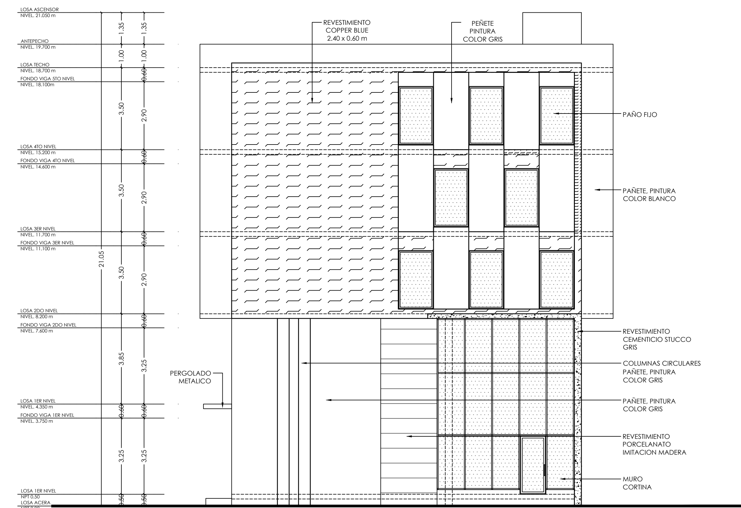
ELEVACION FRONTAL EDIFICIO CORPORATIVO THE PLAZA ESC: 1:100
