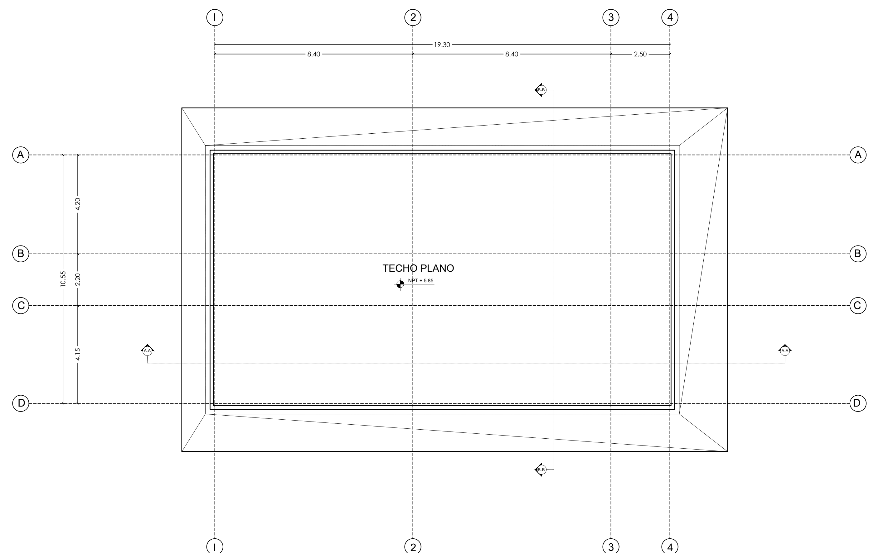
PLANTA ARQUITECTONICA TECHO LOCAL 1 THE PLAZA ESC: 1:100
