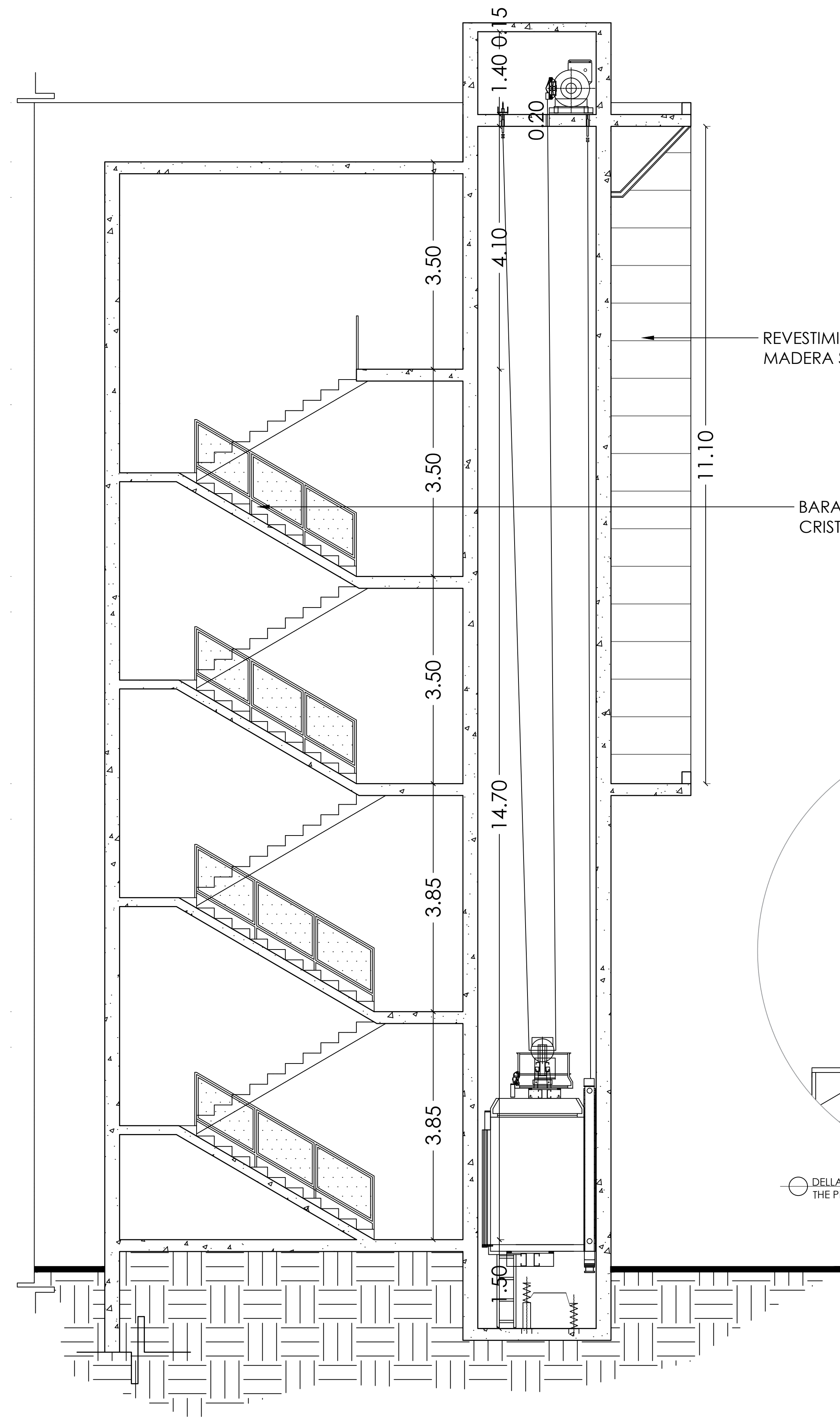
SECCION A-A DE ESCALERA / ASCENSOR EDIFICIO CORPORATIVO THE PLAZA ESC: 1:50
