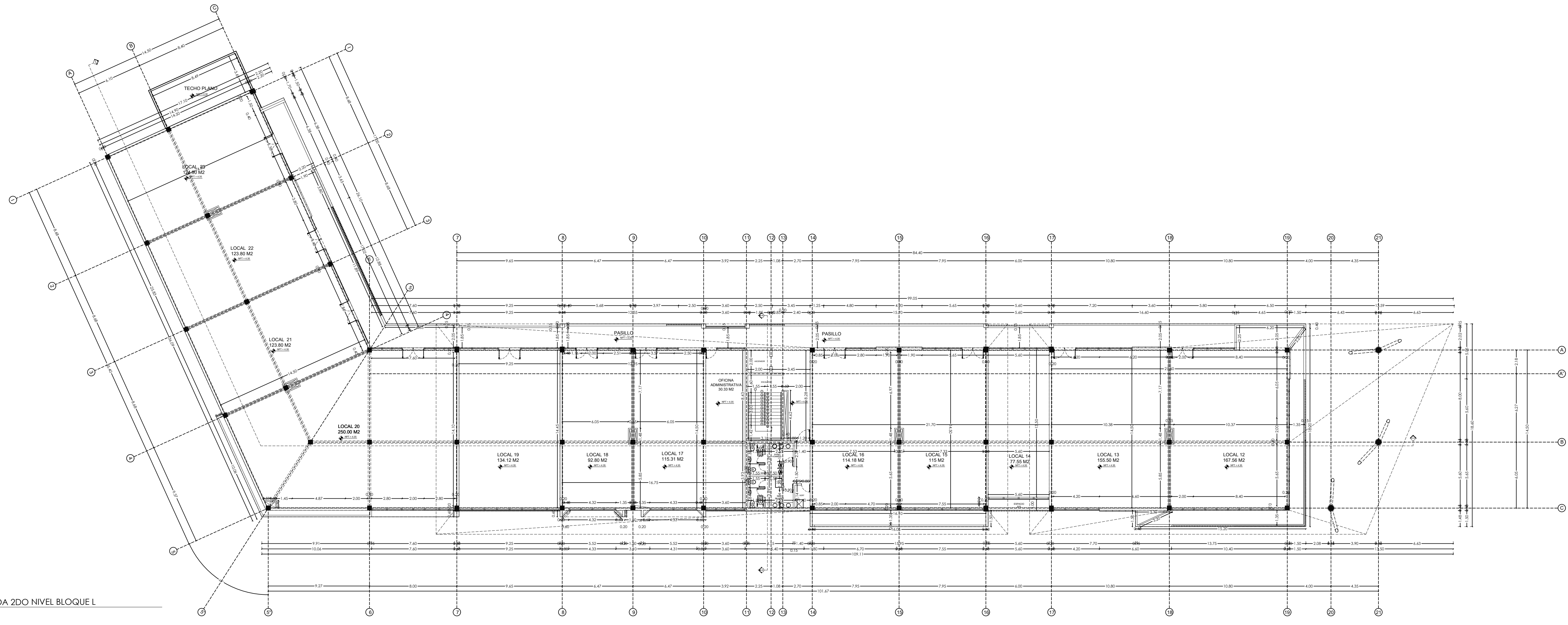
PLANTA ARQUITECTONICA 2DO NIVEL BLOQUE L THE PLAZA ESC: 1:200
