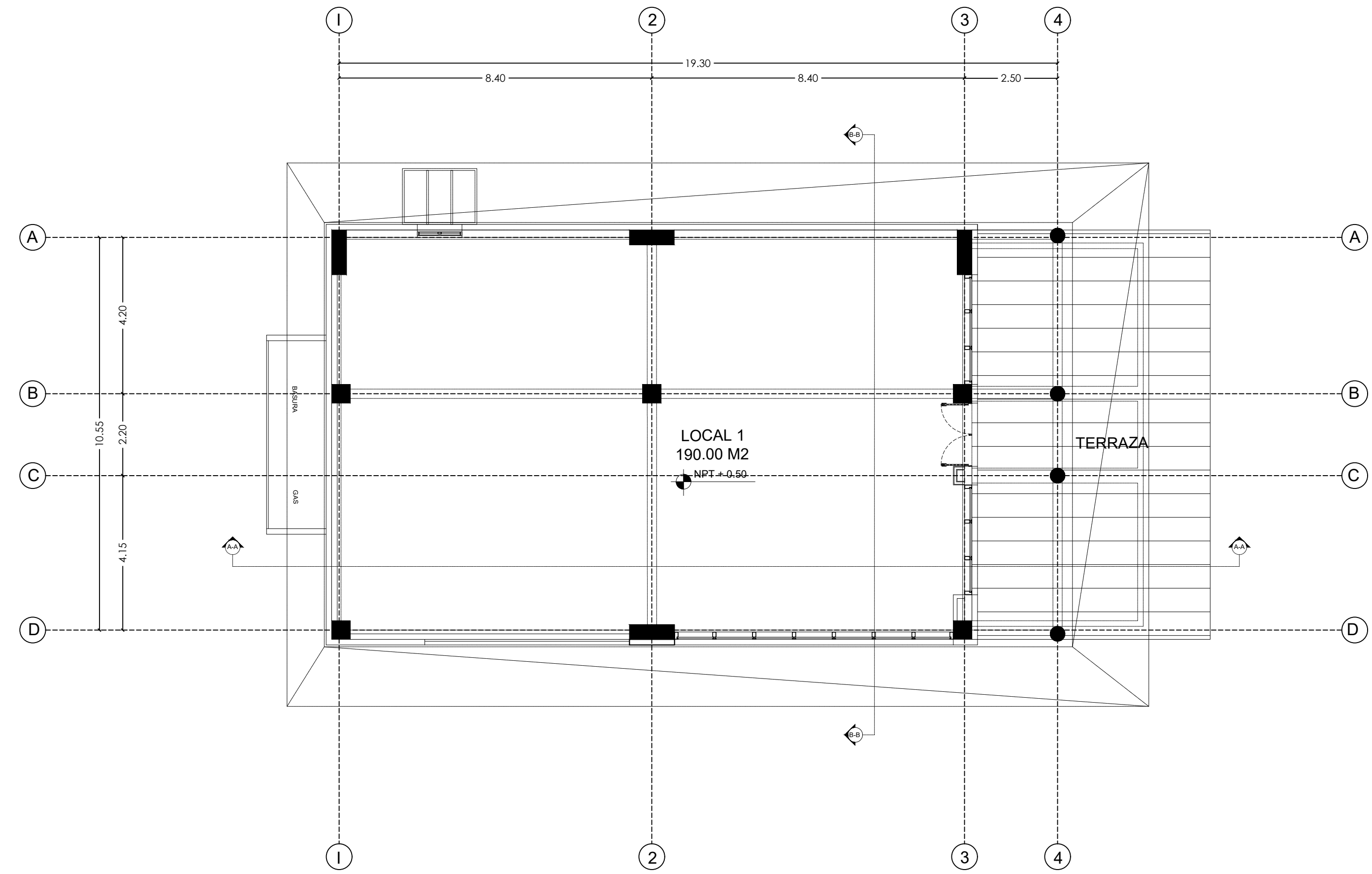
PLANTA ARQUITECTONICA 1ER NIVEL LOCAL 1 THE PLAZA ESC: 1:100
