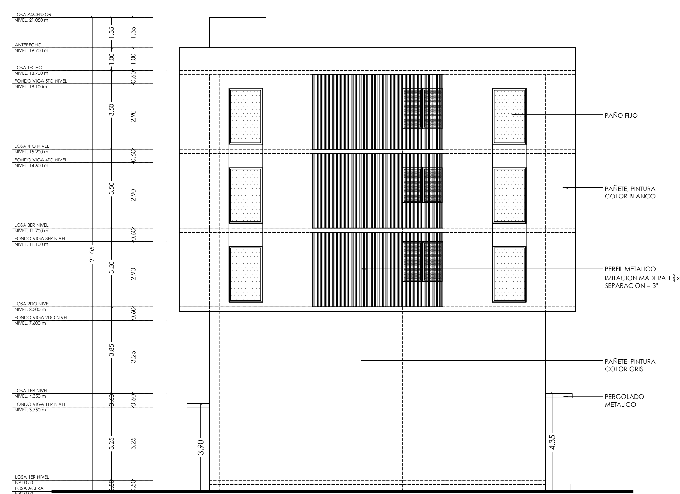
ELEVACION FRONTAL EDIFICIO CORPORATIVO THE PLAZA ESC: 1:100
