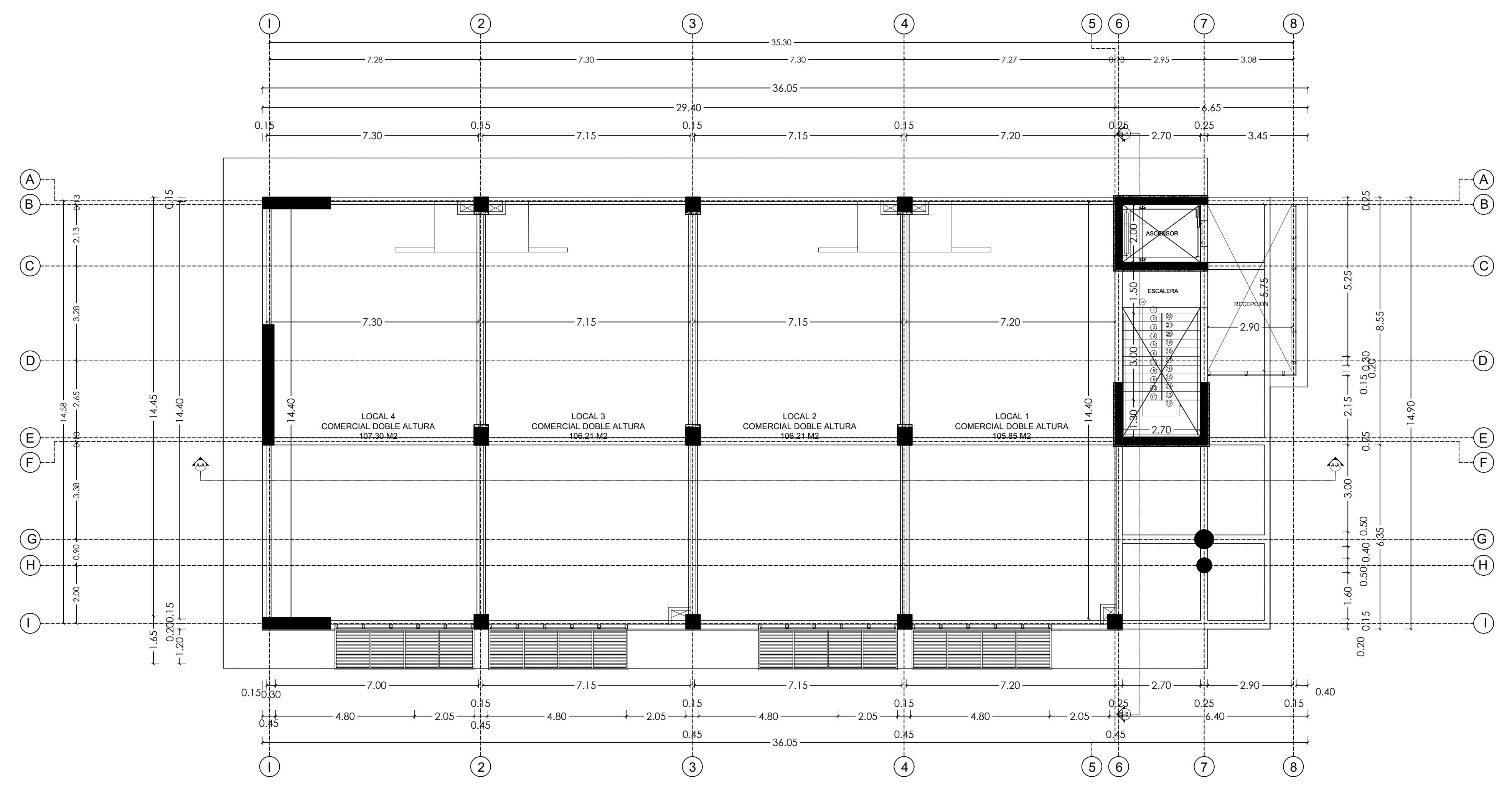
PLANTA DIMENSIONADA 2DO NIVEL EDIFICIO CORPORATIVO THE PLAZA ESC: 1:100
