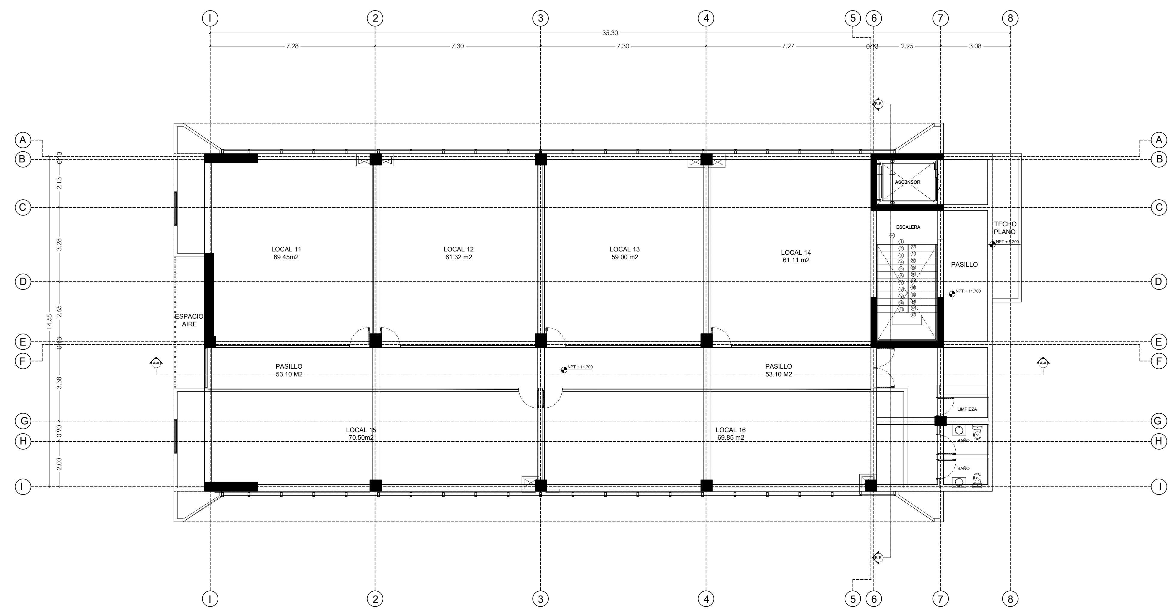
PLANTA ARQUITECTONICA 4TO NIVEL EDIFICIO CORPORATIVO THE PLAZA ESC: 1:100
