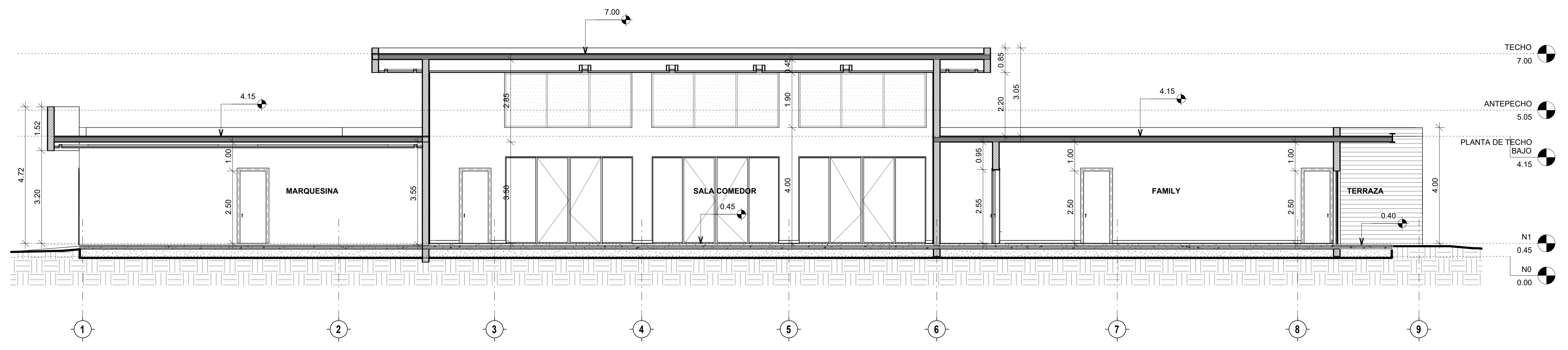
1 SECCION LONGITUDINAL ESC. 1 : 75 A102
