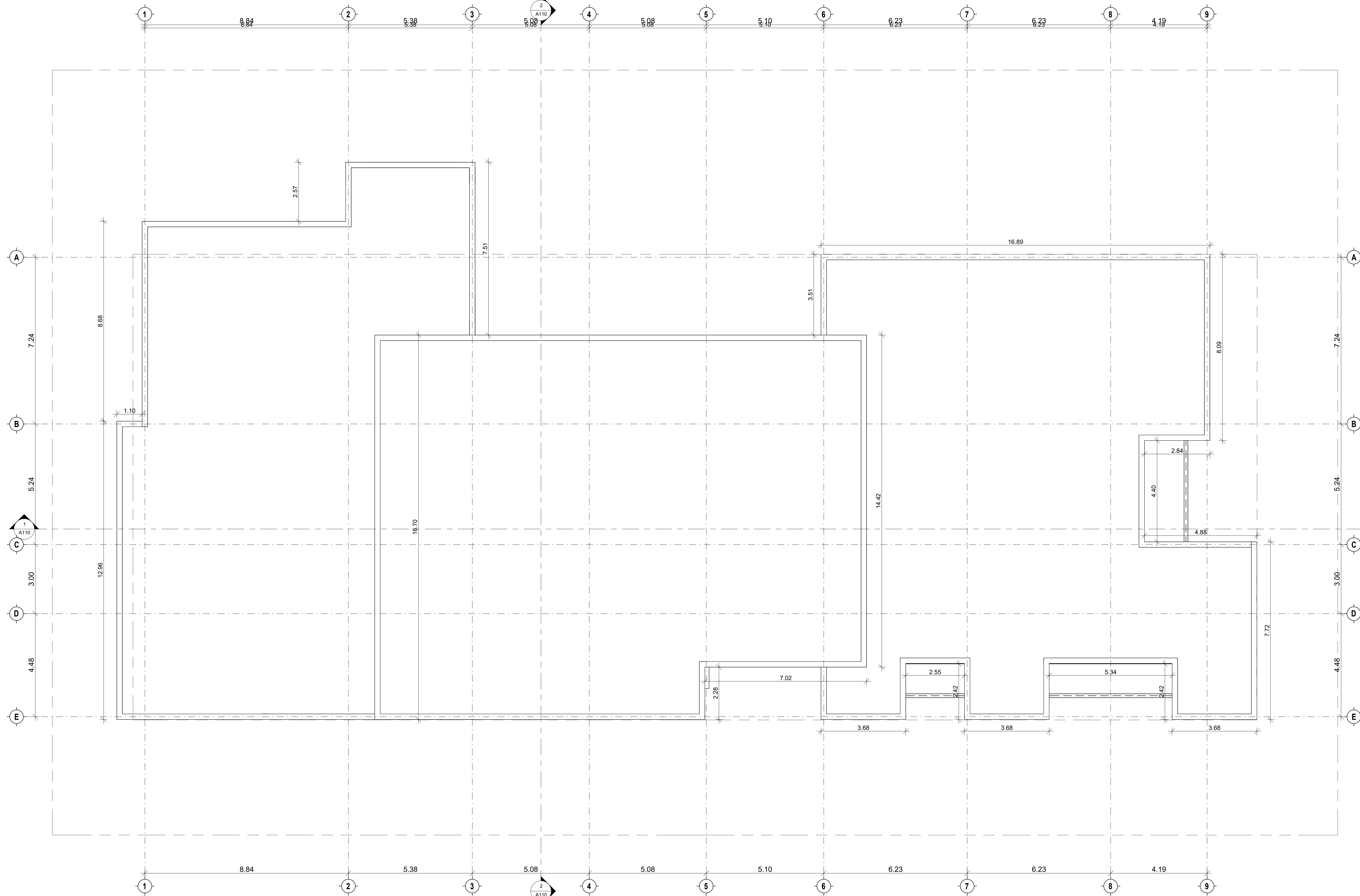
1 PLANTA DIMENSIONADA DE TECHO ESC.1:75
