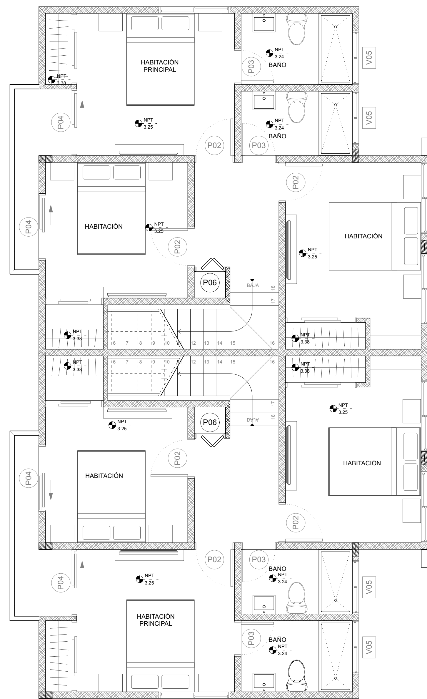
1 Planta Arquitectónica - Nivel 2 Scale: 1:50
