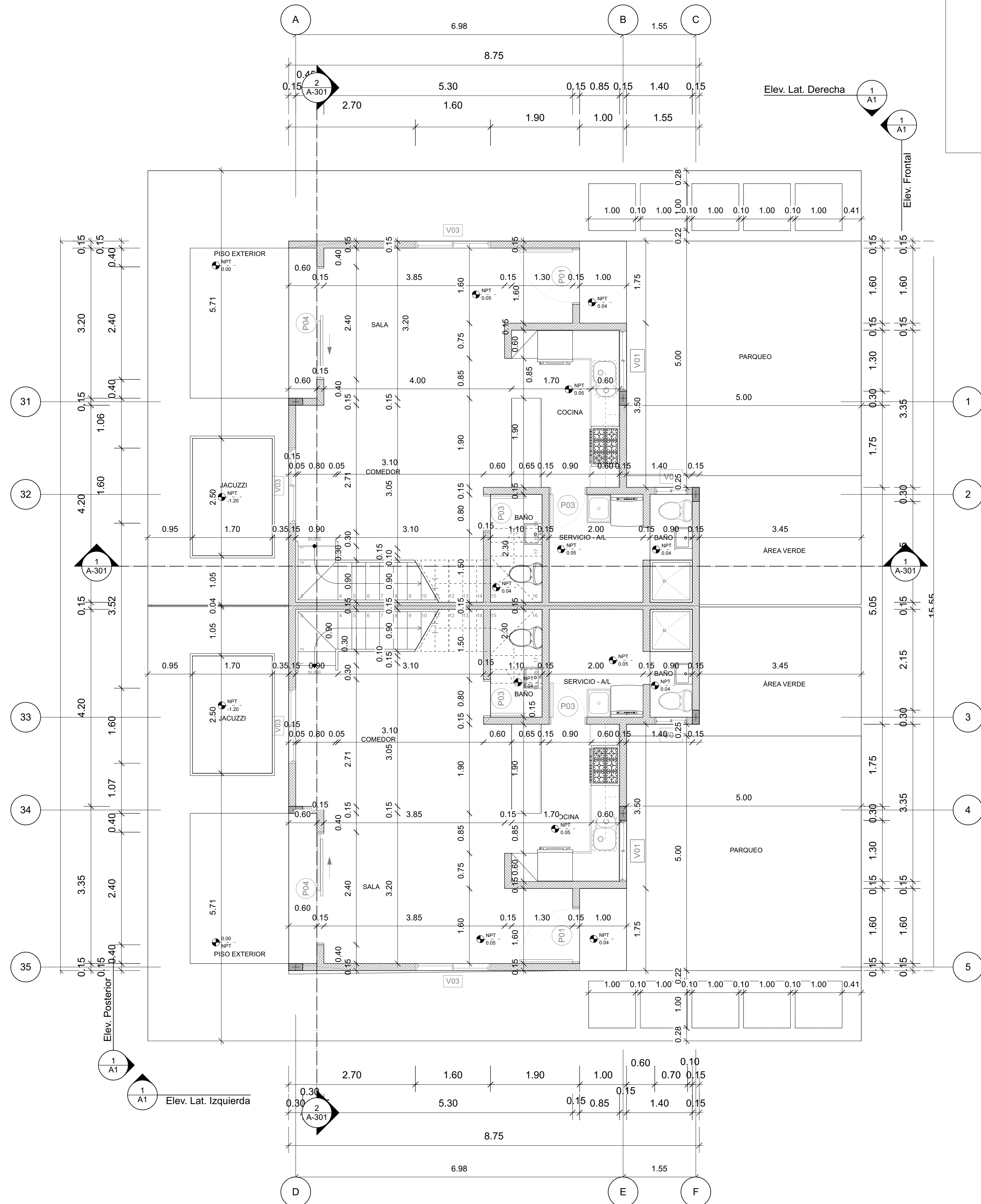
2 Planta Dimensionada - Nivel 1 Scale: 1:50
