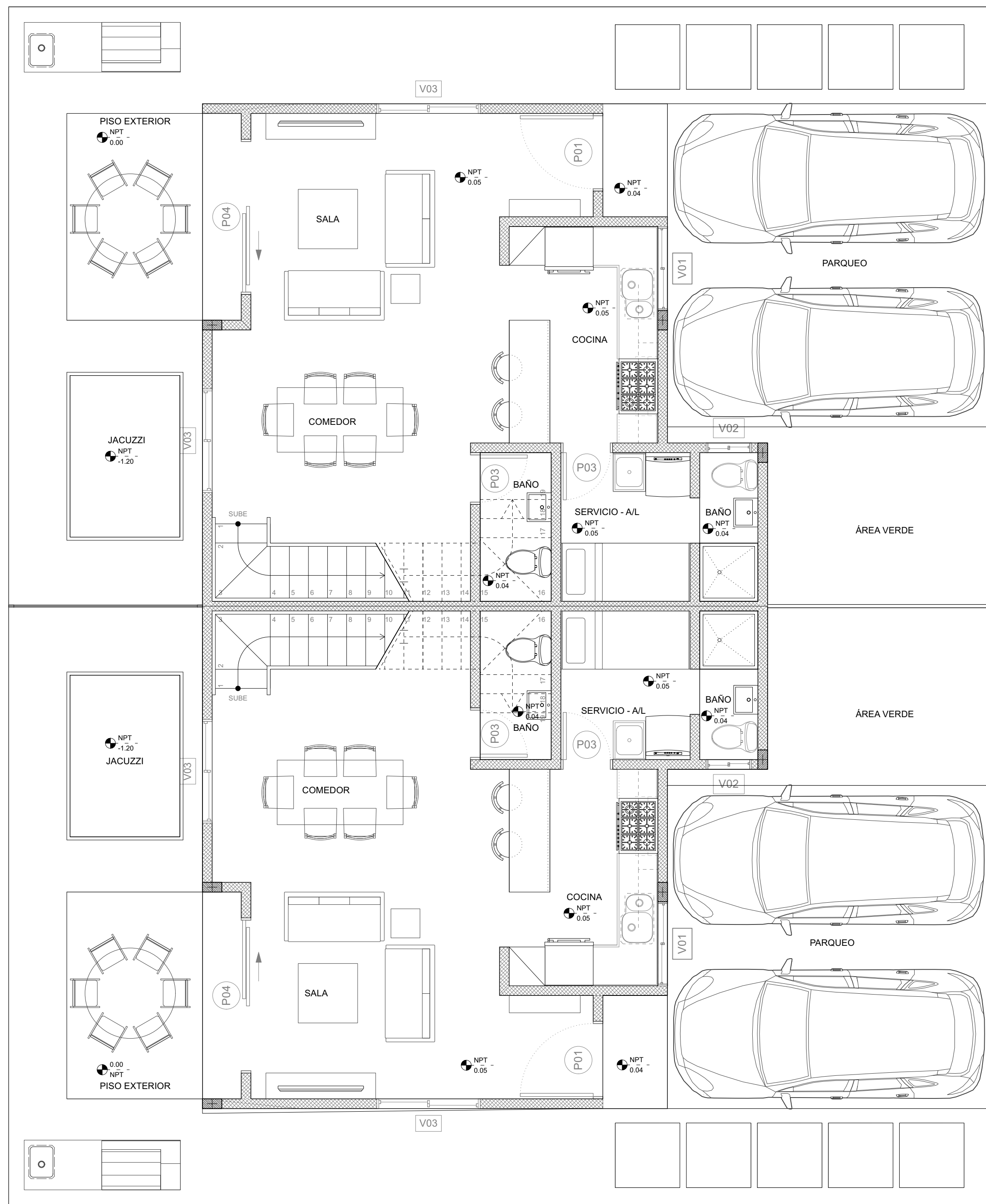
1 Planta Arquitectónica - Nivel 1 Scale: 1:50
