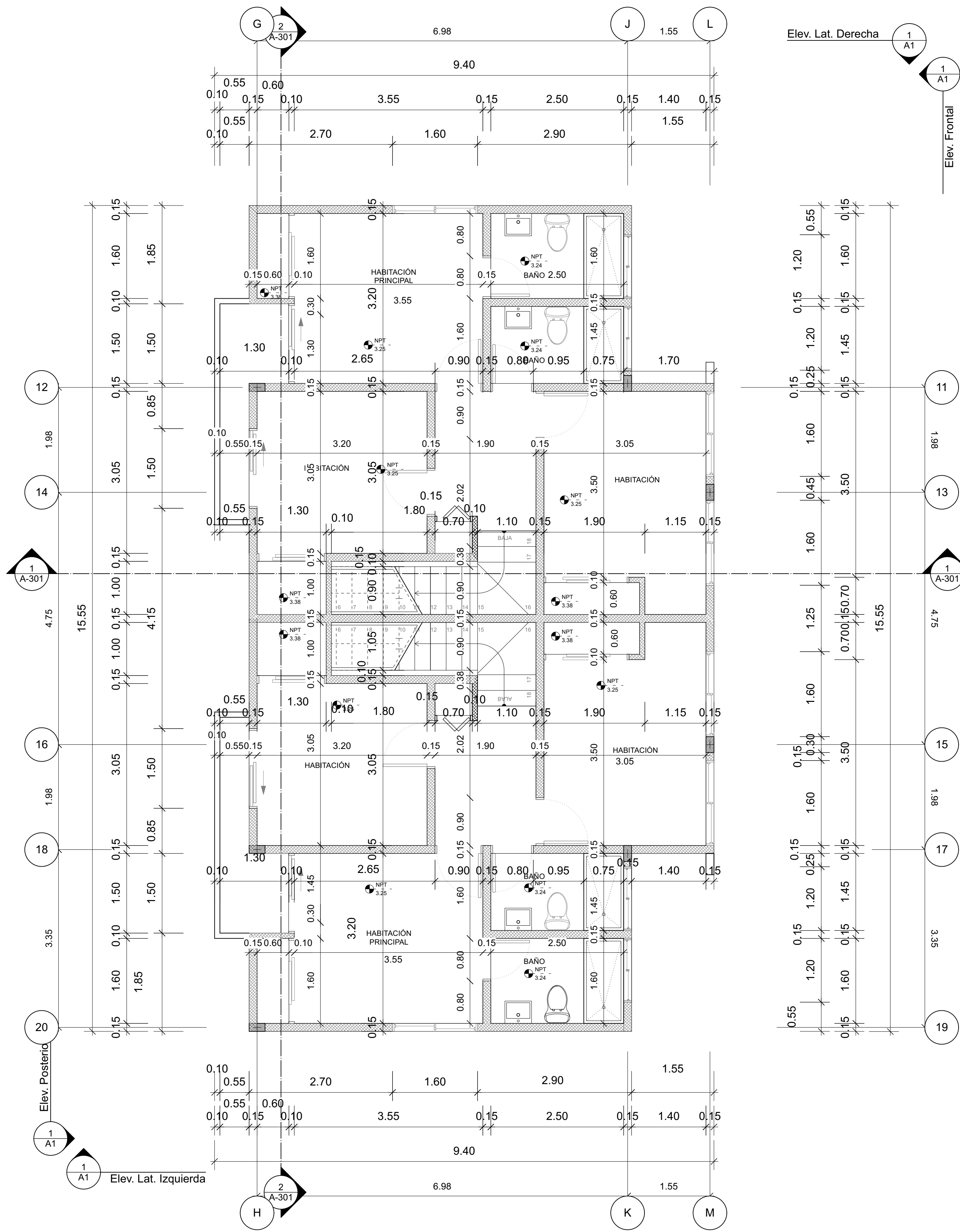
2 Planta Dimensionada - Nivel 2 Scale: 1:50
