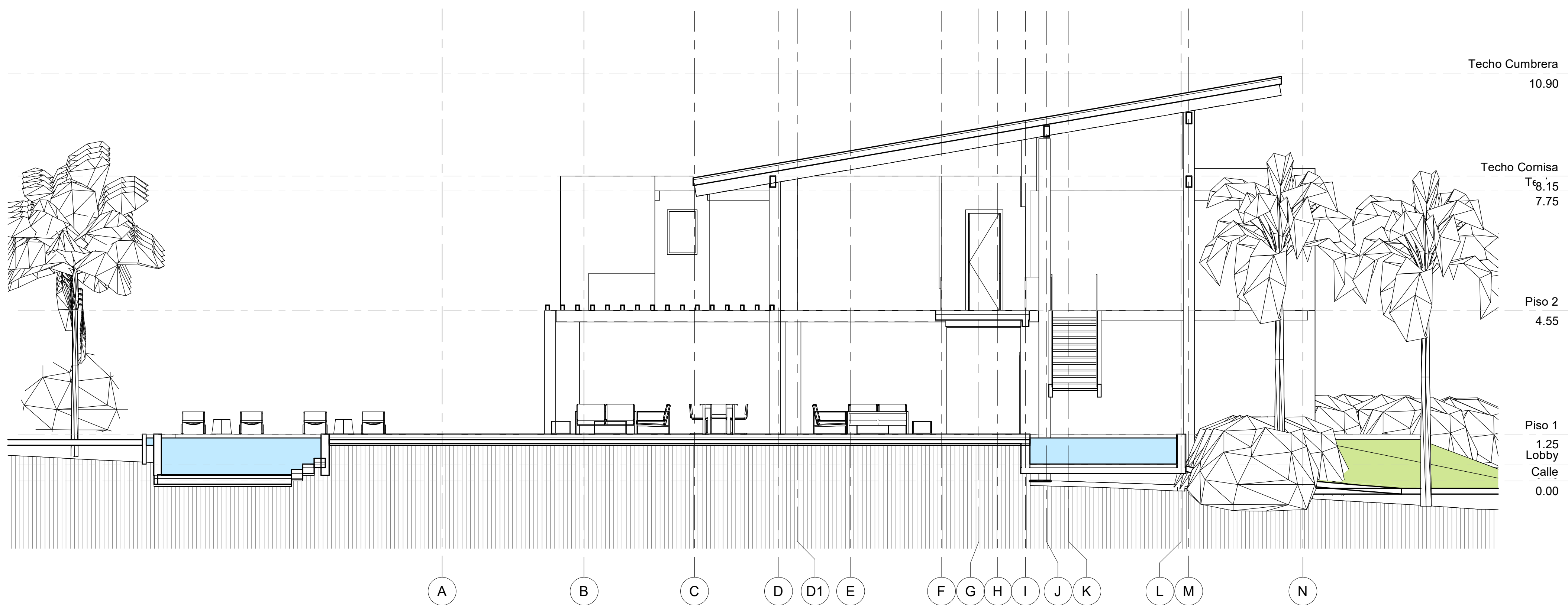
CORTE H
