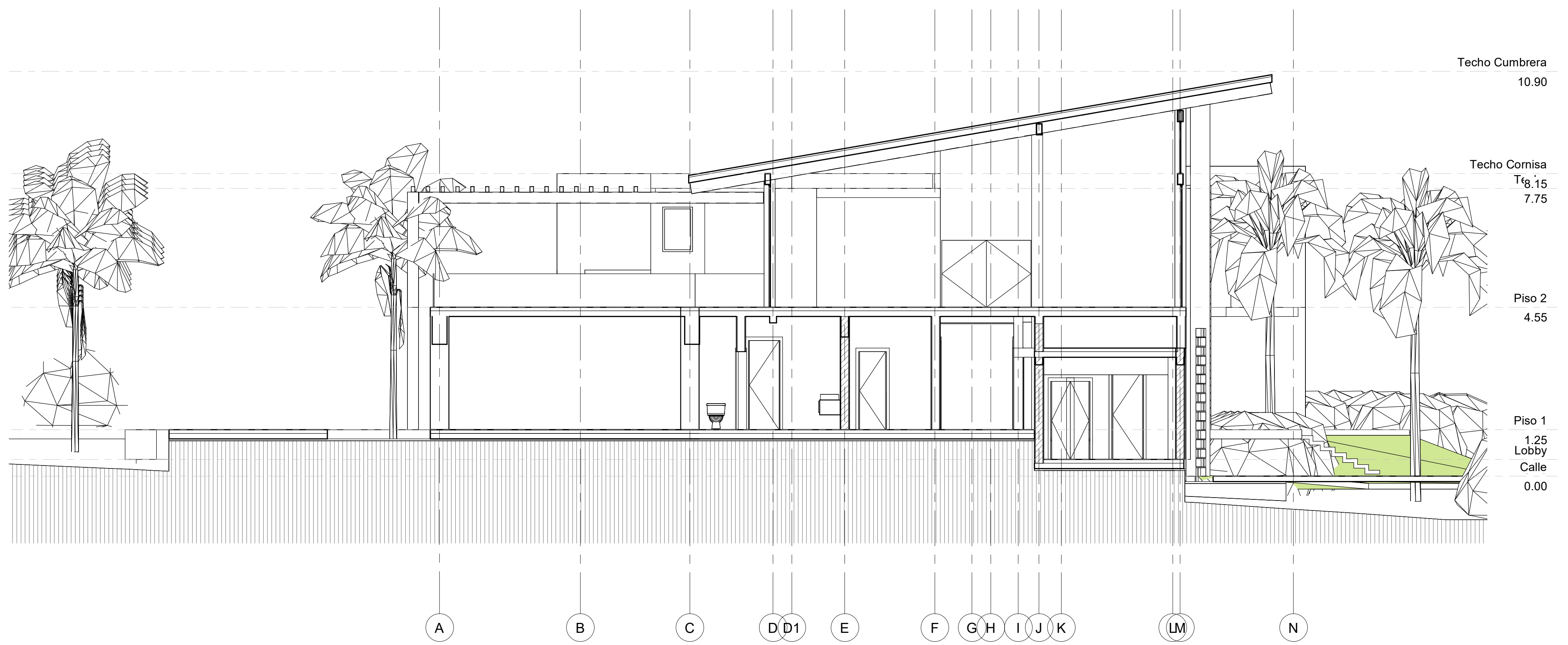
CORTE F
