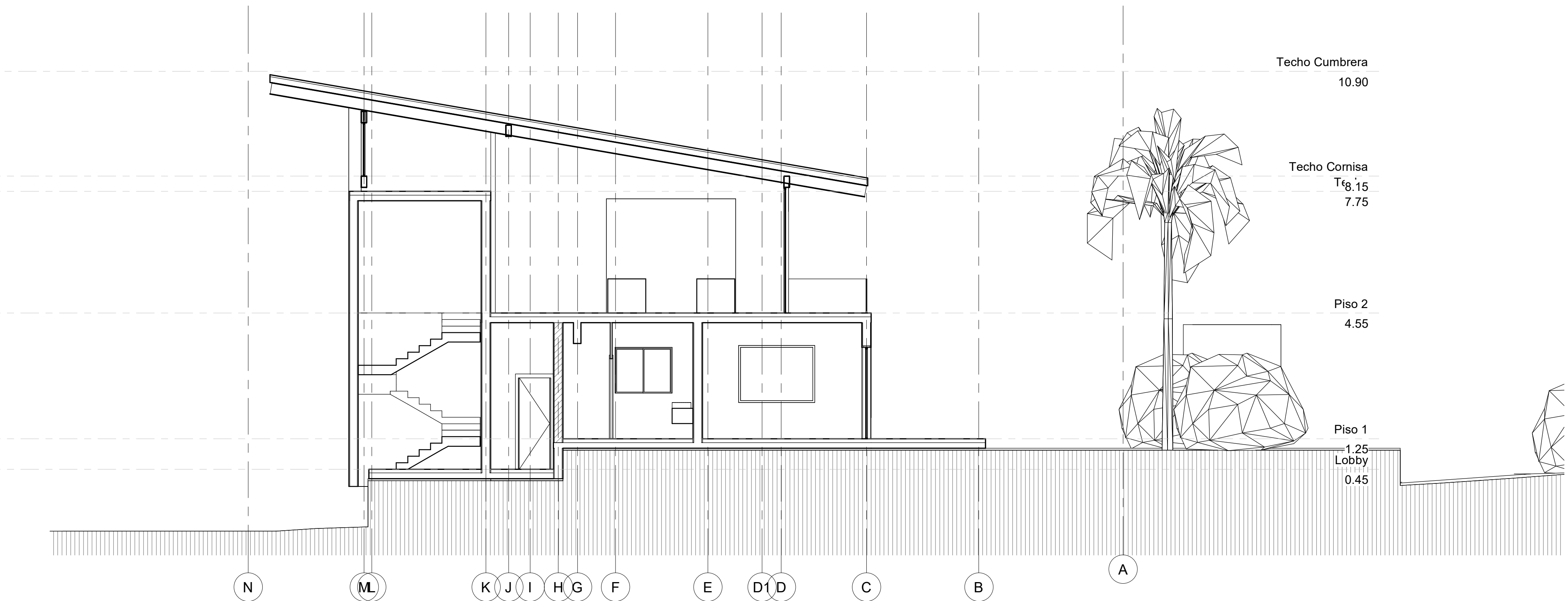
CORTE E
