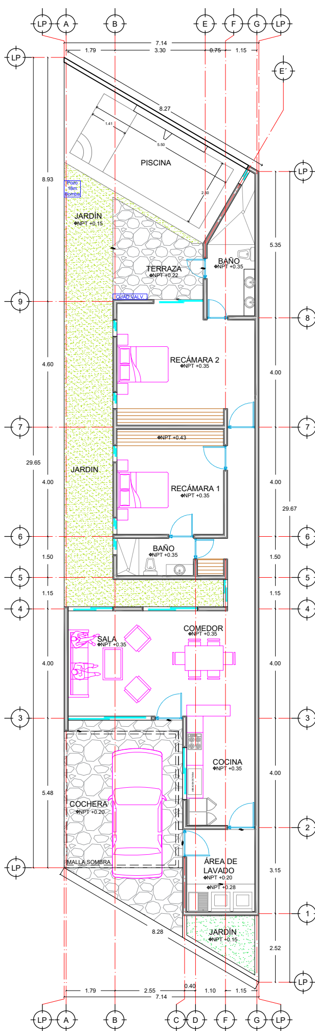
LOTE FC-03 PLANTA ARQUITECTÓNICA
