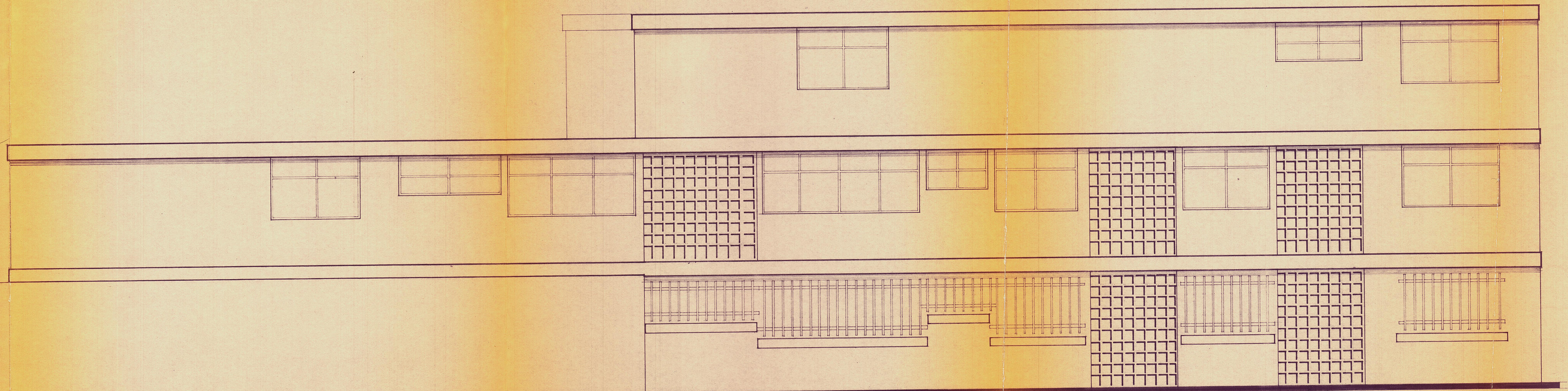
FACHADA POSTERIOR ESC. 1:50
