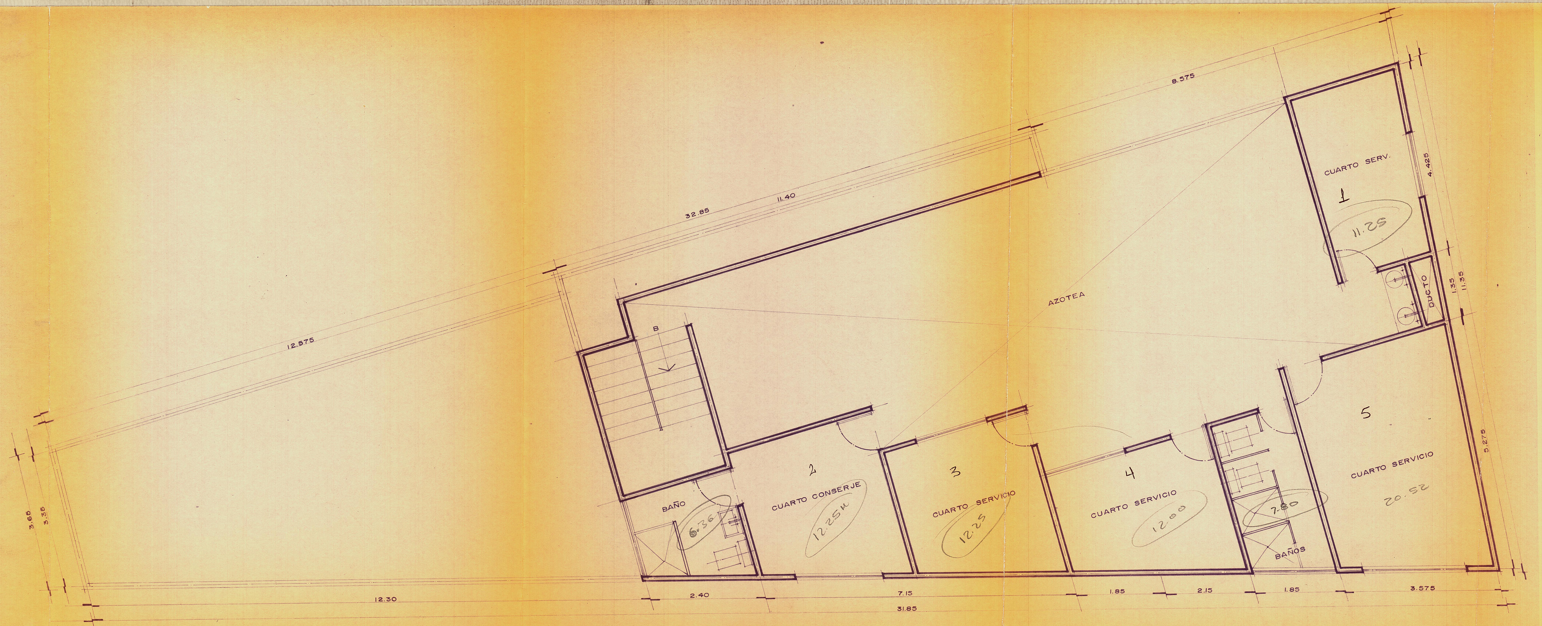
PLANTA NIVEL 3 (SERVICIOS) ESC. 1:50
