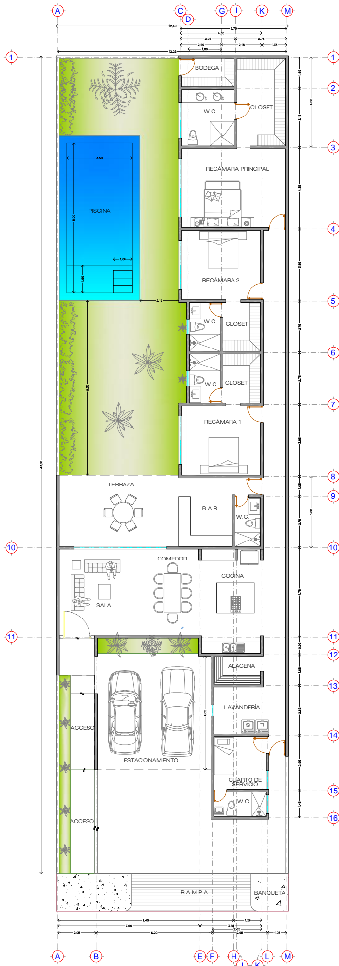
PLANTA ARQUITECTÓNICA
