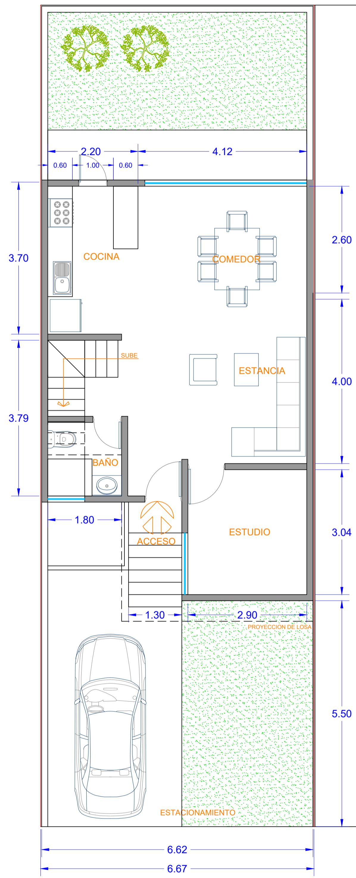
PLANTA BAJA
