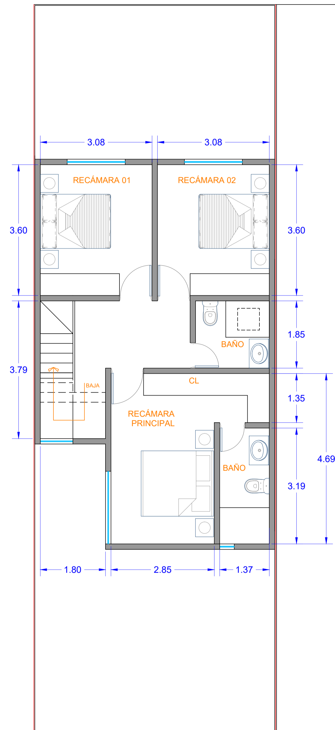
PLANTA ALTA
