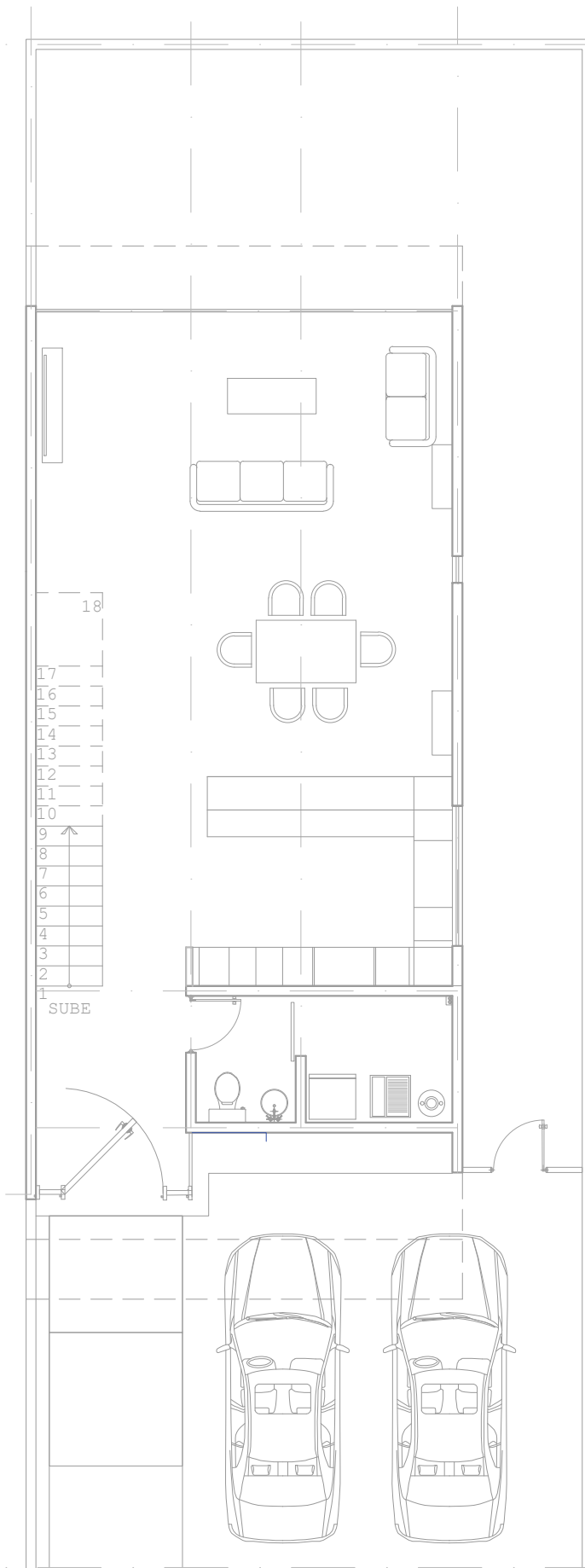
PLANTA BAJA 83.73 m 2
