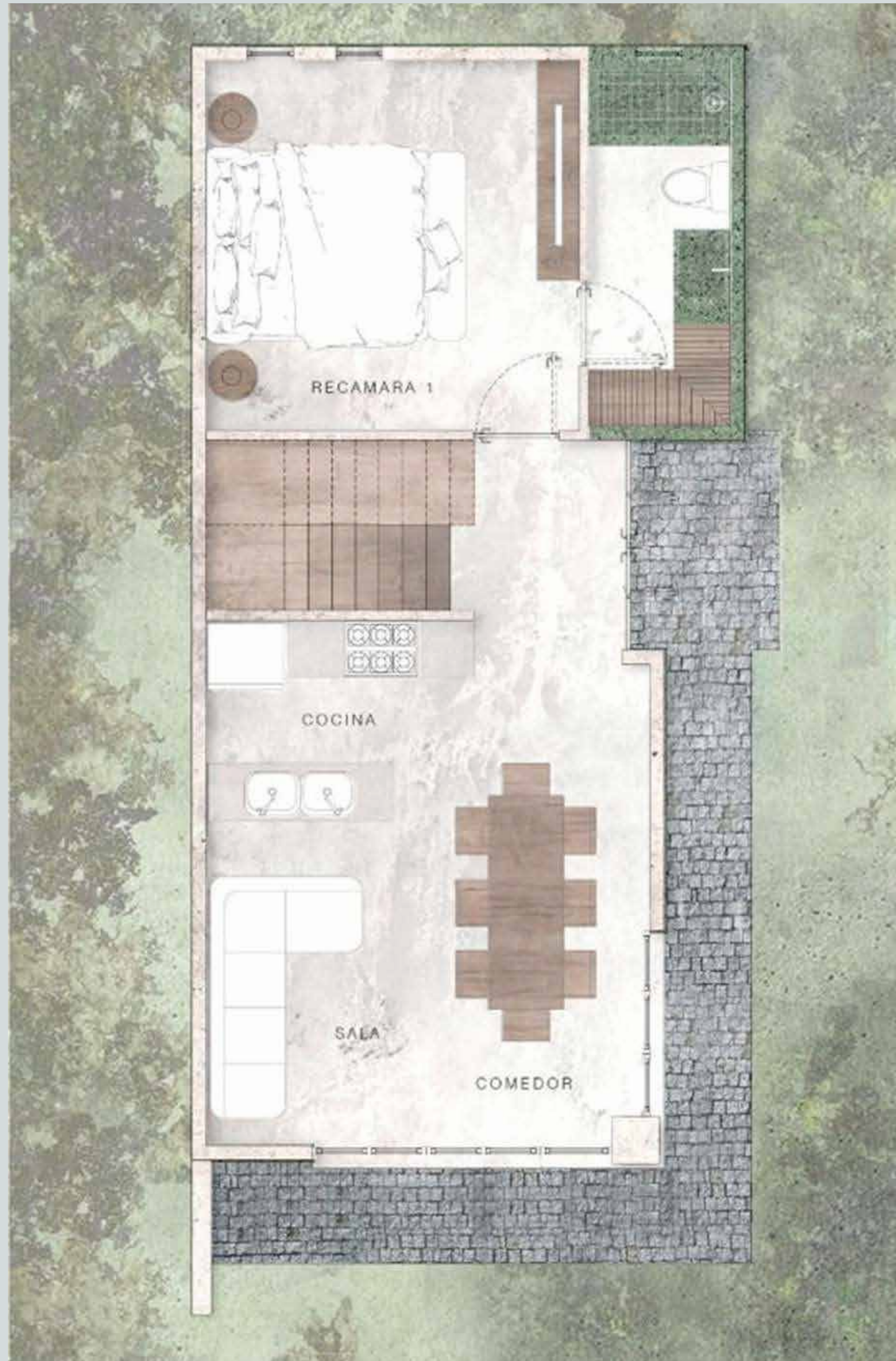
PLANTA BAJA
