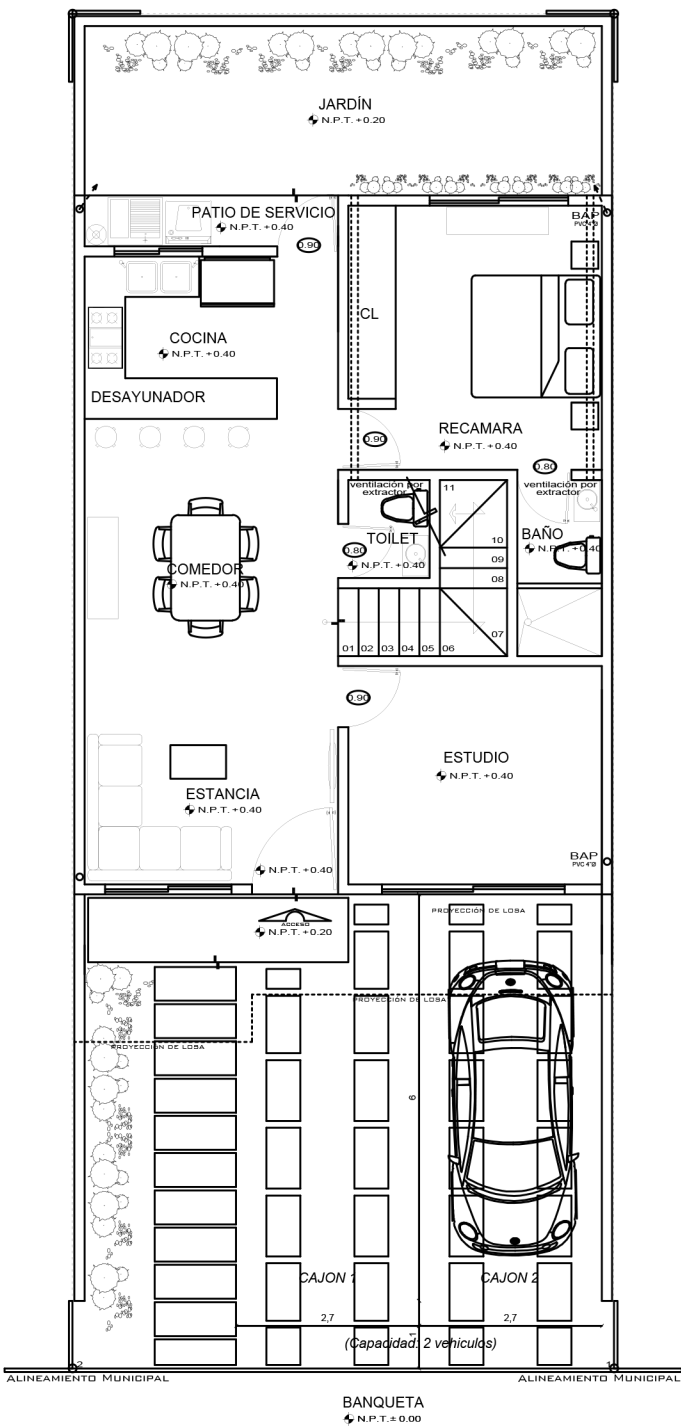
PLANTA ARQUITECTONICA. PLANTA BAJA. ESCALA 1 : 50
