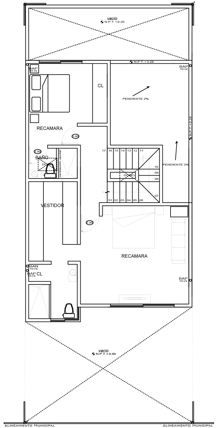
PLANTA ARQUITECTONICA. PLANTA ALTA. ESCALA 1 : 50
