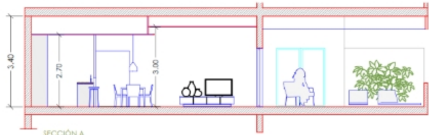
SECCIÓN A
