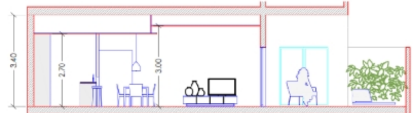
SECCIÓN A
