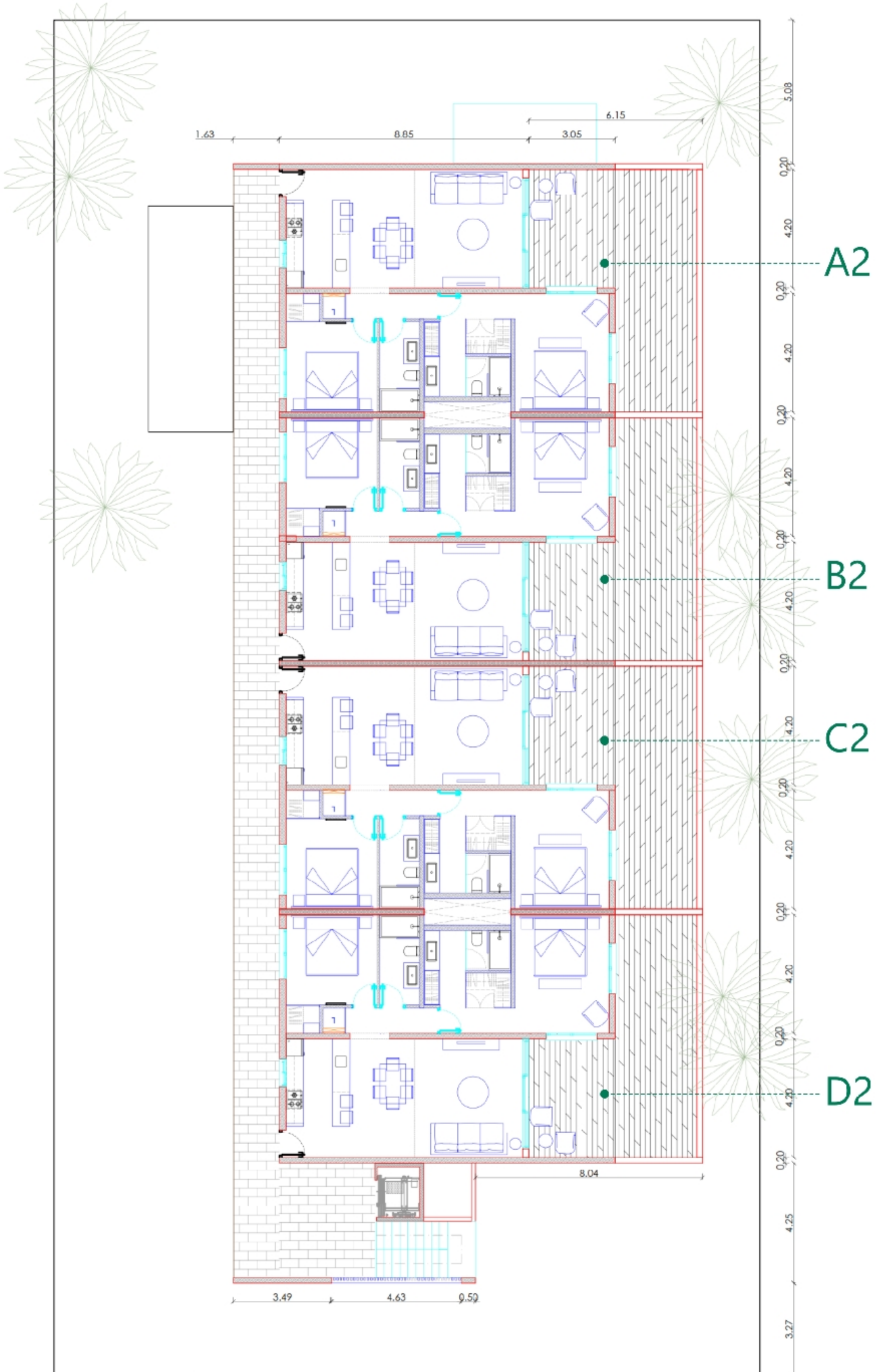
PLANTA 2DO NIVEL
