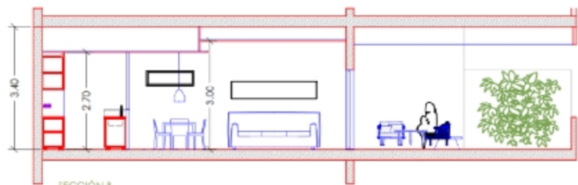
SECCIÓN B
