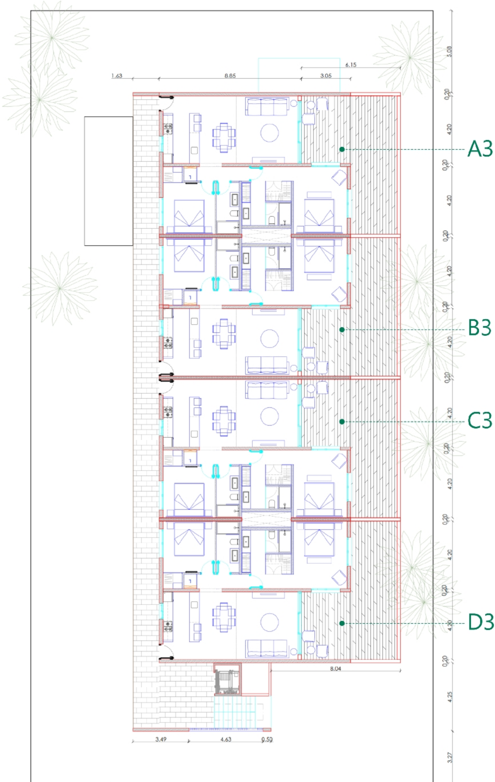
PLANTA 3ER NIVEL
