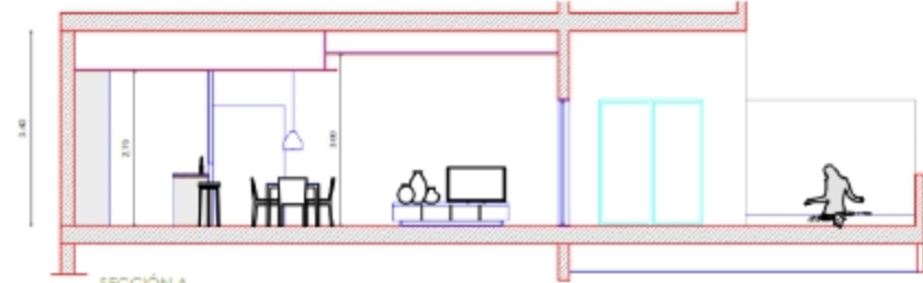
SECCIÓN A
