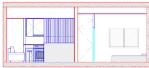
SECCIÓN E
