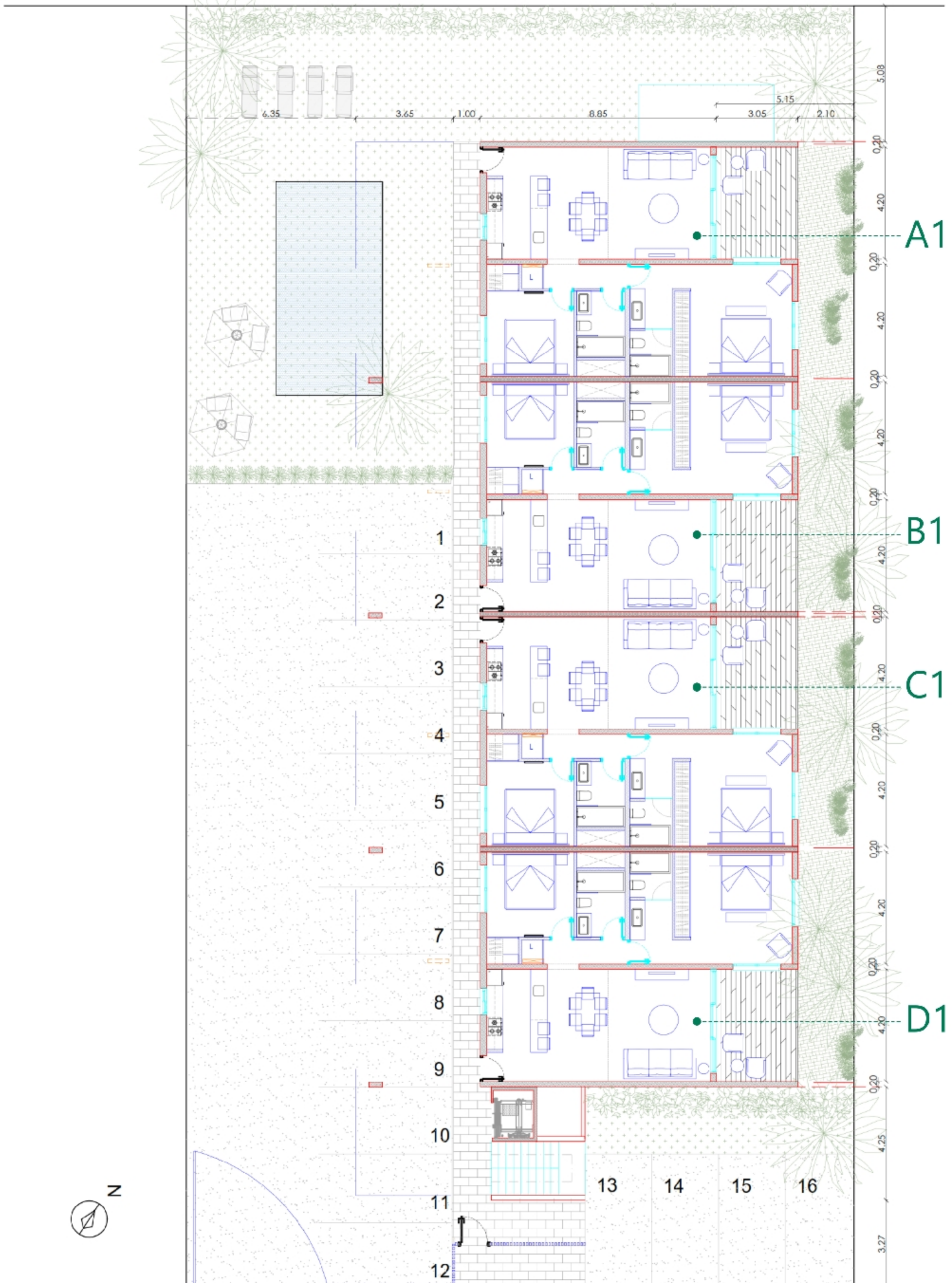
PLANTA 1ER NIVEL
