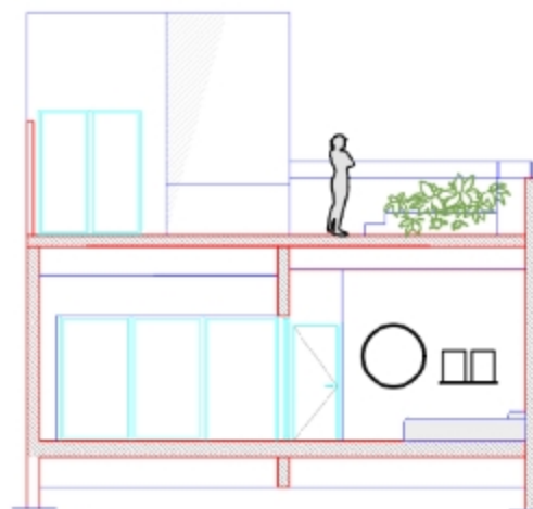
SECCIÓN D
