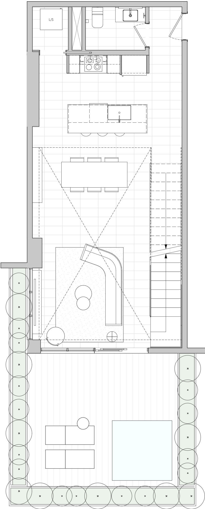
PLANTA ARQUITECTONICA NIVEL 1
