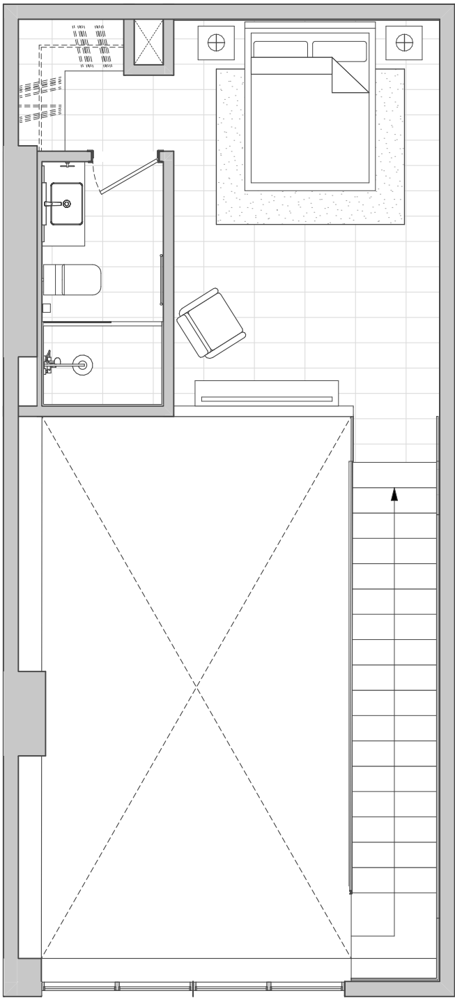
PLANTA ARQUITECTONICA NIVEL 2
