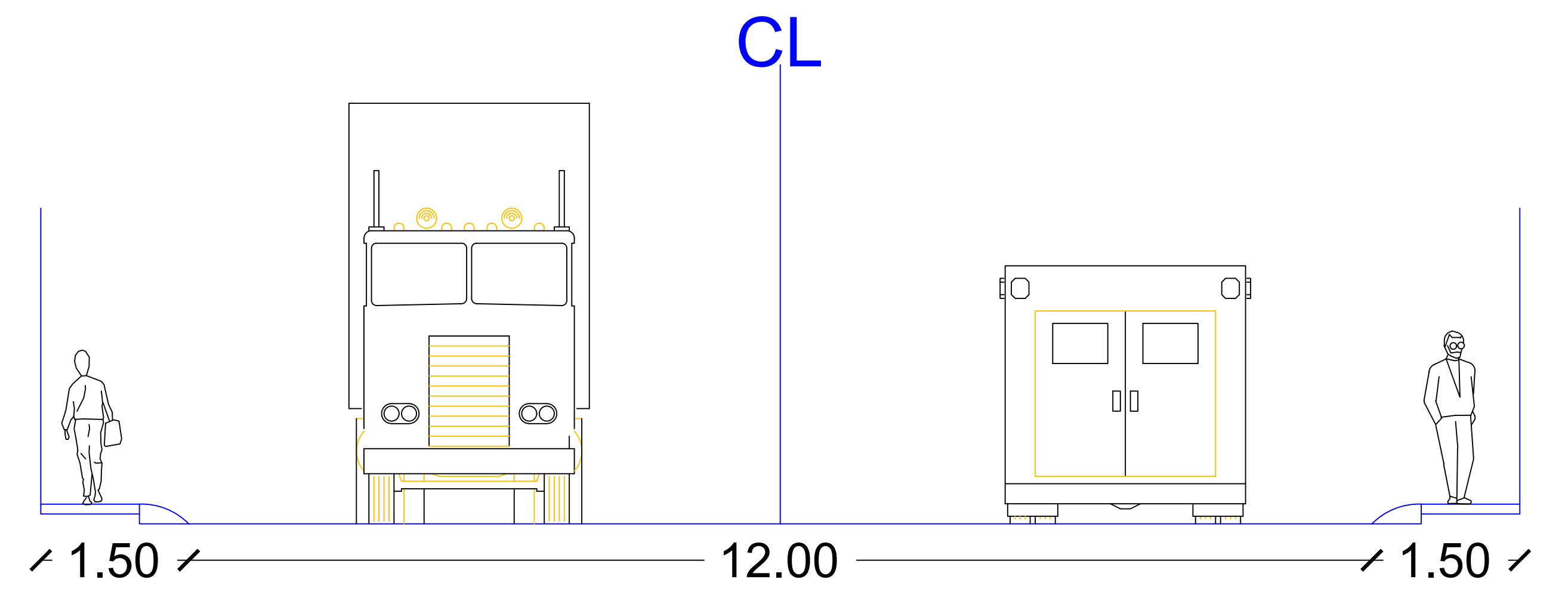
CORTE A-A'
