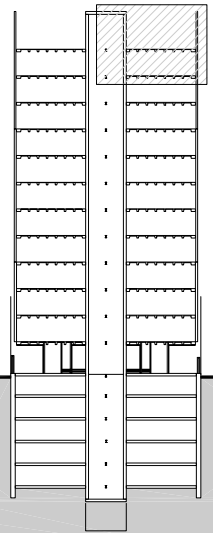
CORTE ESQUEMATICO
