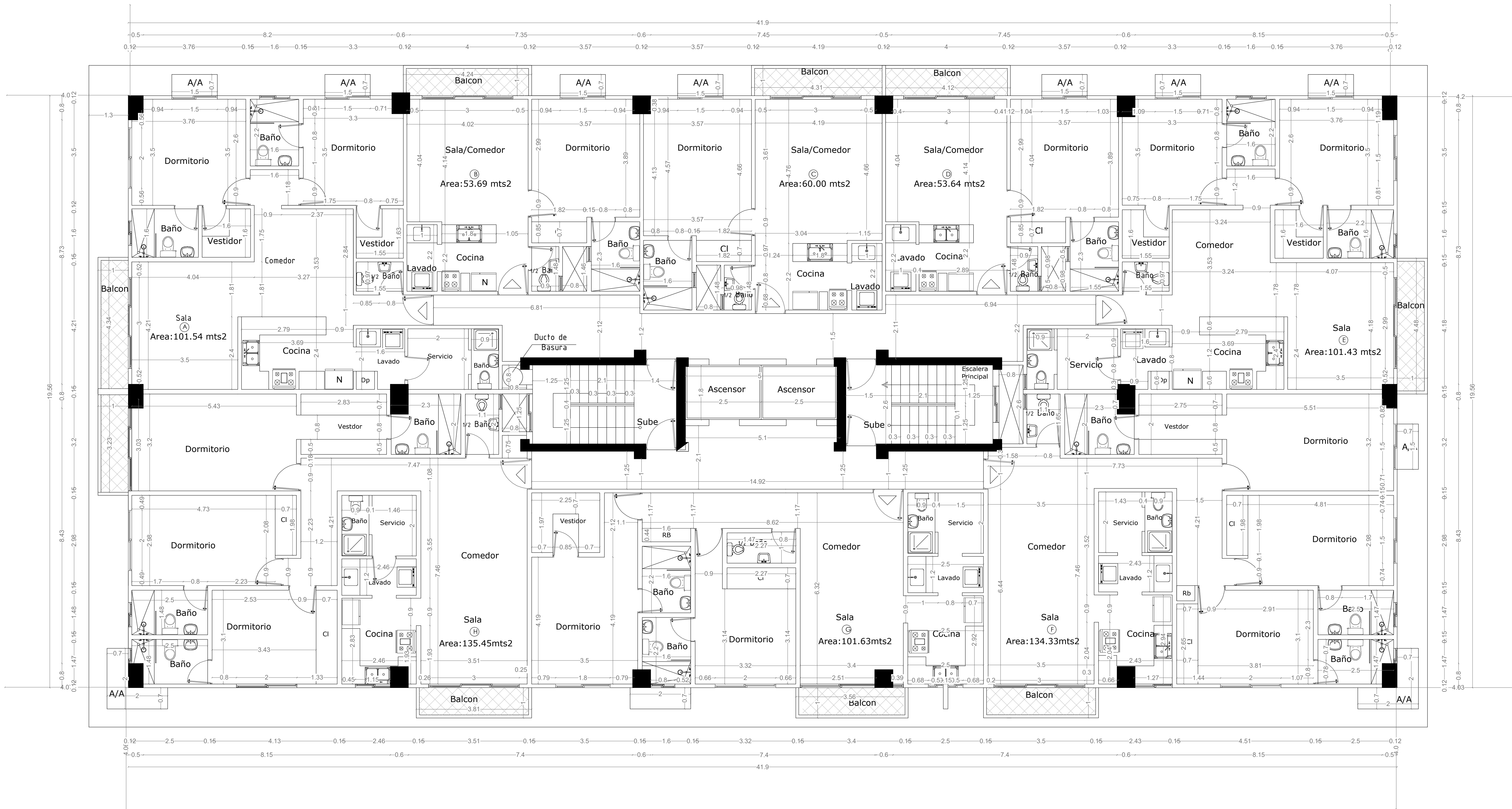
PLANTA ARQ. DIMENSIONADA 2DO. NIVEL TORRE CARMEN OFELIA III ESC.: 1:60
