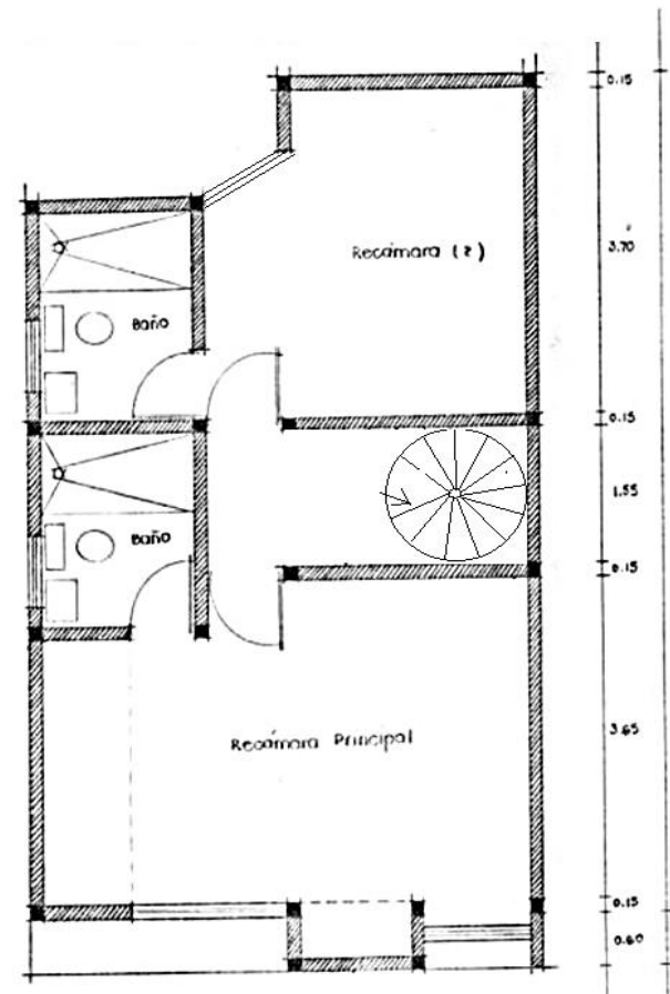
Plano Arquitectónica (Alta) ESCALA: 1:50
