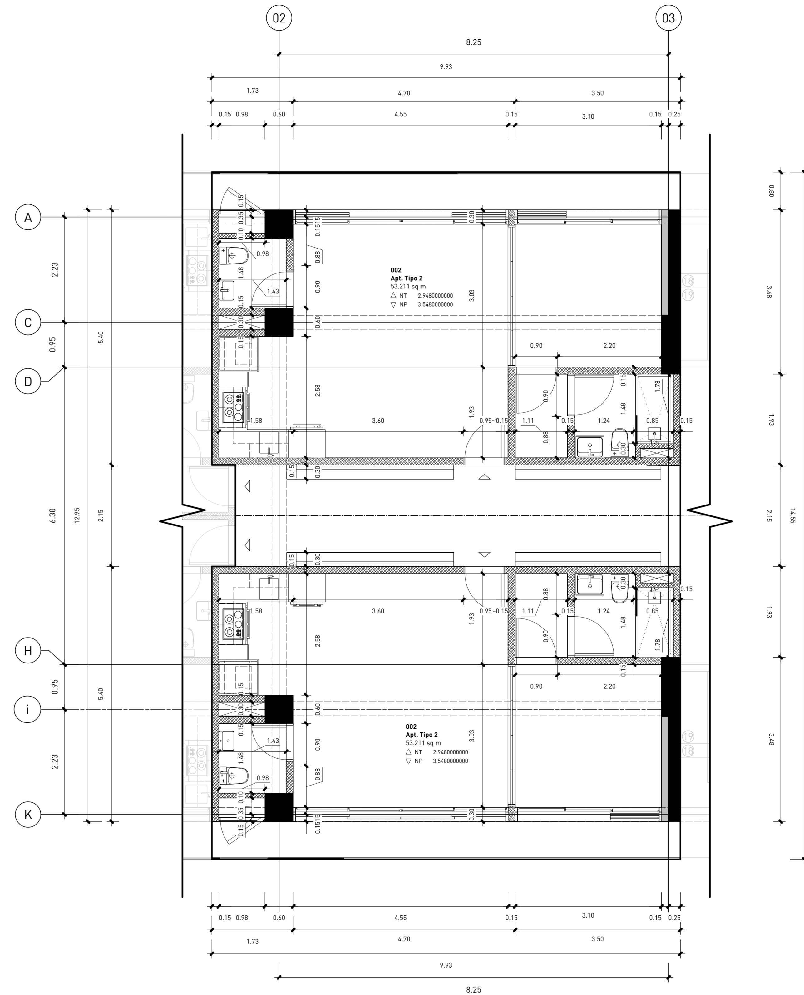
2 Planta Arquitectónica Dimensionada Apts. B-F/C-H Niveles 2-6 A4 22 1:50
