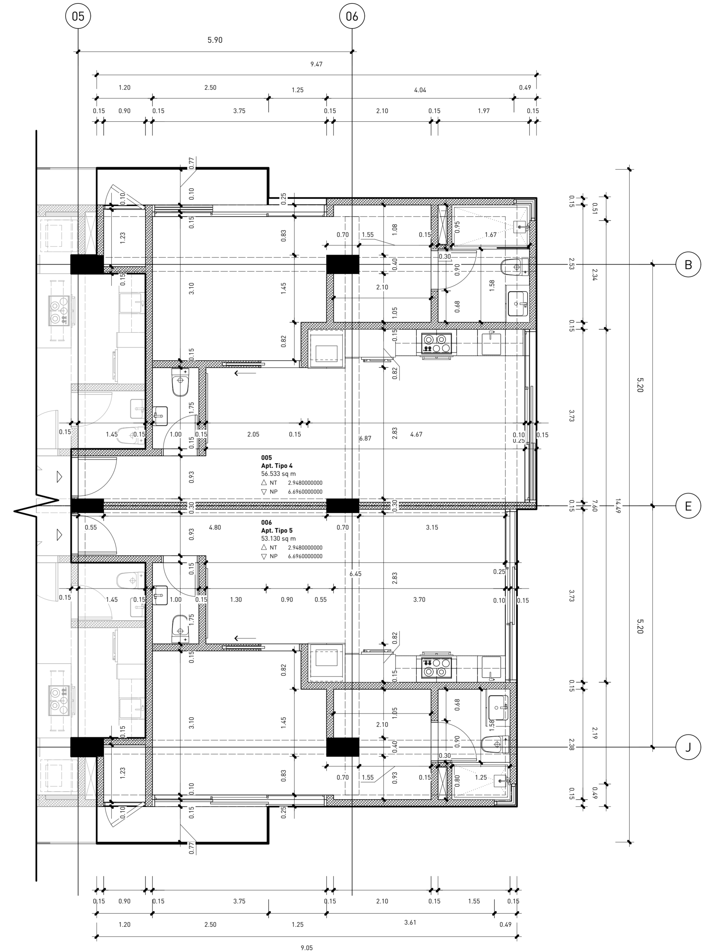
2 A4 15 Planta Arquitectónica Dimensionada Apts. E-F Nivel 3 1:50
