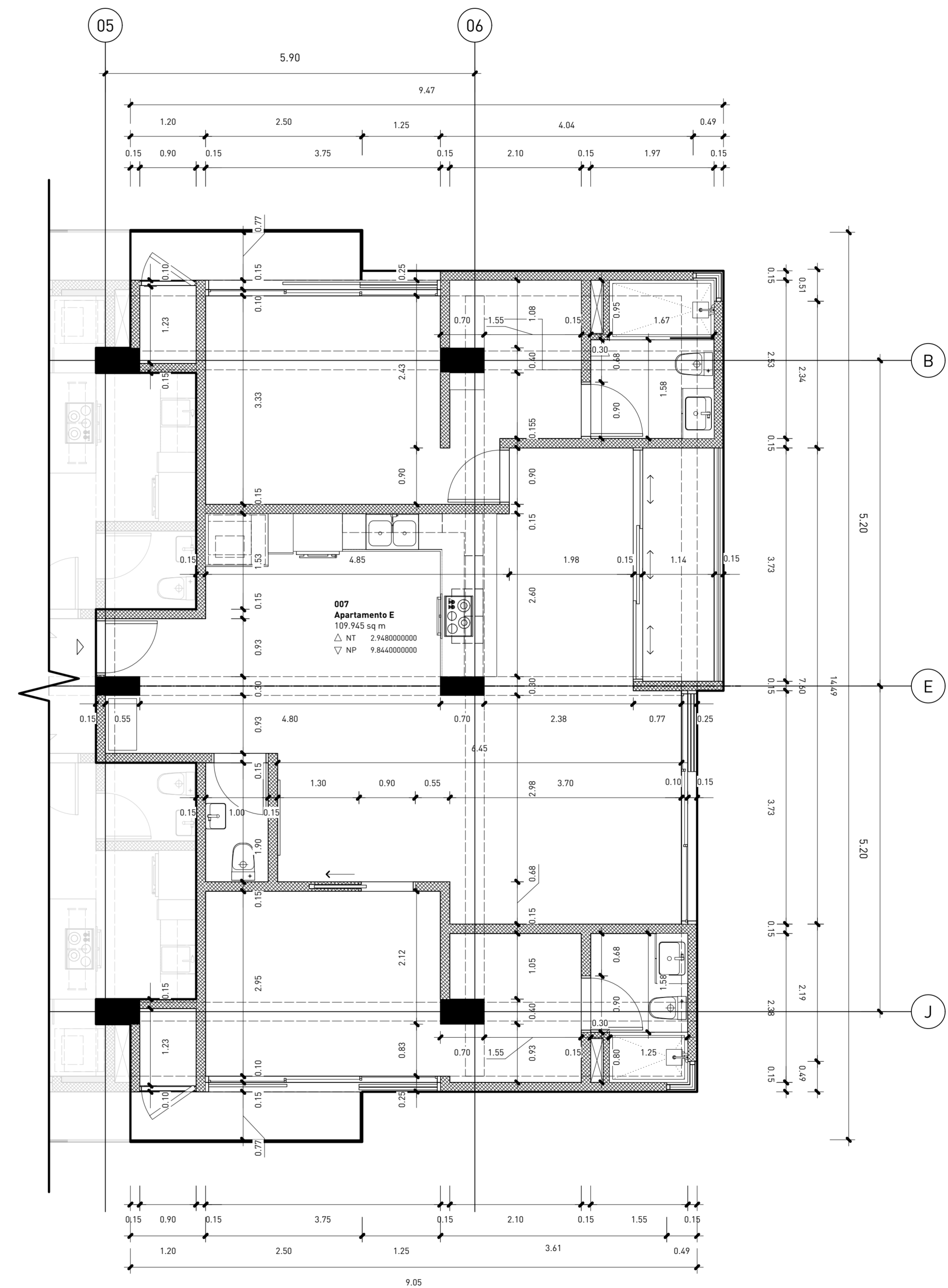
2 A4 18 Planta Arquitectónica Dimensionada Apt. E Niveles 2-6 1:50
