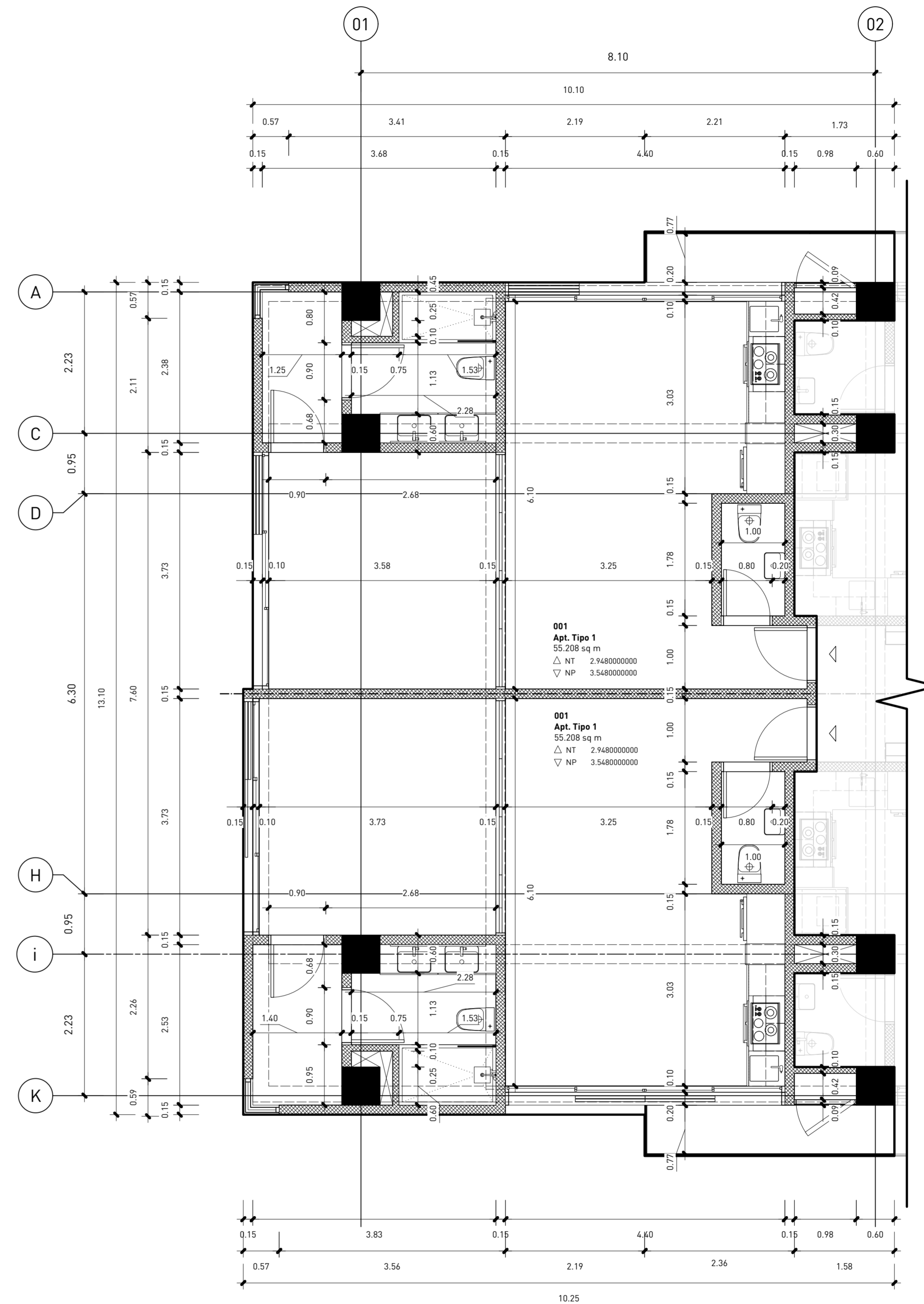
2 Planta Arquitectónica Dimensionada Apts. A-B Niveles 2-6 A4 23 1:50
