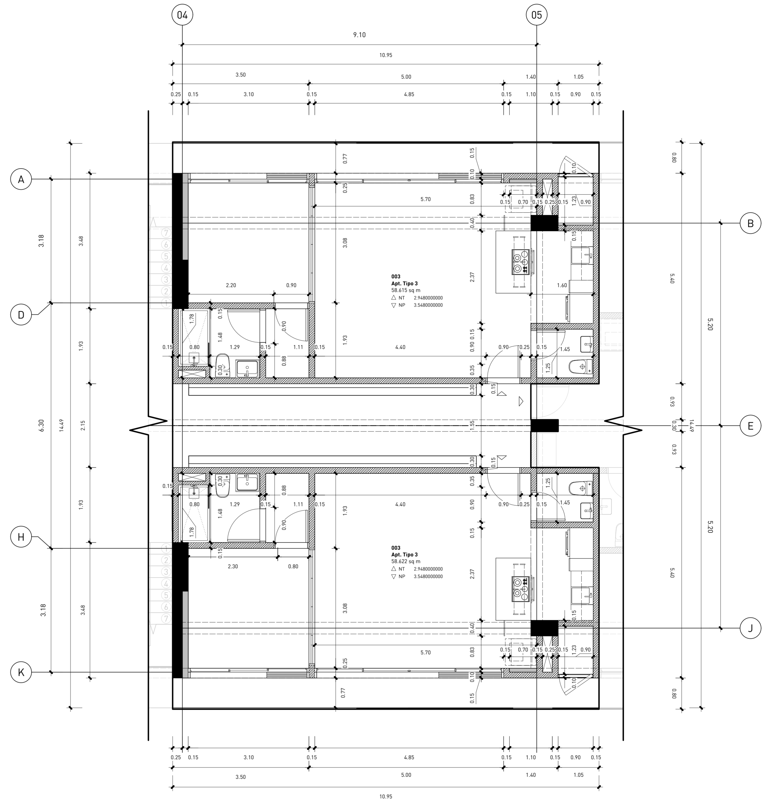
2 A4 21 Planta Arquitectónica Dimensionada Apts. C-E/G-D Niveles 2-6 1:50
