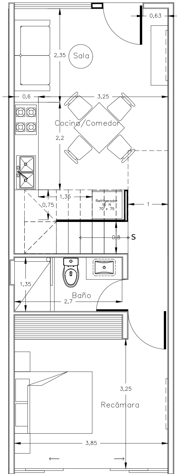
TIPO C 69.60 M2 PLANTA BAJA
