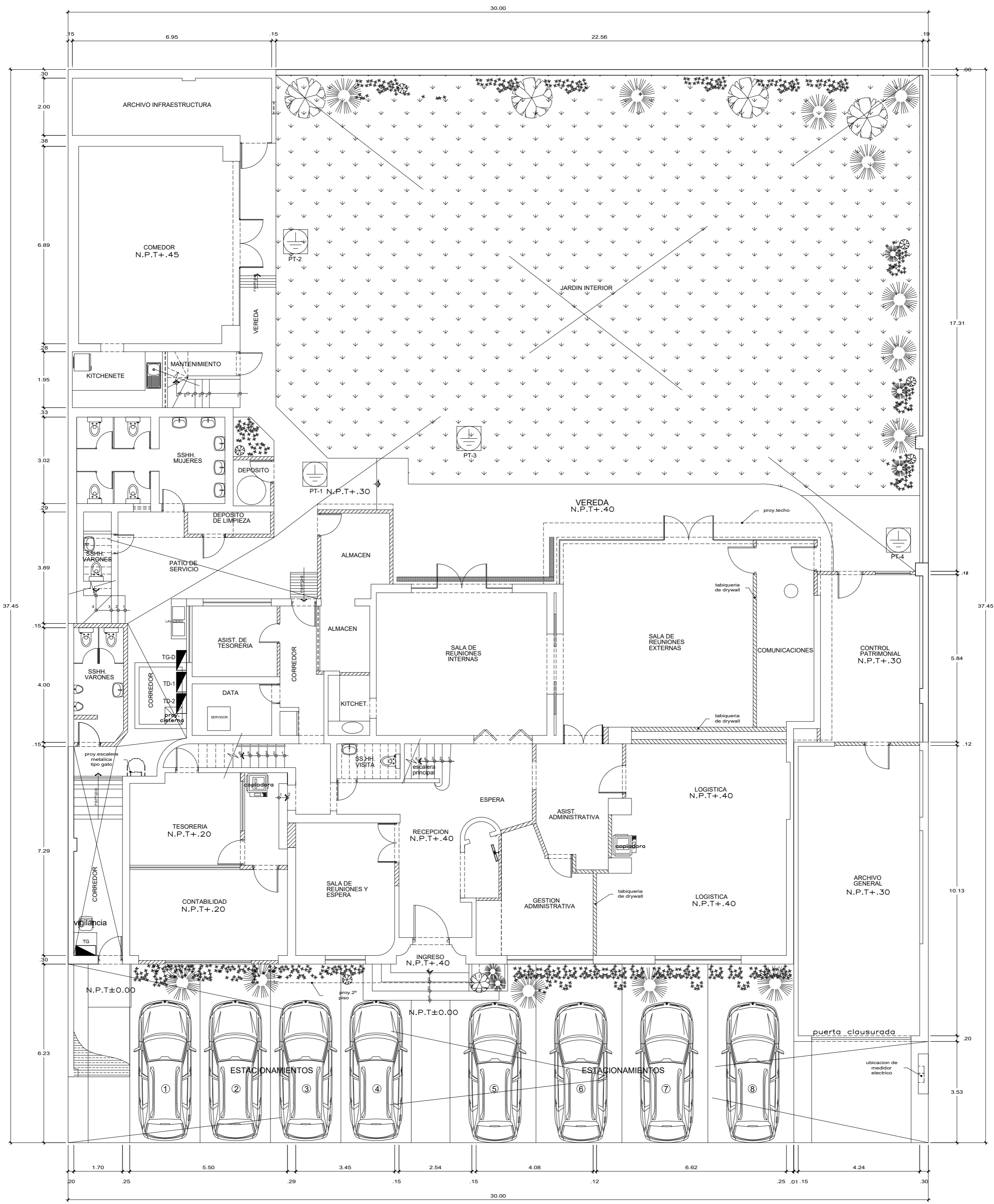
1º PISO-UBICACION DE TABLEROS ELECTRICOS ESCALA : 1/100
