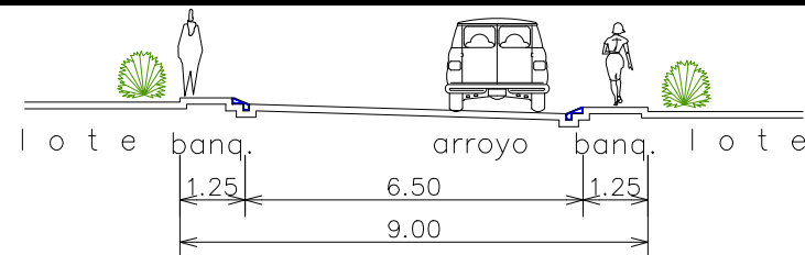
SECCIÓN DE CALLE PRIVADA
