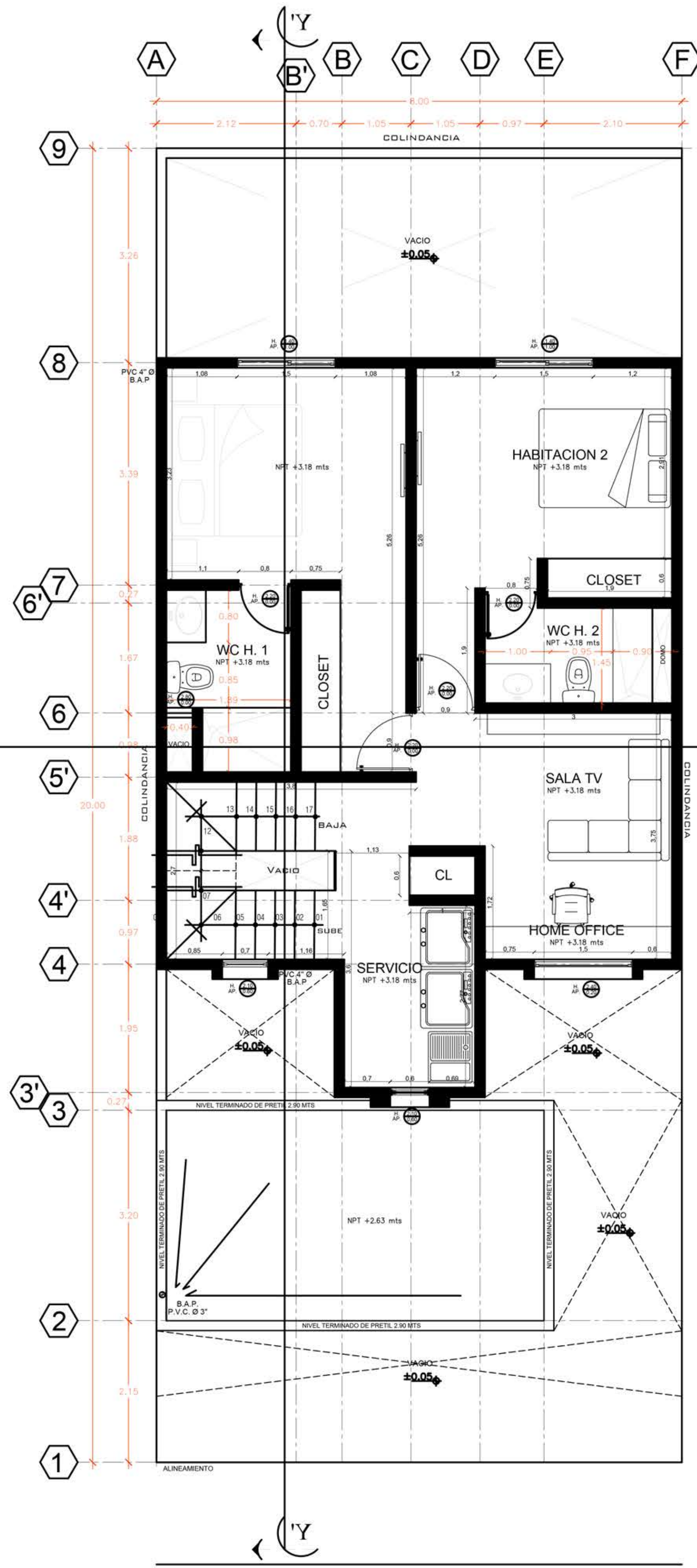
PLANTA ALTA
