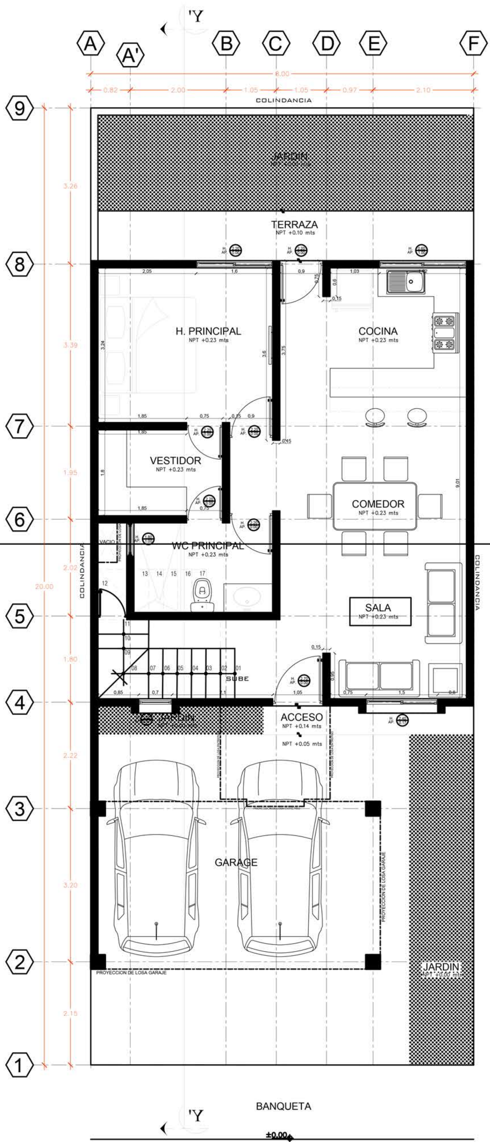
PLANTA BAJA
