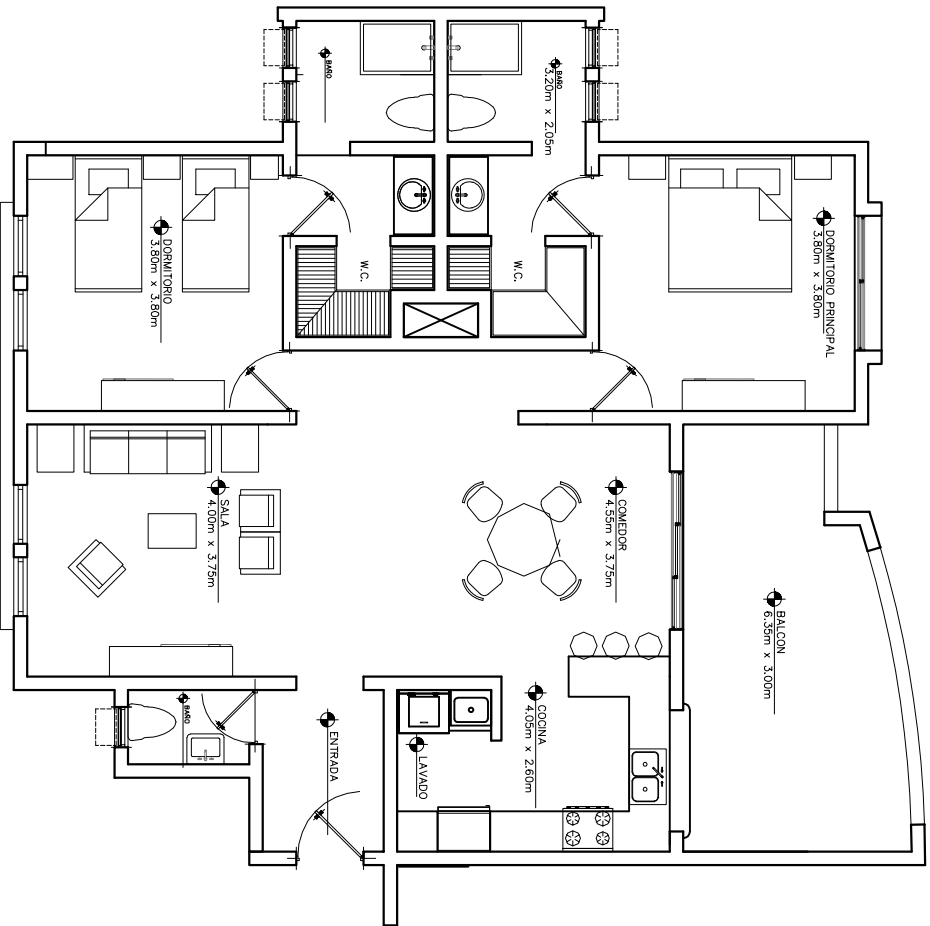
APARTAMENTOS DE 2 HABITACIONES Y 2,5 BAÑOS AREA INTERIOR = 142.00 m2
