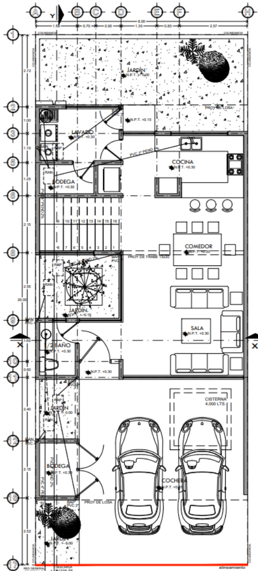
01 PLANTA BAJA 108.00 M 2
