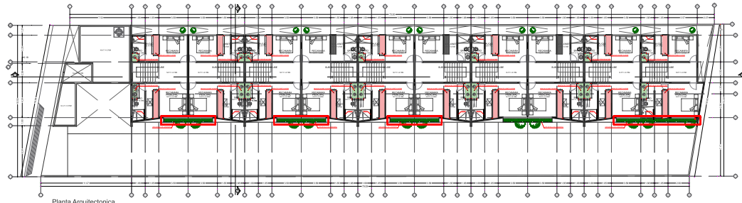
Planta Arquitectonica ALTA
