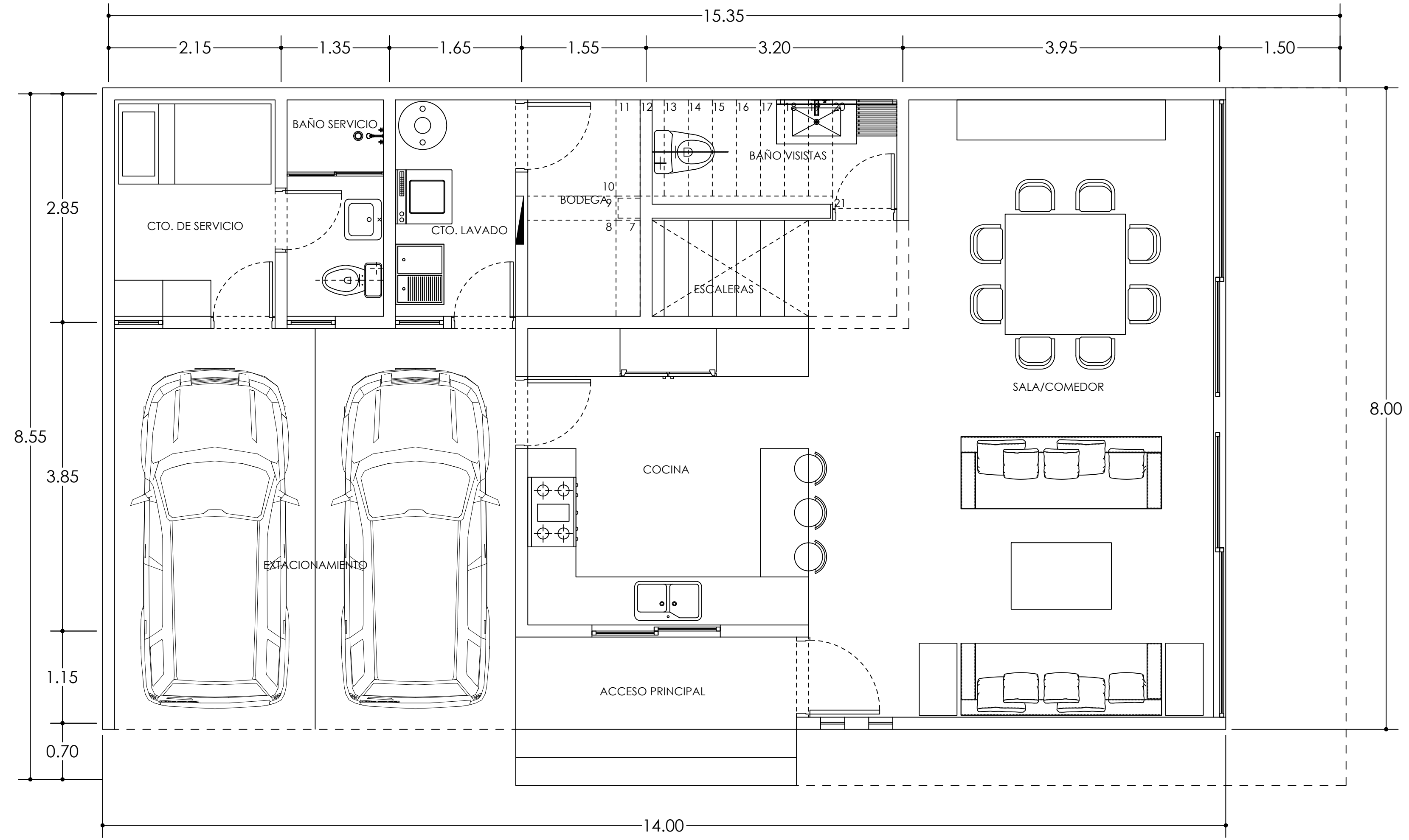
TRIPLOGIA CASA B PLANTA BAJA
