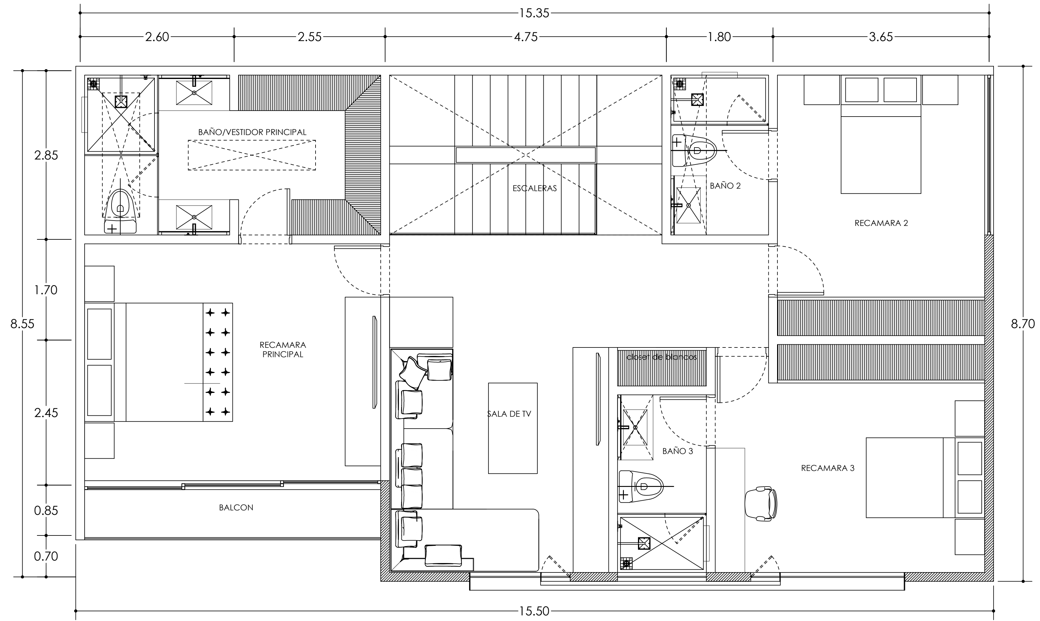
TIPOLOGIA CASA B PLANTA ALTA
