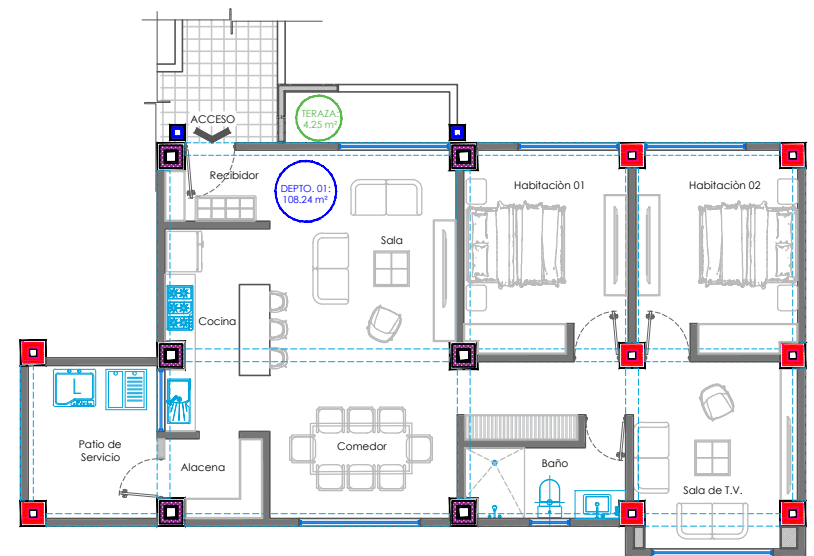
02 ARQUITECTÓNICO - PLANTA TIPO TORRE MASTRETTA Departamento Tipo 112.49 m 2
