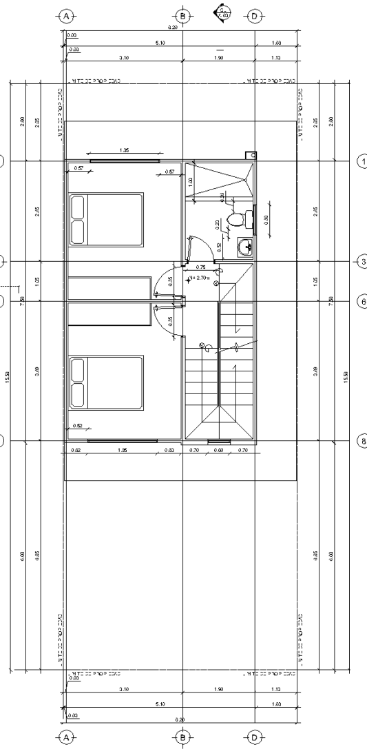
PLANTA SEGUNDO NIVEL
