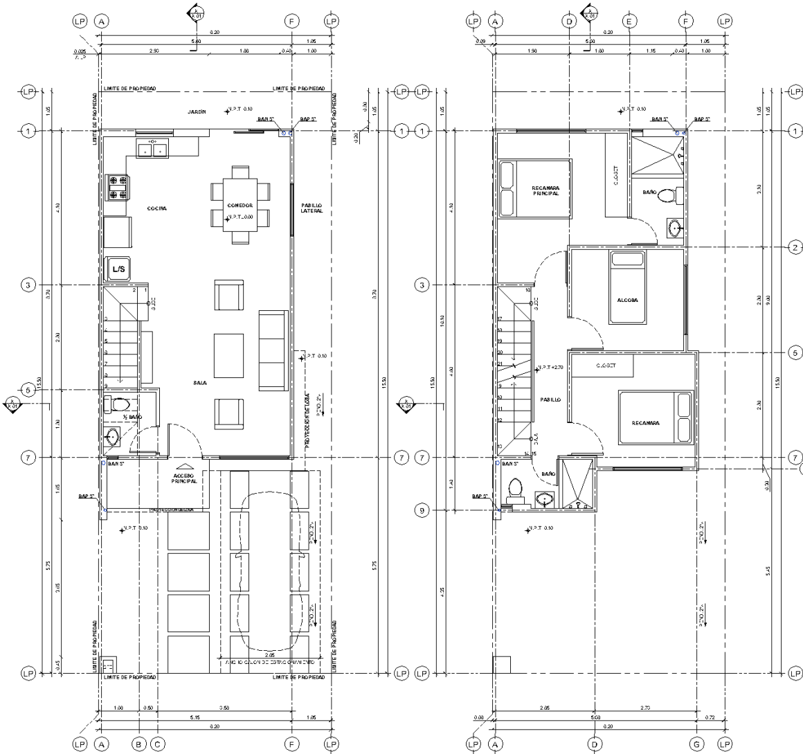
PLANTA PRIMER NIVEL
