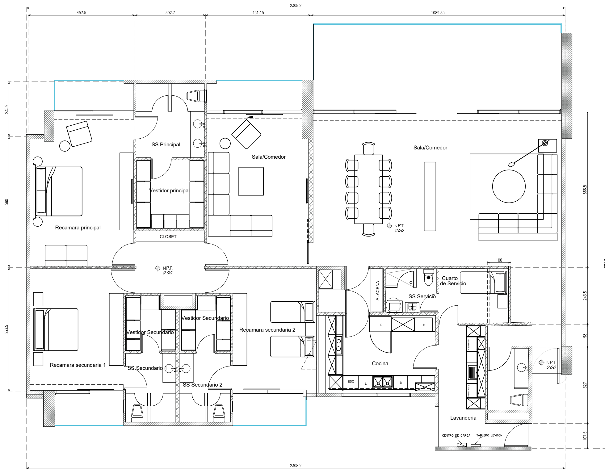
PLANTA ARQUITECTONICA AREA DPTO. 703: 353.83M2
