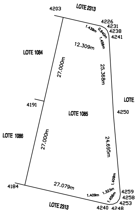
CUADRO DE CONSTRUCCION LOTE 1085
