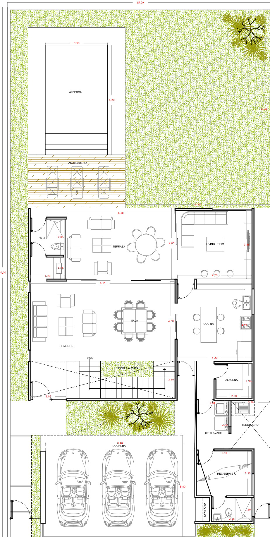
PLANTA ARQUITECTONICA PRIMER NIVEL 207.00 M2
