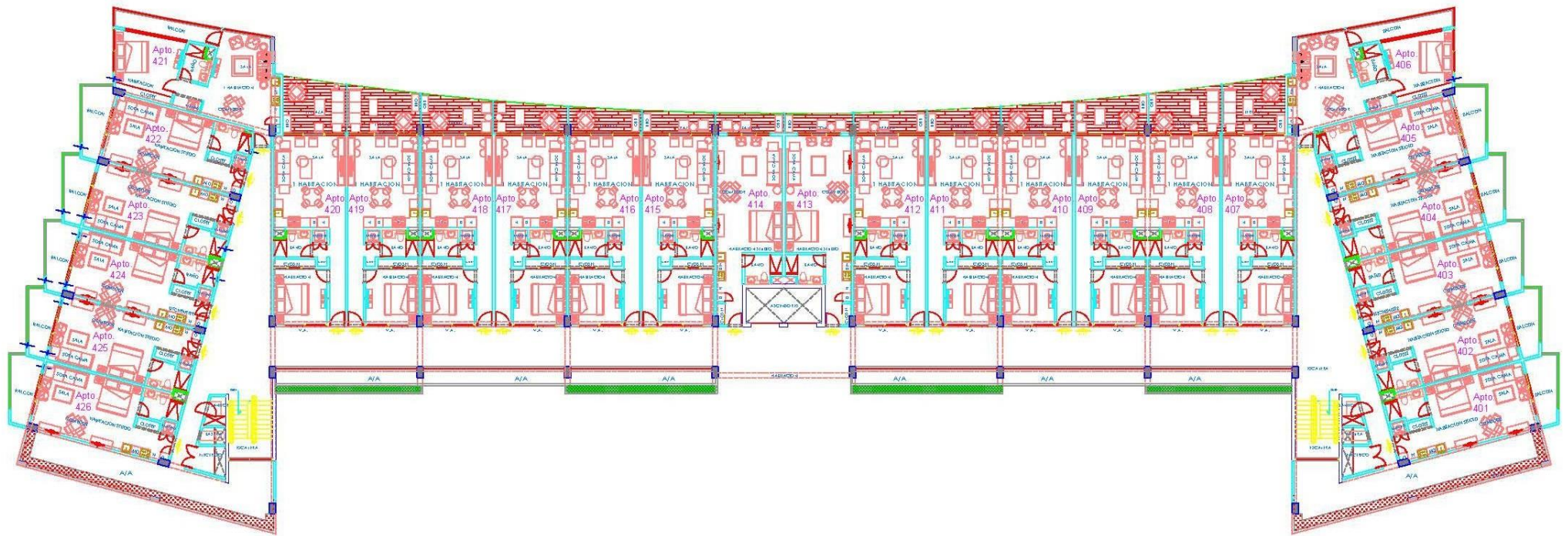
PLANTA ARQUITECTONICA 4to. NIVEL
